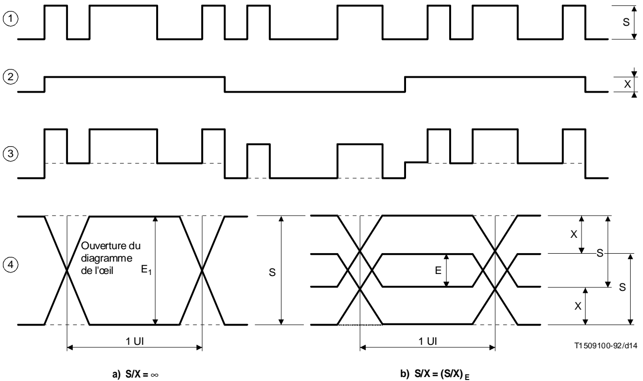
FIGURE II.4/G.957 Configuration de mesure de S/X
