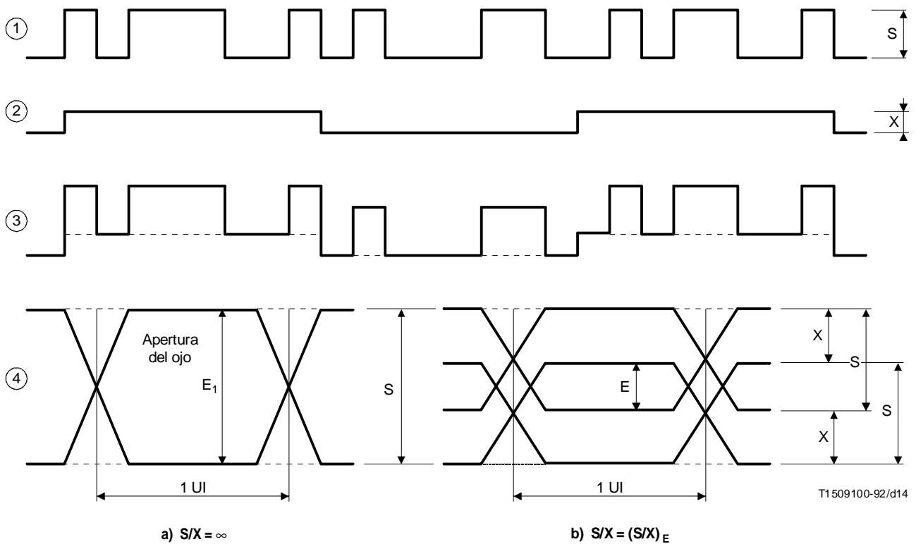
FIGURA II.4/G.957 Configuración para la medición de S/X
