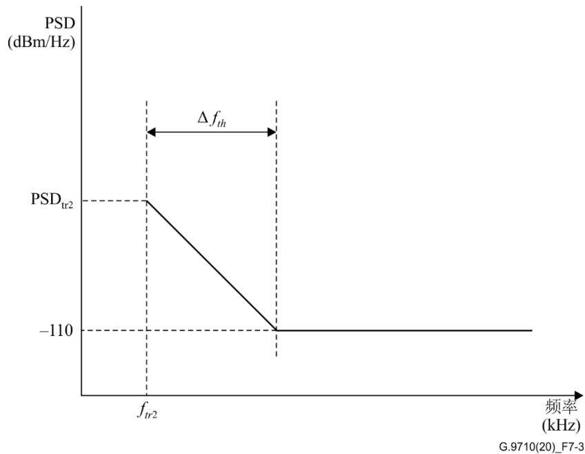
图7-3 – 高频端的带外LPM
