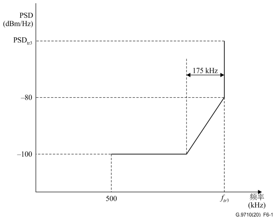
图6-1 – 低频端的阻带掩膜
