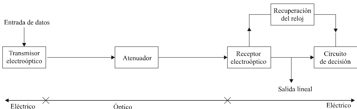
Figura 1/G.976 – Posible posición de la salida lineal para la prueba del equipo terminal
