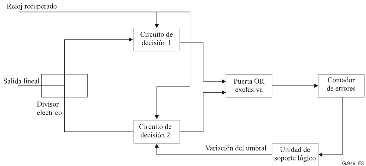
Figura 3/G.976 – Diagrama esquemático de una implementación de equipo de medición de la Q
