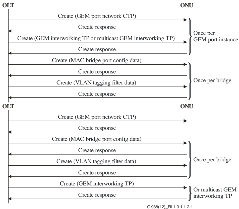
G.988(12)_Fil.1.3.1.1.2-1
