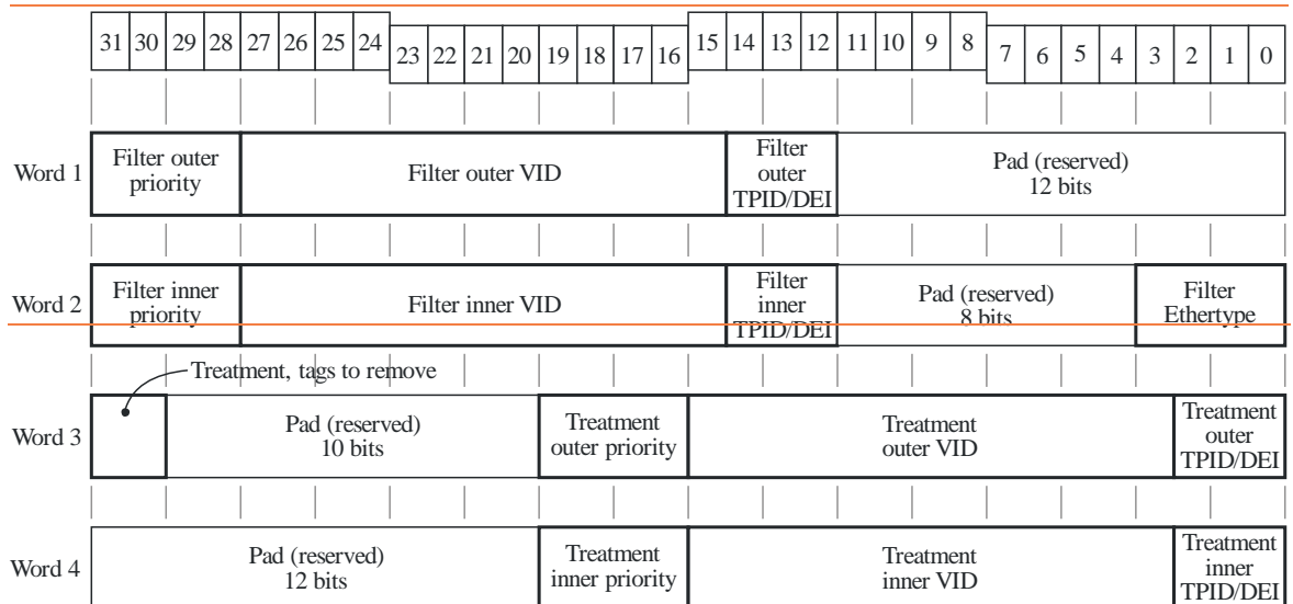
G.988(12)_F9.3.13-1
