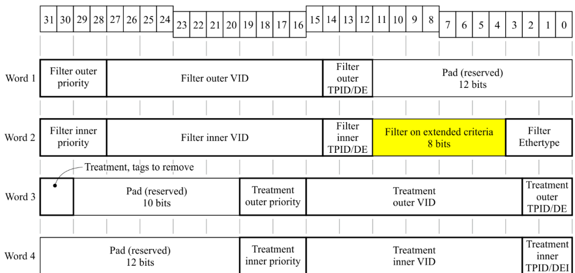
G.988(17)-Amd.1(18)_F9.3.13-1
