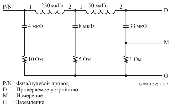
Рисунок С.1 – Эквивалент сети электропитания
