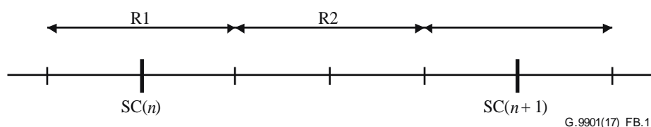
Рисунок В.1 – Режекция частоты
