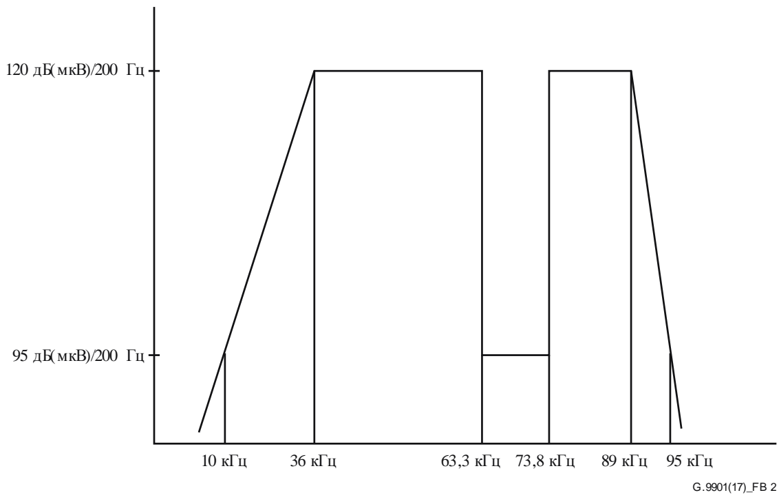
Рисунок В.2 – Спектр с двумя режекциями, произведенными для совместной работы с модемом системы связи по линии электропередачи с расширенной частотной манипуляции
