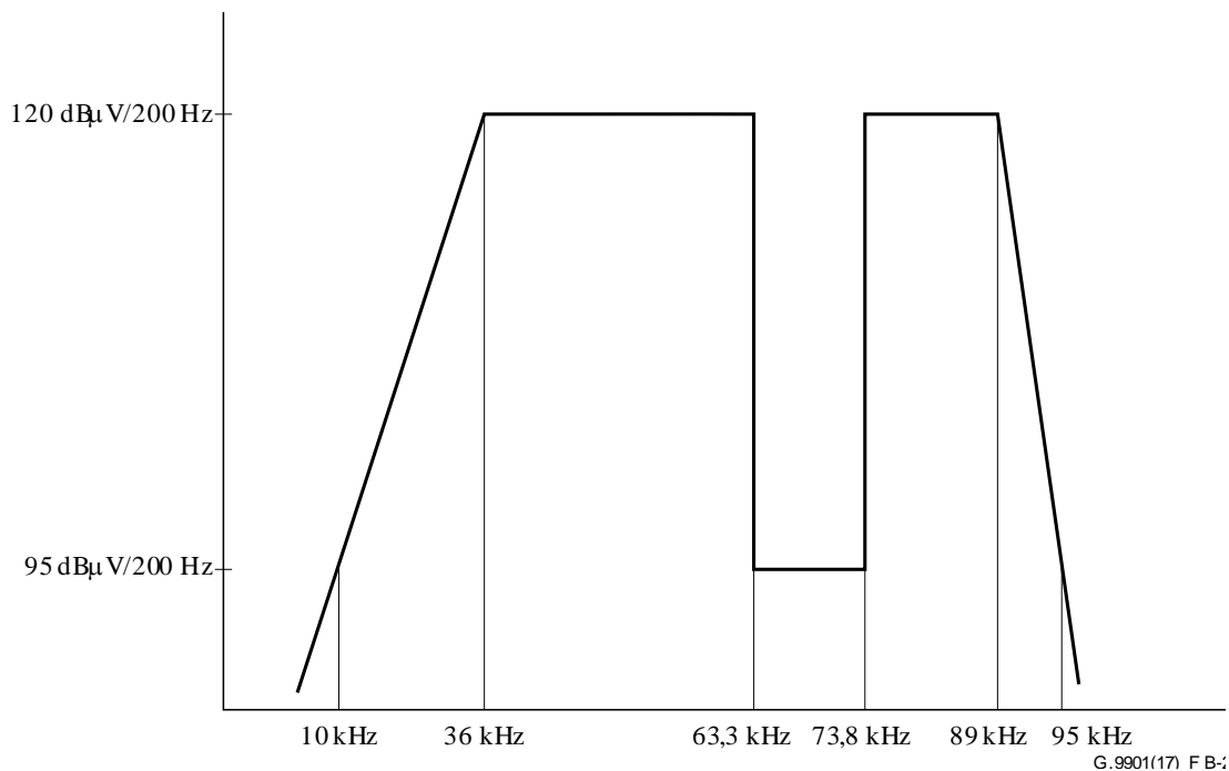
Figura B.2 – Espectro con dos filtros de banda eliminada insertados para cohabitar con el módem de comunicación por línea eléctrica con modulación por desplazamiento de fase ampliada
