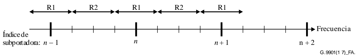
Figura A.1 – Aplicación de filtro de banda eliminada
