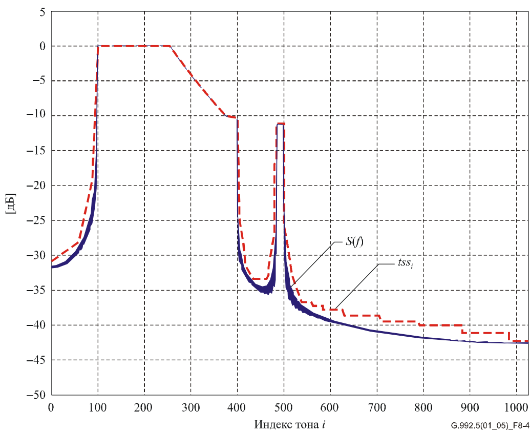
Рисунок 8-4/G.992.5 – Пример значений \log_{10} tss_i (в дБ) исходящего потока как функции от индекса поднесущей
