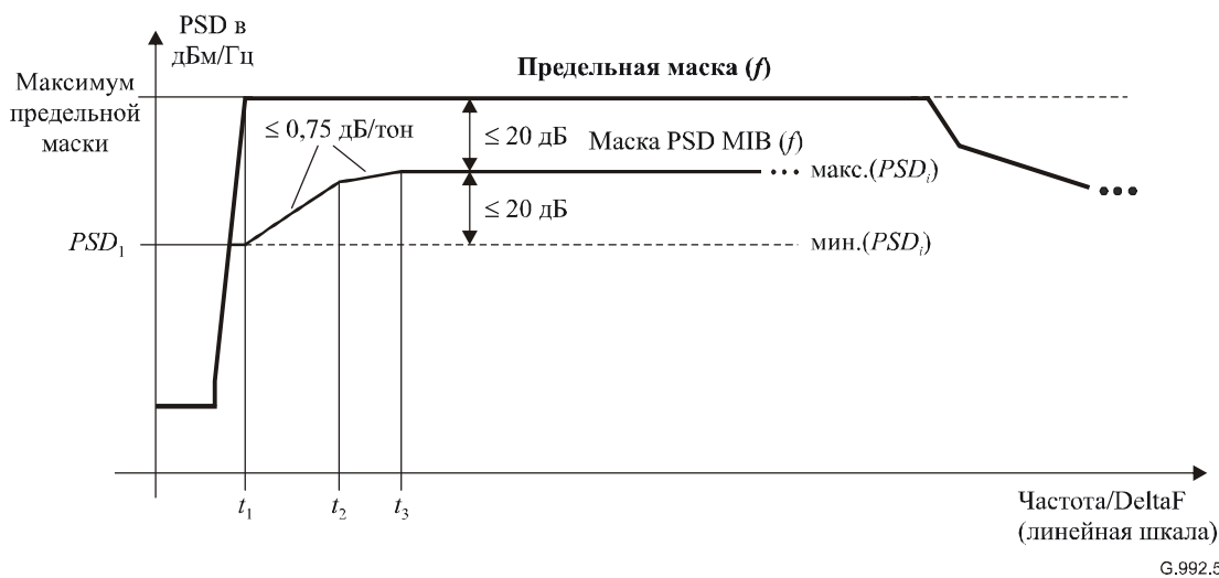
Рисунок 8.5.1-3/G.992.5 – Иллюстрация ограничений на внутриполосное формирование PSD MIB
