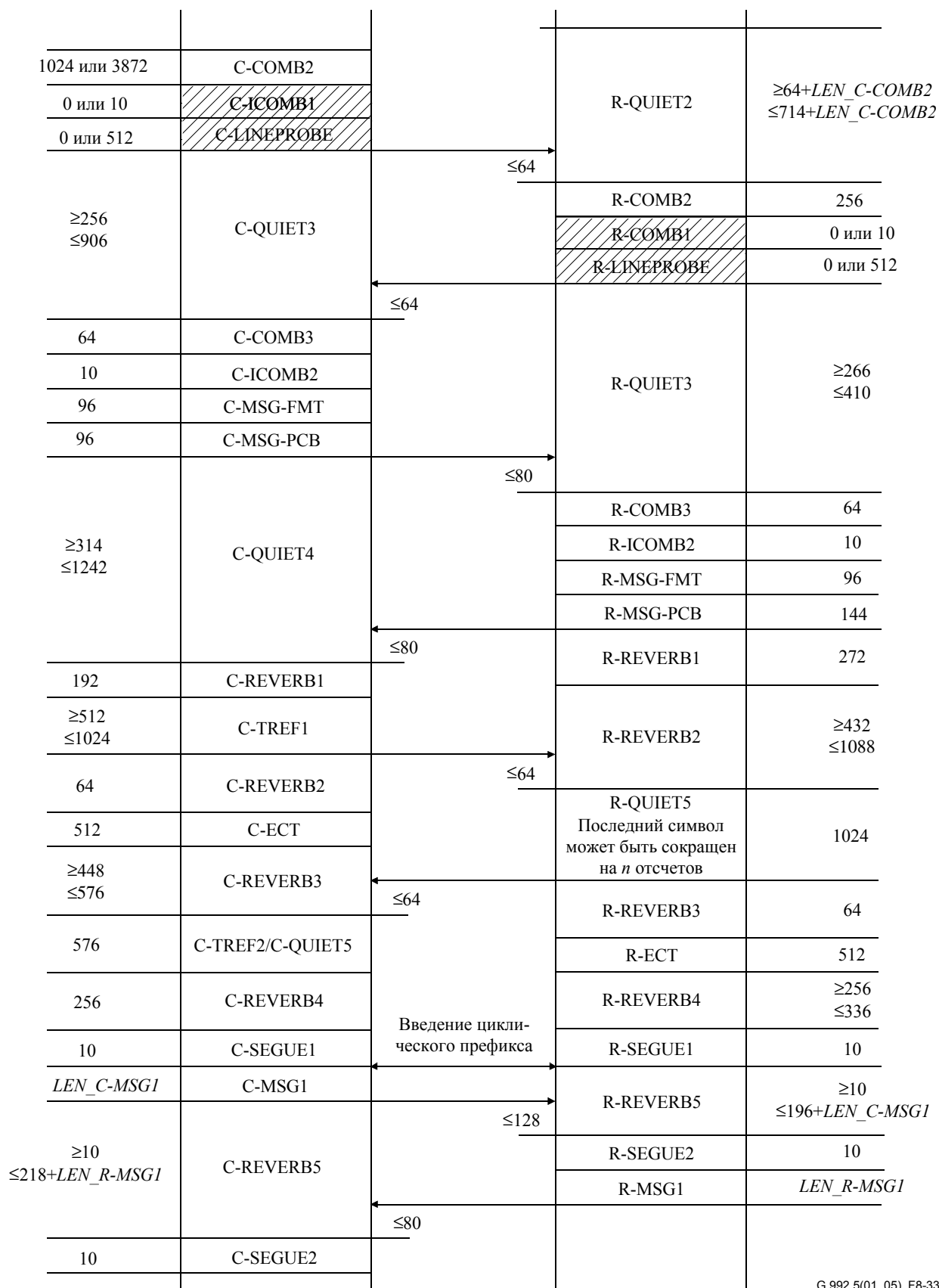
Рисунок 8-33/G.992.5 – Временная диаграмма короткой процедуры инициализации (часть 1)
