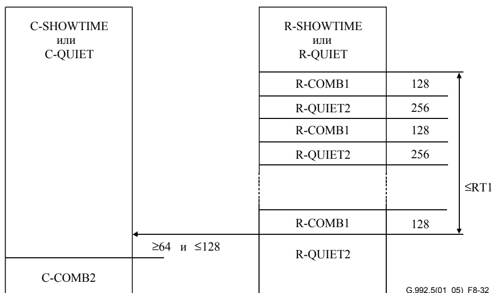
Рисунок 8-32/G.992.5 – Временная диаграмма вхождения в короткую процедуру инициализации, иницируемой ATU-R
