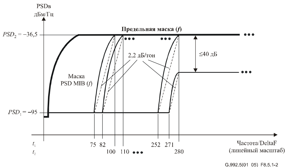
Рисунок 8.5.1-2/G.992.5 – Иллюстрация полосы непропуска в первой части полосы частот
