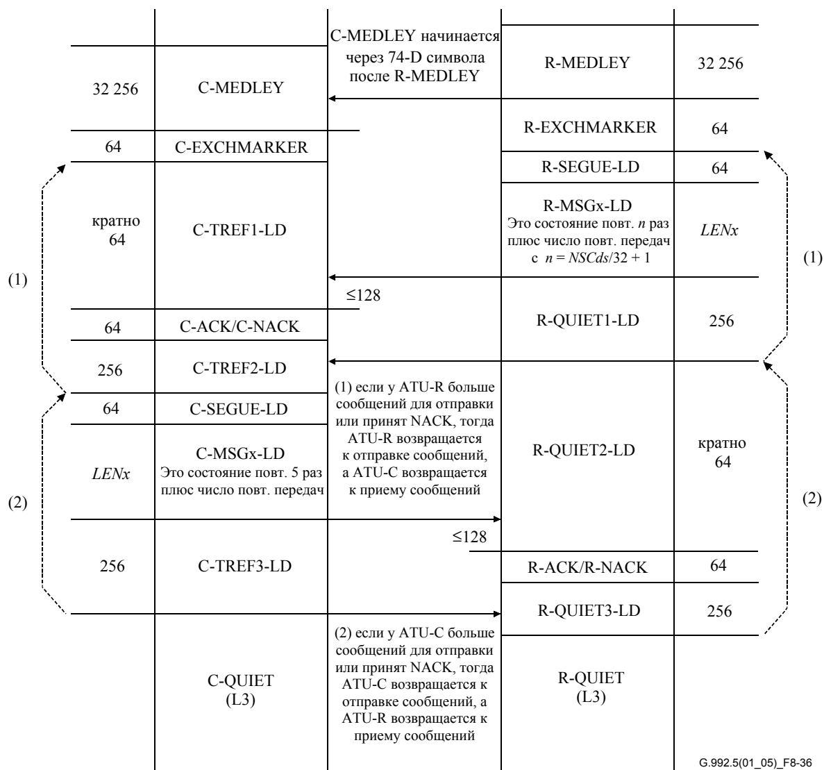
Рисунок 8-36/G.992.5 – Временная диаграмма диагностики шлейфа (часть 2)
