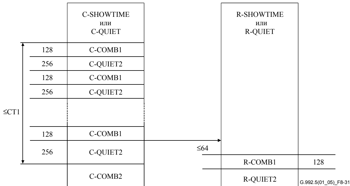
Рисунок 8-31/G.992.5 – Временная диаграмма вхождения в короткую процедуру инициализации, инициируемой ATU-C
