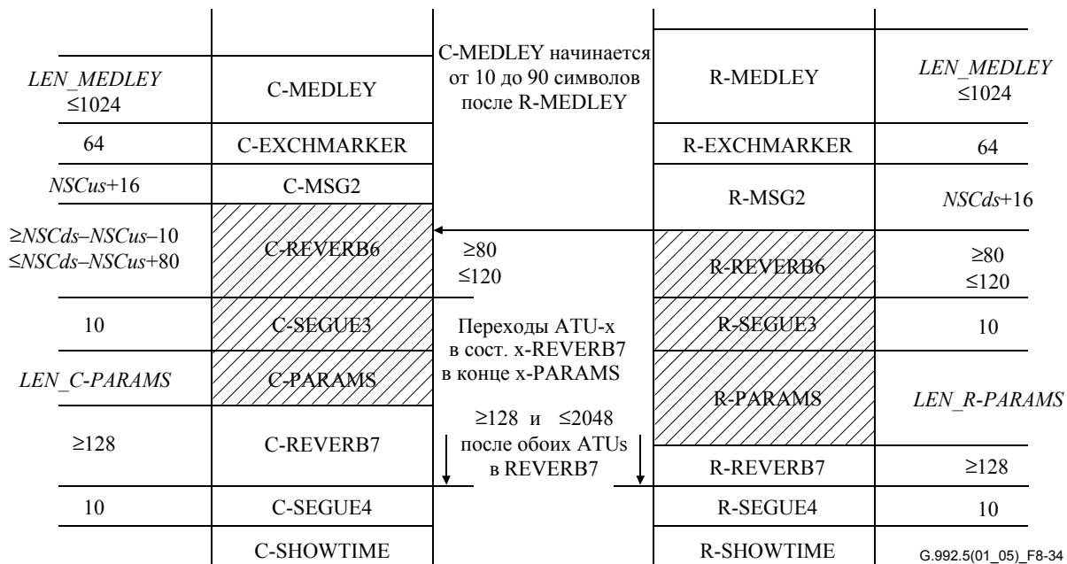
Рисунок 8-34/G.992.5 – Временная диаграмма короткой процедуры инициализации (часть 2)
