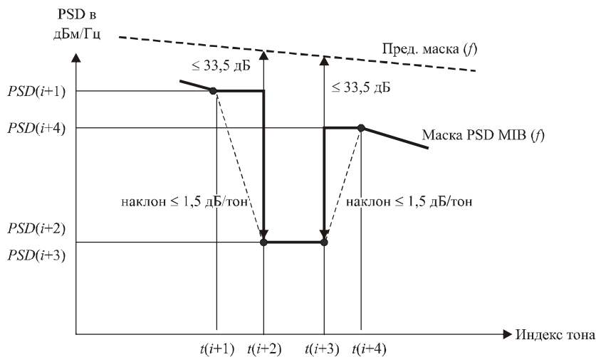
Рисунок 8.5.1-1/G.992.5 – Ограничения для точек излома и маски PSD MIB (f)
