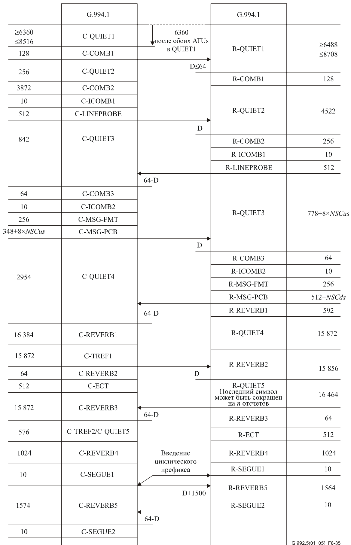
Рисунок 8-35/G.992.5 – Временная диаграмма диагностики шлейфа (часть 1)
