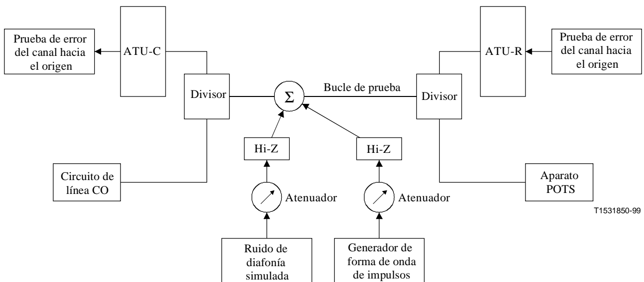
Figura 2/G.996.1 – Montaje de prueba en laboratorio para medir los márgenes de calidad de funcionamiento para el canal hacia el origen con divisores
