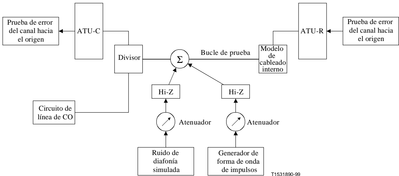
Figura 6/G.996.1 – Montaje de prueba de laboratorio para medir los márgenes de calidad de funcionamiento para el canal hacia el origen sin un divisor en la ATU-R
