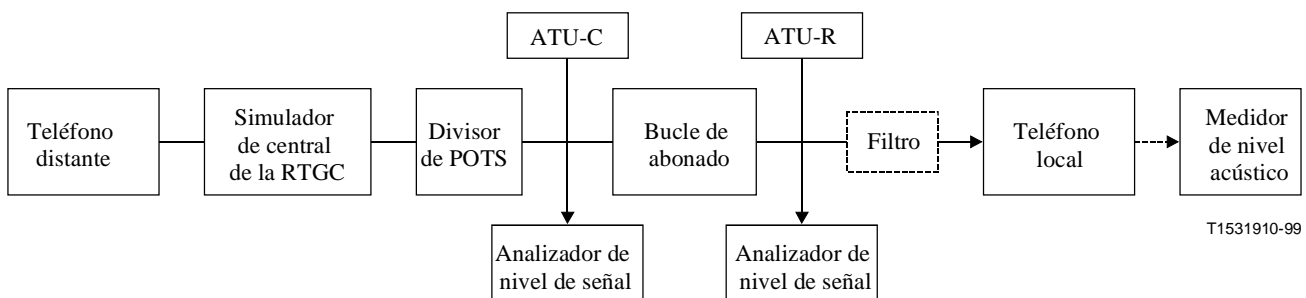
Figura 8/G.996.1 – Configuración de prueba
