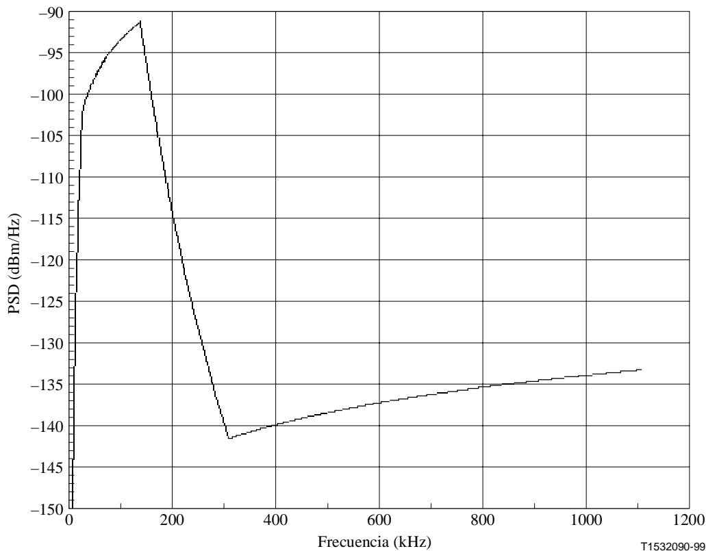
Figura 26/G.996.1 – PSD teórica de NEXT de señales G.992.2 hacia el origen con 49 perturbadores en el sentido hacia el destino
