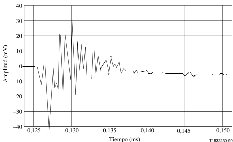
Figura 40/G.996.1 – Impulso de prueba 2
