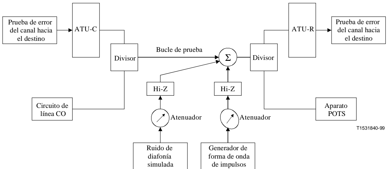
Figura 1/G.996.1 – Montaje de prueba en laboratorio para medir los márgenes de calidad de funcionamiento para el canal hacia el destino con divisores
