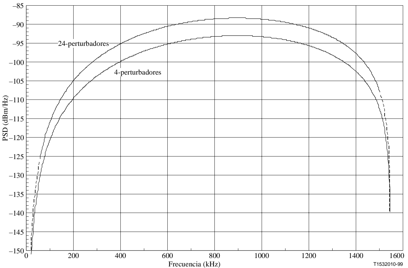
Figura 18/G.996.1 – NEXT de T1 de 4 y 24 perturbadores
