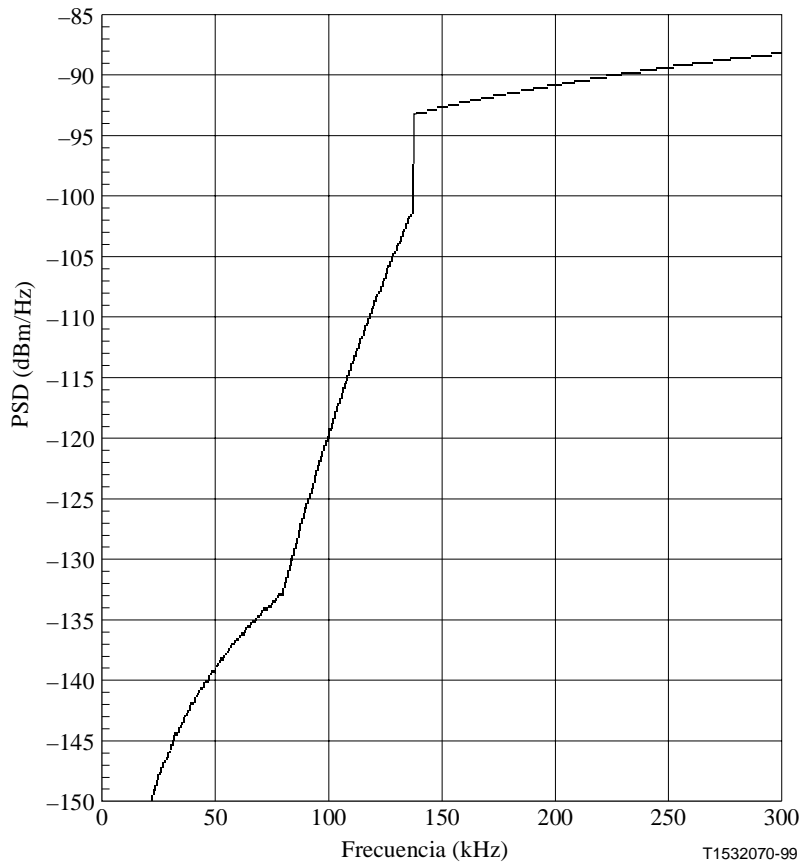
Figura 24/G.996.1 – NEXT de señales G.992.2 hacia el destino con 49 perturbadores en el sentido hacia el origen
