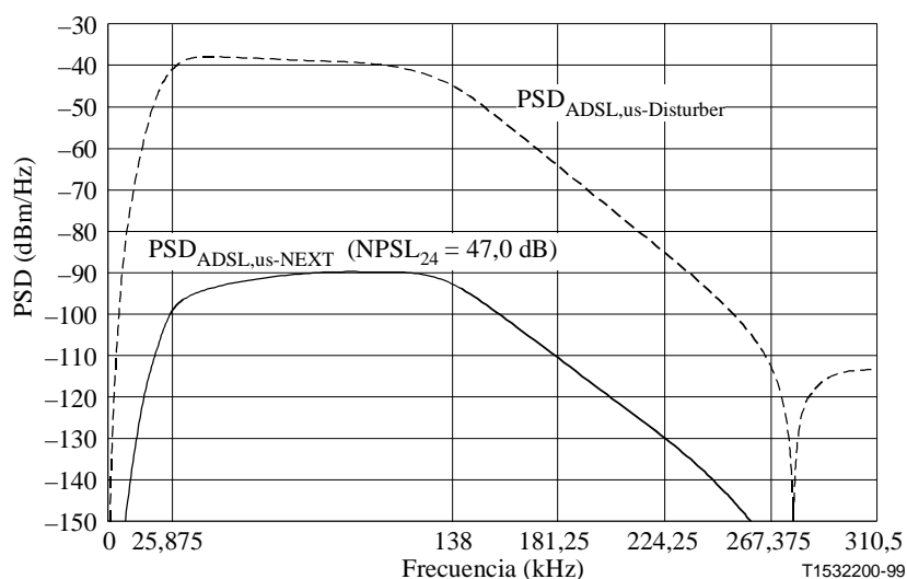
Figura 37/G.996.1 – NEXT hacia el origen de señales G.992.1/G.992.2 de 24 perturbadores
