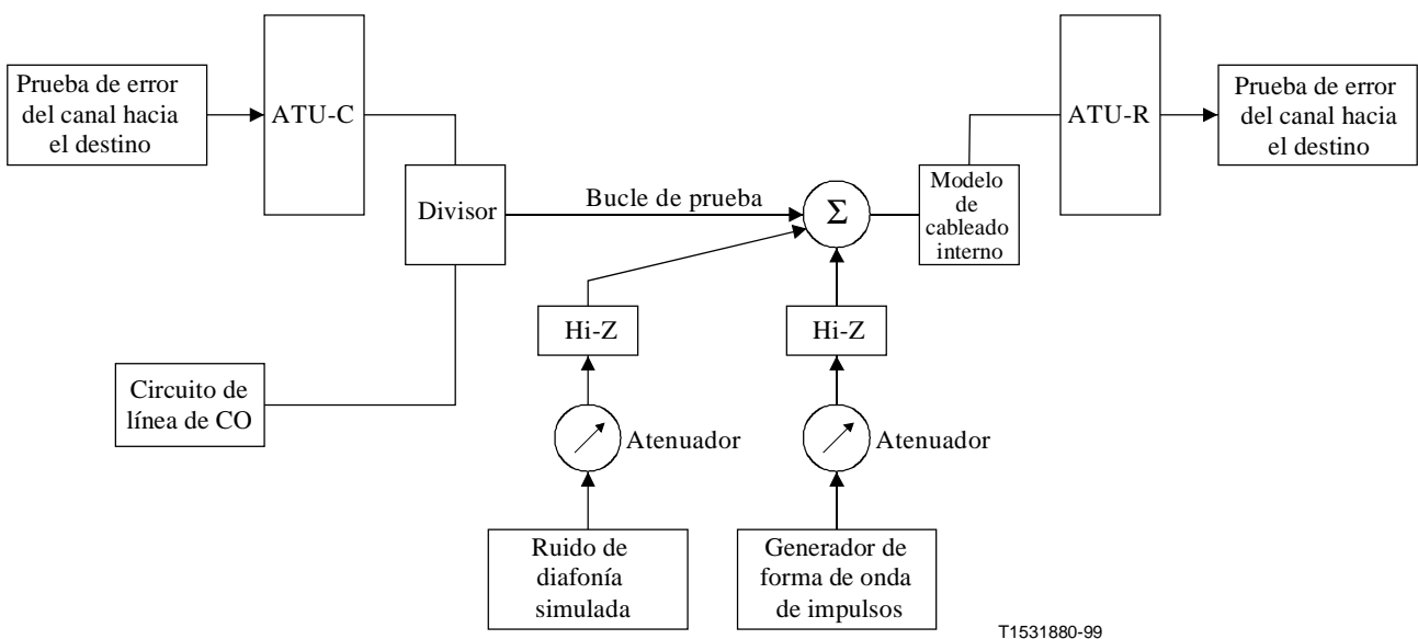
Figura 5/G.996.1 – Montaje de prueba de laboratorio para medir los márgenes de calidad de funcionamiento para el canal hacia el destino sin un divisor en la ATU-R
