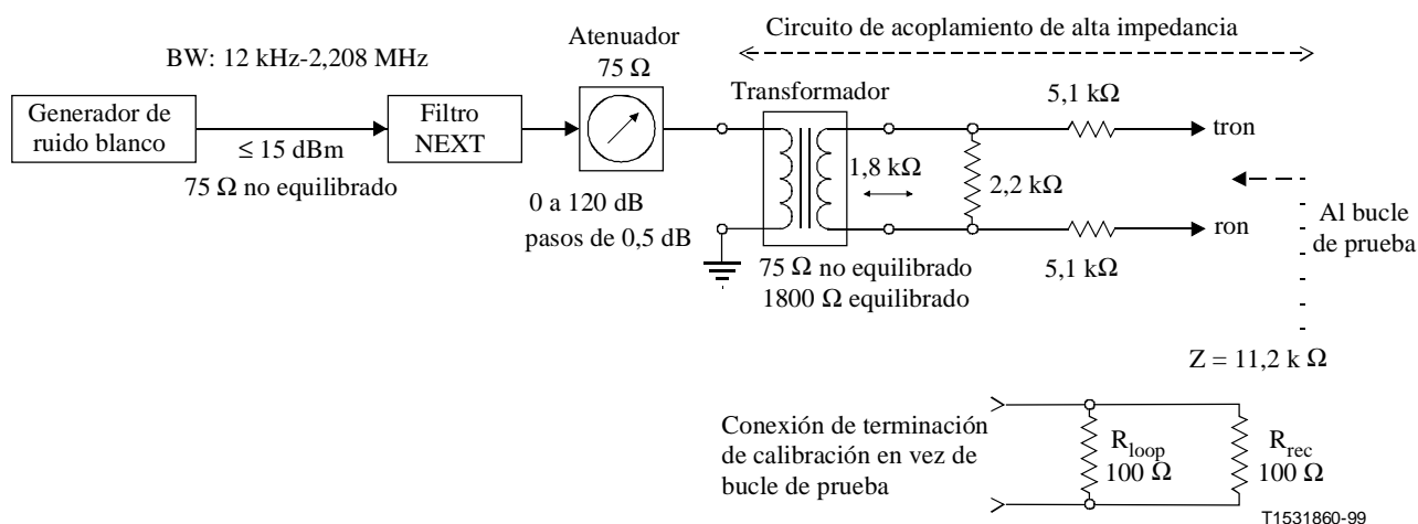
Figura 3/G.996.1 – Circuito de inyección de diafonía de alta impedancia
