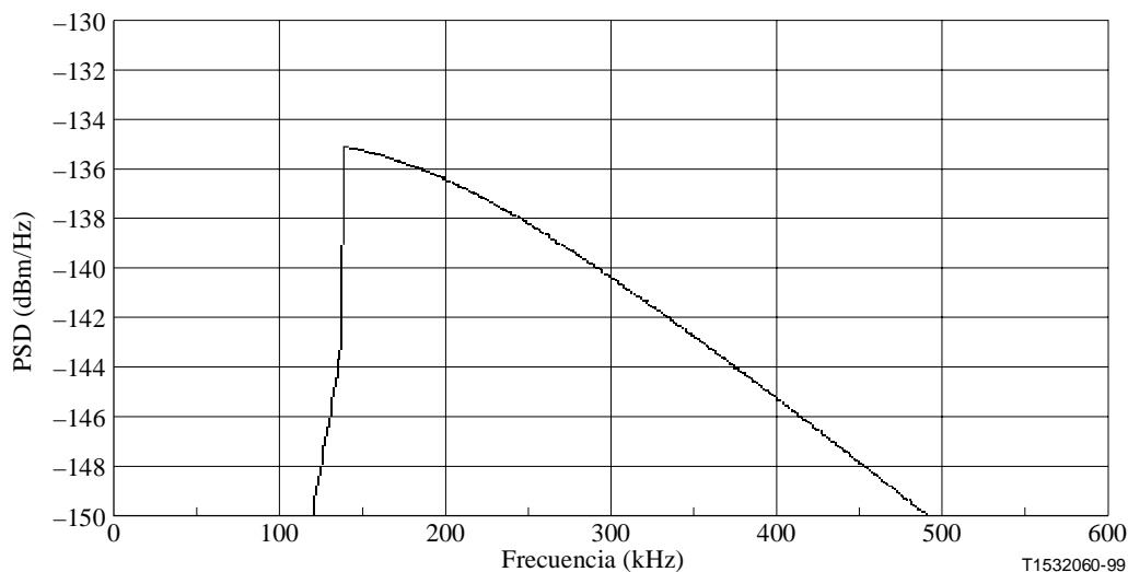
Figura 23/G.996.1 – FEXT de señales G.992.2 hacia el destino con 49 perturbadores en el bucle T #7
