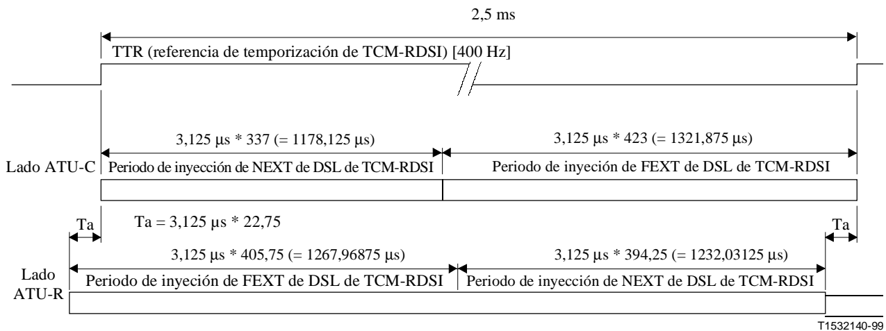
Figura 31/G.996.1 – Temporización de inyección de NEXT y FEXT alternas de DSL de TCM-RDSI
