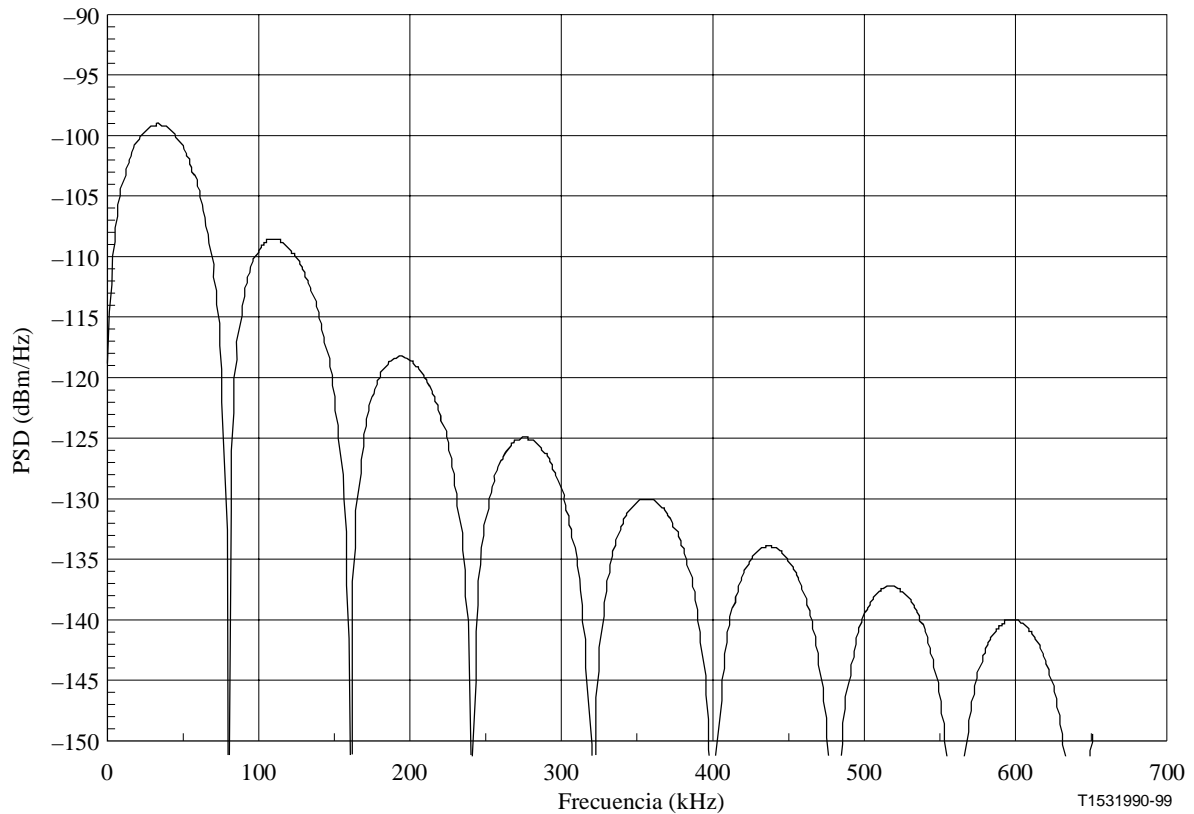
Figura 16/G.996.1 – NEXT de DSL de 24 perturbadores
