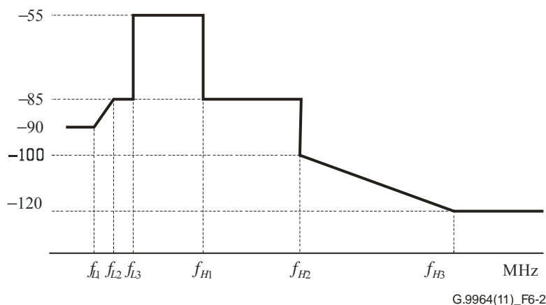
图6-2 – 25 MHz-PB、50 MHz-PB和100 MHz-PB 频段规划电力线基带传输的极限PSD掩膜（业余无线电频段陷波未列出）
