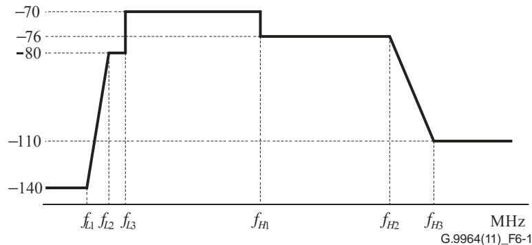
图 6-1 – 电话线传输的极限PSD掩膜 （业余无线电频段的陷波未显示）
