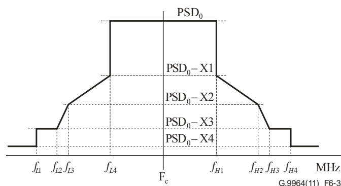
Figure 6-3 – Gabarit limite de densité PSD d'un canal unique pour l'émission à fréquence radioélectrique sur les câbles coaxiaux
