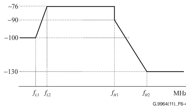
Figure 6-4 – Gabarit limite de densité PSD pour l'émission dans la bande de base sur un câble coaxial
