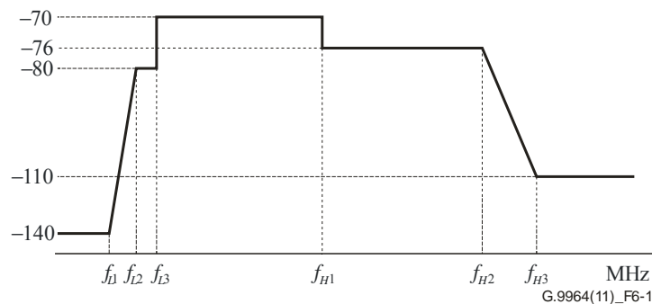
Figure 6-1 – Gabarit limite de densité PSD pour l'émission sur les lignes téléphoniques (les bandes radioamateur éliminées ne sont pas représentées)
