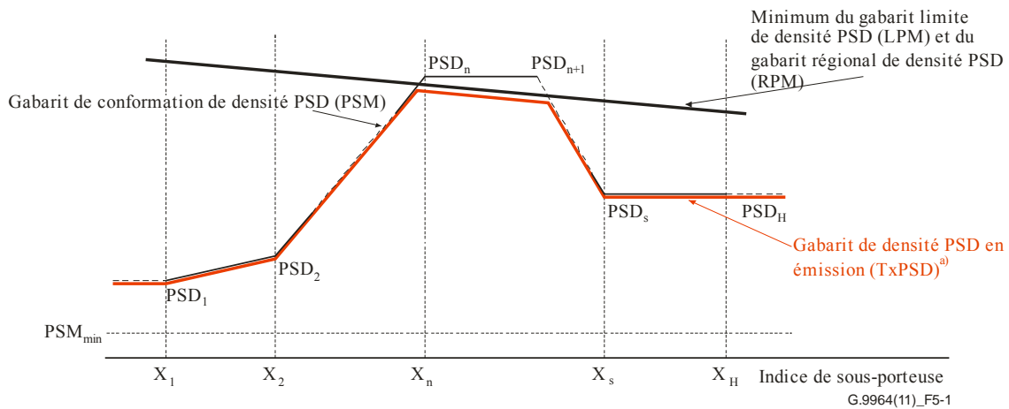
Figure 5-1 – Structure du gabarit de densité PSD en émission
