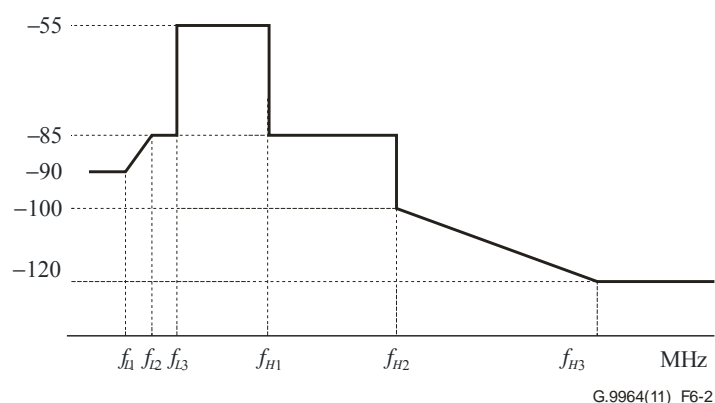
Figure 6-2 – Gabarit limite de densité PSD pour l'émission sur les lignes électriques pour les plans de bande 25 MHz-PB, 50 MHz-PB et 100 MHz-PB (les bandes radioamateur éliminées ne sont pas représentées)
