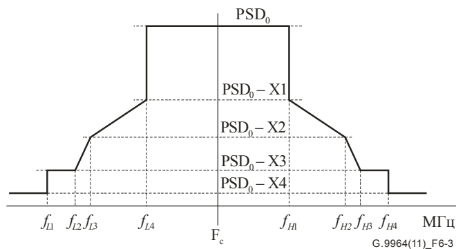
Рисунок 6-3 – Маска ограничения PSD одного канала для передачи РЧ-сигналов по коаксиальному кабелю
