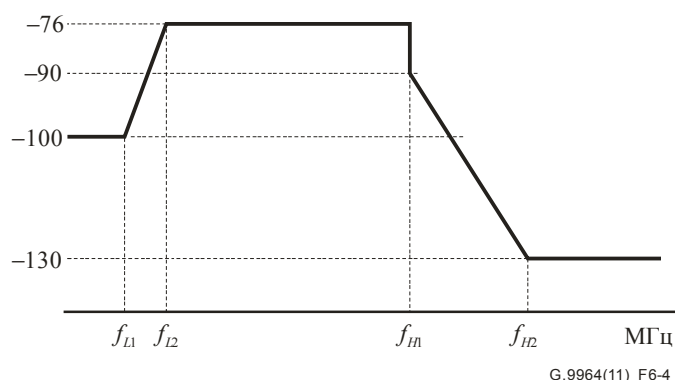
Рисунок 6-4 – Маска ограничения PSD базового диапазона коаксиального кабеля
