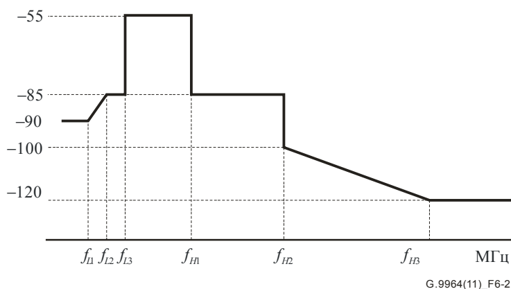
Рисунок 6-2 – Маска ограничения PSD для передачи сигналов по линиям электропитания для частотных планов 25 МГц-РВ, 50 МГц-РВ и 100 МГц-РВ (участки подавления диапазонов любительской радиосвязи не показаны)
