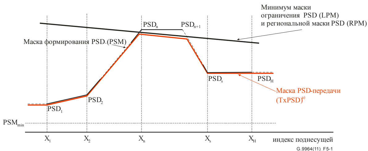
Рисунок 5-1 – Построение маски PSD-передачи
