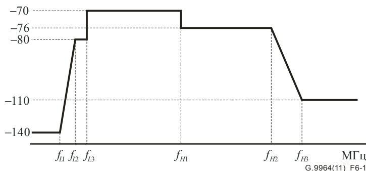
Рисунок 6-1 – Маска ограничения PSD для передачи сигналов по телефонным линиям (участки подавления диапазонов любительской радиосвязи не показаны)
