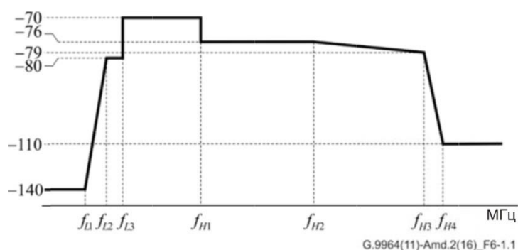
Рисунок 6-1.1 – Маска ограничения PSD для передачи сигналов по телефонным линиям (участки подавления диапазонов любительской радиосвязи не показаны)
