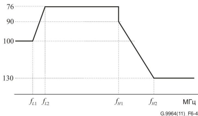
Рисунок 6-4 – Маска ограничения PSD базового диапазона коаксиального кабеля
