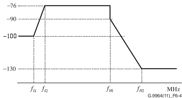
图 6-4 – 基带同轴电缆的极限PSD掩膜（配置1 OFB）
