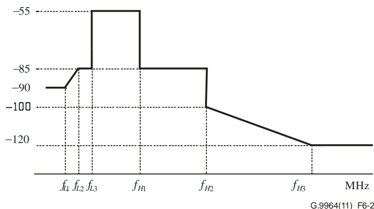
图6-2 – 25 MHz-PB、50 MHz-PB和100 MHz-PB 频段规划OFB电力线基带传输的极限PSD掩膜（业余无线电频段陷波未列出）
