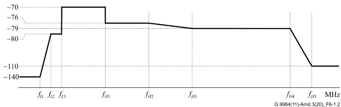
图 6-1.2 – 电话线传输的极限PSD掩膜 (业余无线电频段的陷波未显示)
