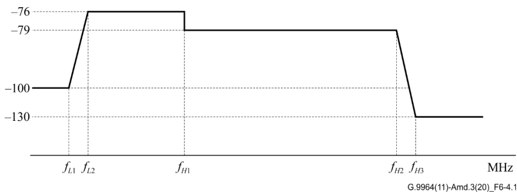
图 6-4.1 – 基带同轴电缆的极限PSD掩膜（配置2 OFB）
