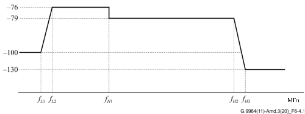
Рисунок 6-4.1 – Маска ограничения PSD коаксиального кабеля (OFB профиля 2)
