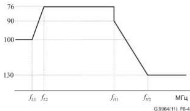
Рисунок 6-4 – Маска ограничения PSD базового диапазона коаксиального кабеля (OFB профиля 1)
