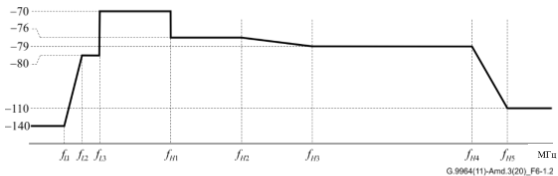
Рисунок 6-1.2 – Маска ограничения PSD для передачи сигналов по телефонным линиям (участки подавления диапазонов любительской радиосвязи не показаны)
