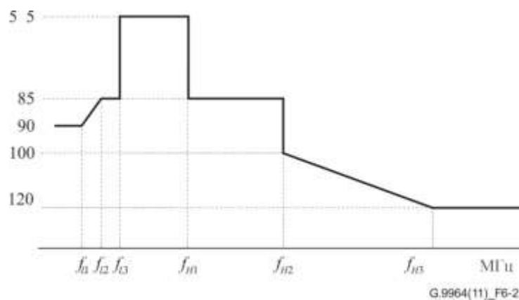
Рисунок 6-2 – Маска ограничения PSD для передачи сигналов по линиям электропитания для OFB частотных планов 25 МГц-РВ, 50 МГц-РВ и 100 МГц-РВ (участки подавления диапазонов любительской радиосвязи не показаны)
