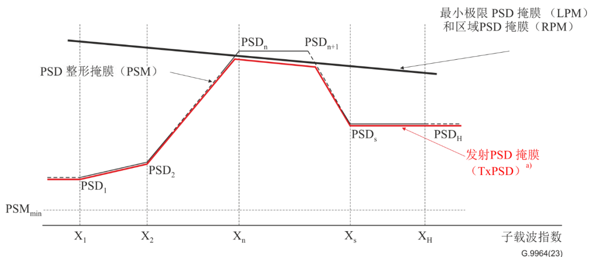
图5-1 – 建立发射PSD掩膜
