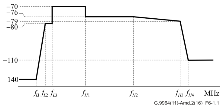
图6-1.1 – 电话线传输的LPM (业余无线电频段的陷波未显示)
