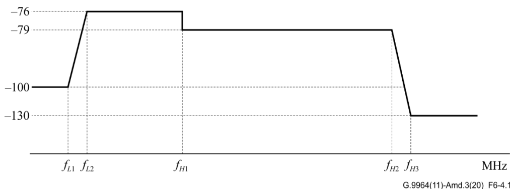
图6-4.1 – 基带同轴电缆的LPM（配置2 OFB）
