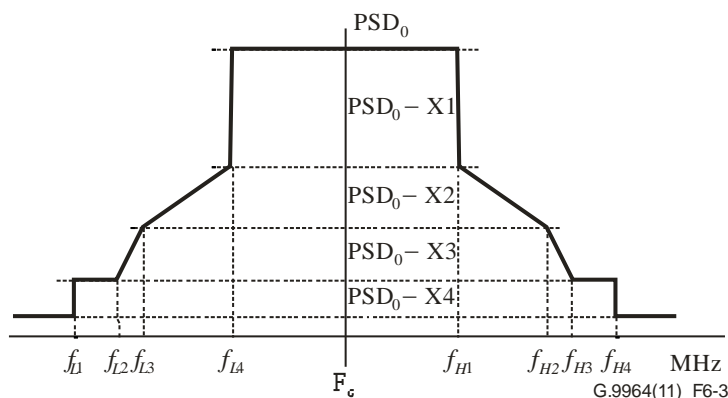
图6-3 – 单信道同轴电缆RF传输的LPM
