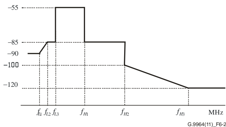
图6-2 – 25 MHz-PB、50 MHz-PB和100 MHz-PB OFB电力线基带传输的LPM（业余无线电频段陷波未列出）
