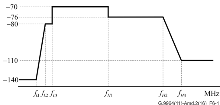
图6-1 – 电话线传输的LPM (业余无线电频段的陷波未显示)
