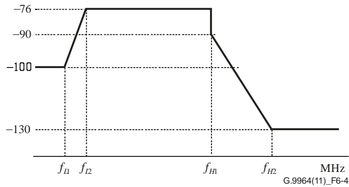
图6-4 – 基带同轴电缆的LPM（配置1 OFB）
