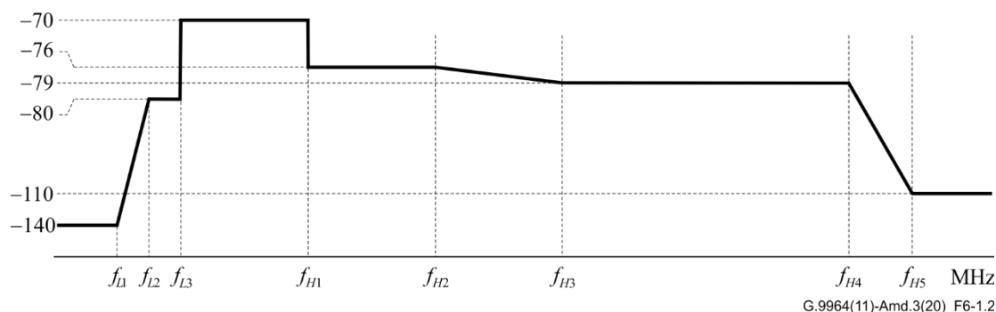
图6-1.2 – 电话线传输的LPM (业余无线电频段的陷波未显示)
