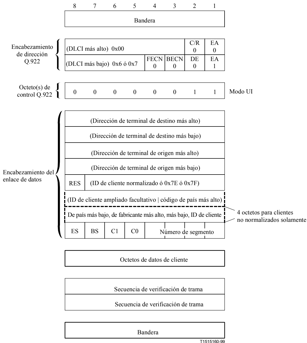
Figura 2/H.224 – Estructura de los octetos del protocolo H.224
