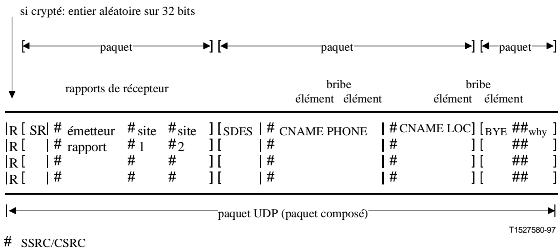
Figure A.1/H.225.0 – Exemple de paquet composé RTCP
