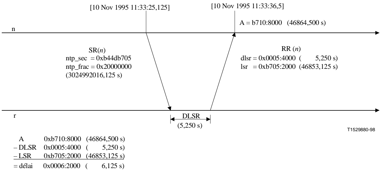
Figure A.2/H.225.0 – Exemple de calcul de temps de transmission aller-retour
