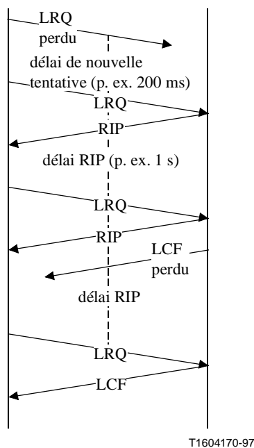
Figure 2/H.225.0 – Exemple d'utilisation du message RIP
