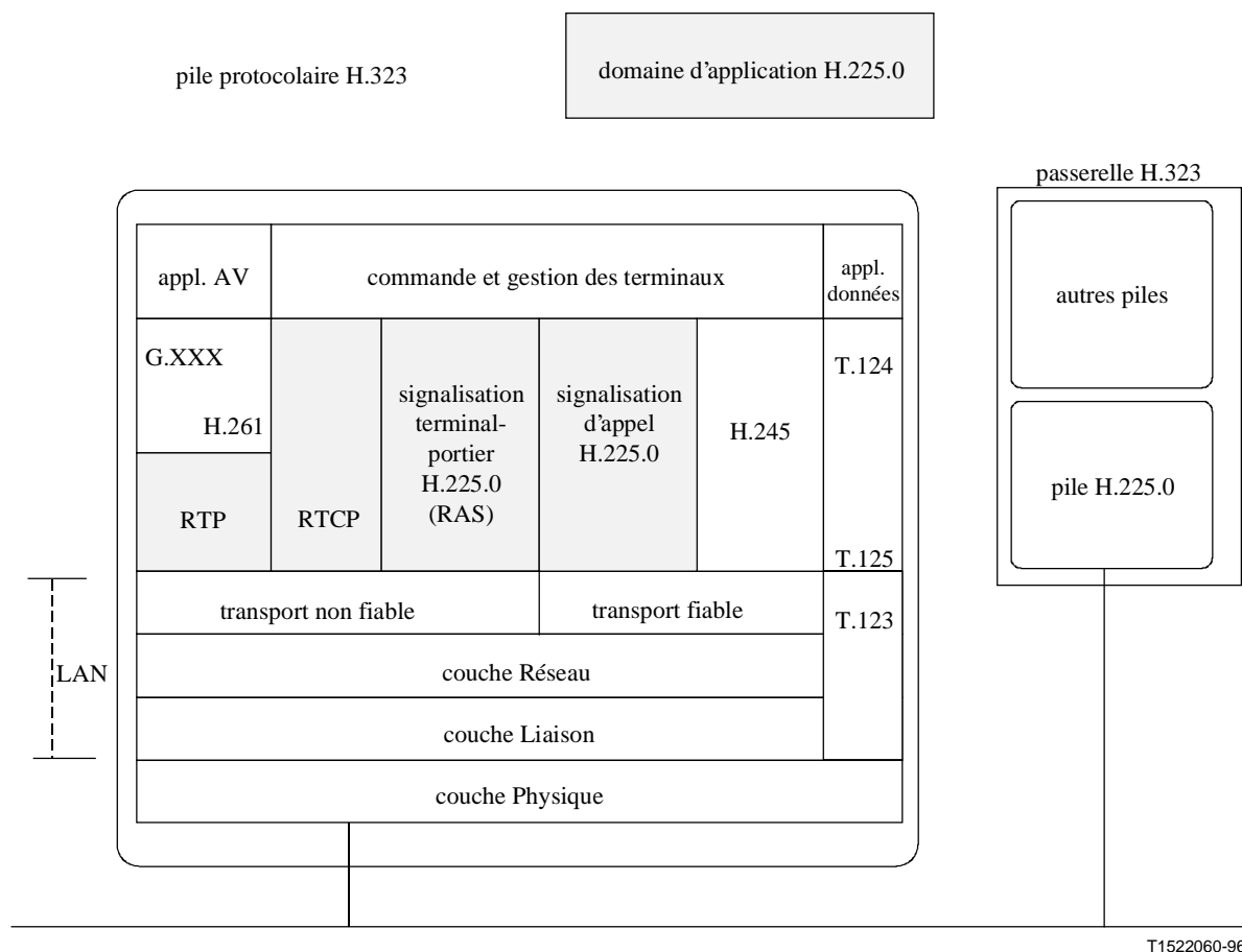
Figure 1/H.225.0 – Domaine d'application H.225.0
