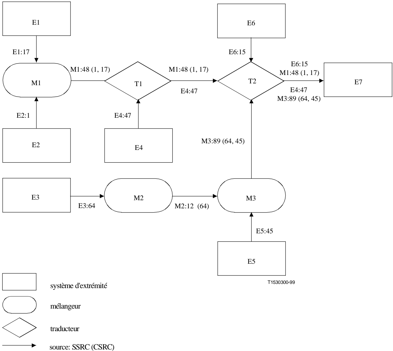
Figure A.3/H.225.0 – Exemple de réseau RTP avec des systèmes d'extrémité, des mélangeurs et des traducteurs
