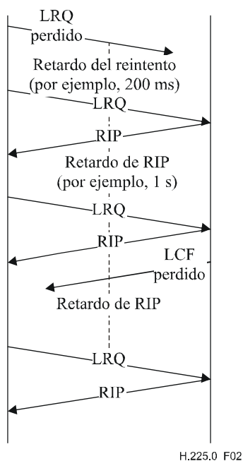
Figura 2/H.225.0 – Ejemplo de utilización del mensaje RIP
