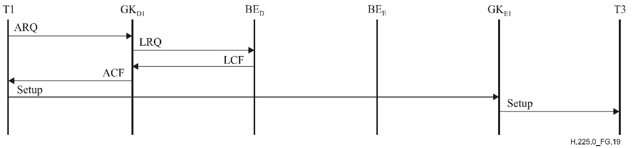
Figura G.19/H.225.0 – Ejemplo de llamada encaminada hacia el controlador de acceso utilizando descriptor caché
