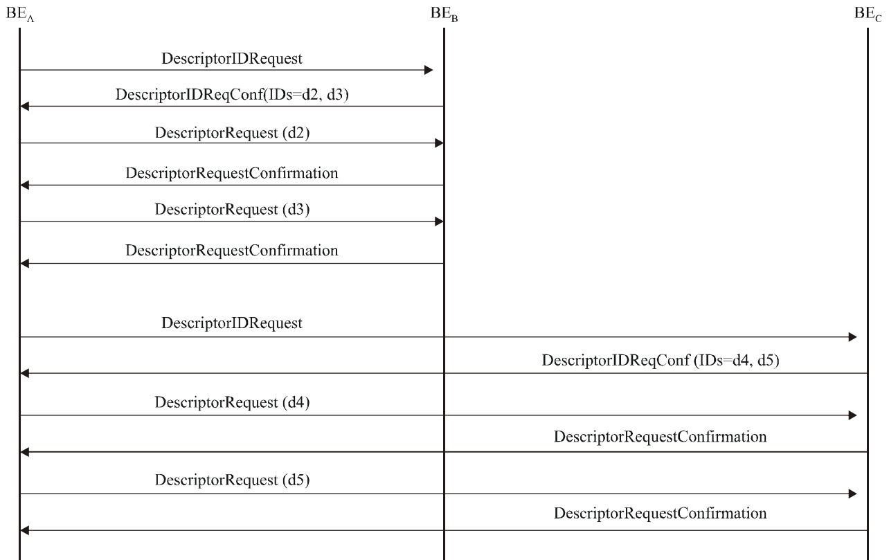
Figura G.8/H.225.0 – Ejemplo de intercambios de descriptores
