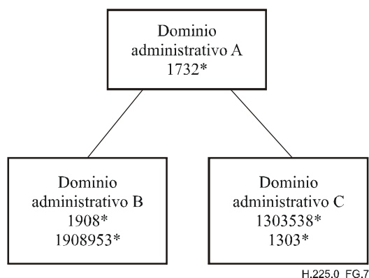
Figura G.7/H.225.0 – Ejemplos de red distribuida para señalización
