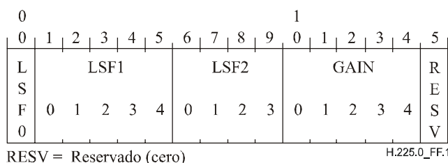
Figura F.1/H.225.0 – Formato de paquetización CNG de los anexos B/G.729, F/G.729 y G/G.729
