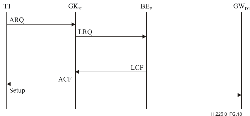
Figura G.18/H.225.0 – Ejemplo de llamada en que un elemento de frontera local utiliza un descriptor caché
