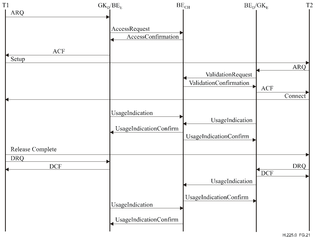
Figura G.21/H.225.0 – Ejemplo de validación e informe de utilización de llamada con centro de resolución
