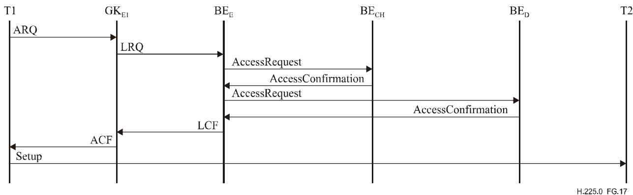
Figura G.17/H.225.0 – Ejemplo de encaminamiento con centro de resolución que utiliza información de contacto para responder al elemento de frontera distante
