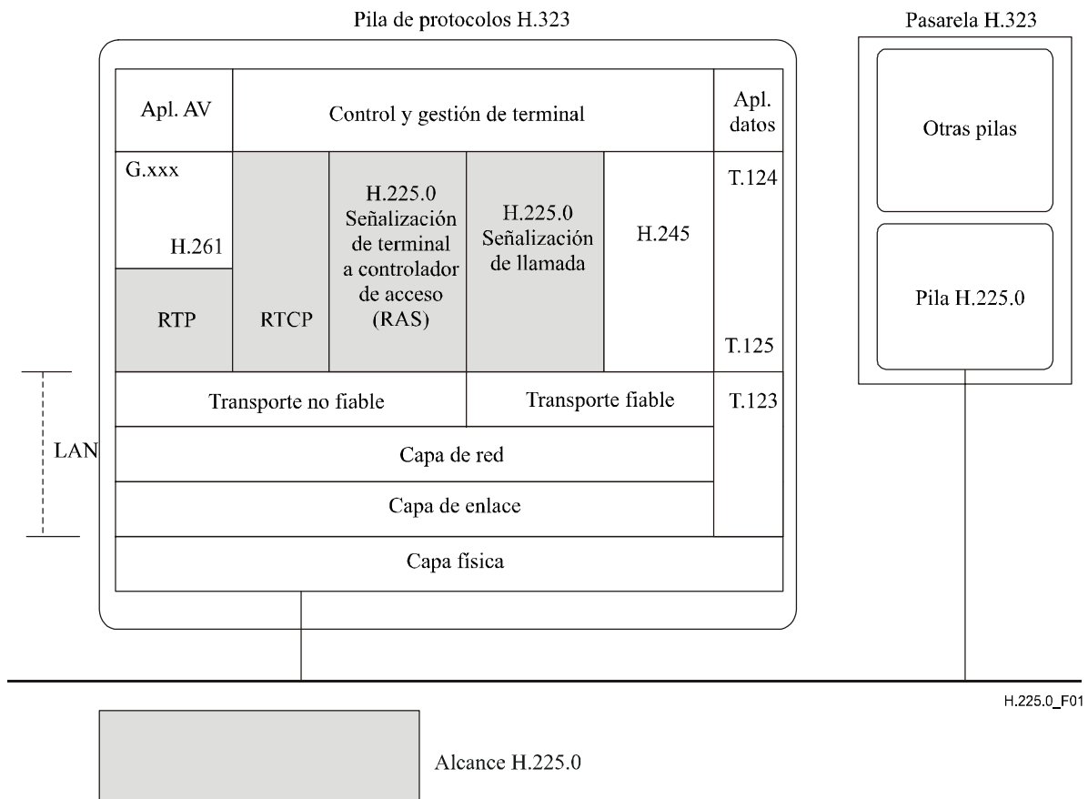
Figura 1/H.225.0 – Alcance H.225.0
