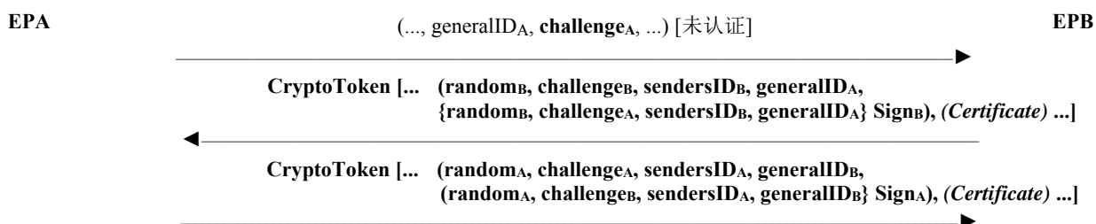
图 9 – 具有签名的基于证书认证，二次扫描
