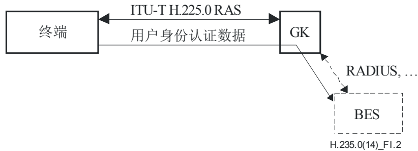
图I.2 – 后端业务方案
