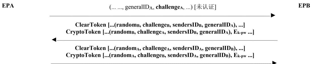
图 5 – 具有对称加密的口令，二次扫描
