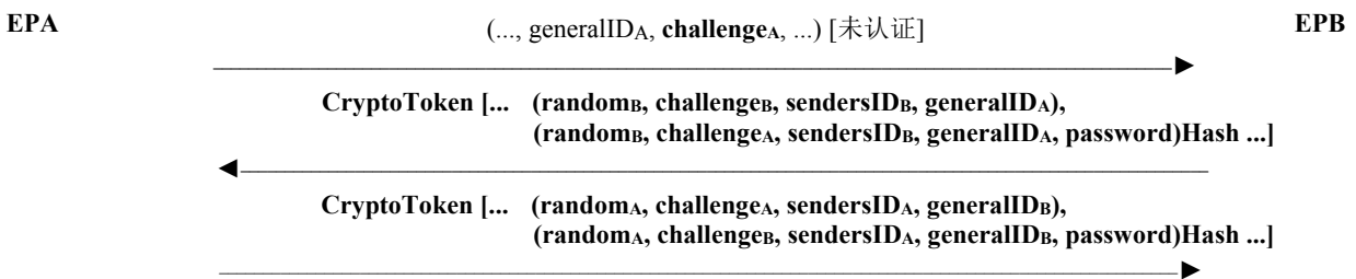
图 7 – 具有hash的口令，二次扫描
