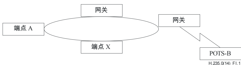
图 I.1 – Tokens
