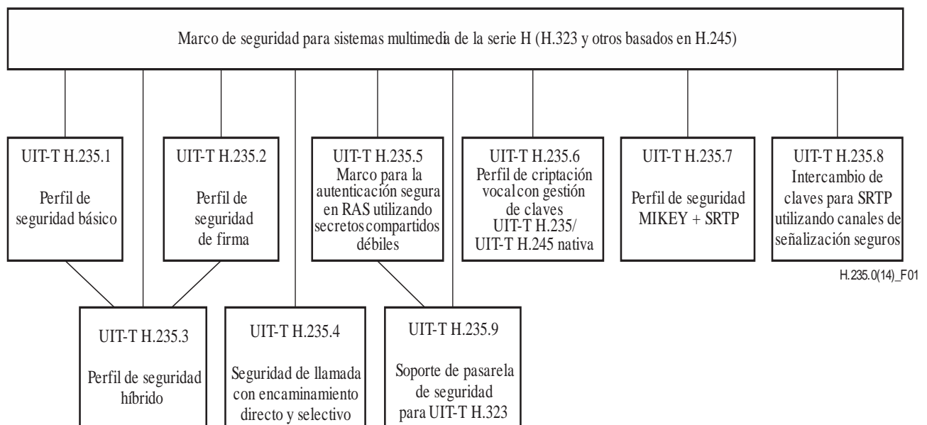
Figura 1 – Estructura de la subserie de Recomendaciones UIT-T H.235.x
