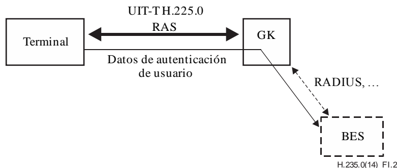
Figura I.2 – Escenario con servidor fuera del terminal
