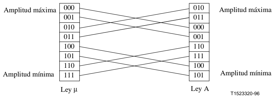
Figura X.1/H.242 – Orden de los segmentos de acuerdo con la amplitud, MIC ley \mu y ley A
