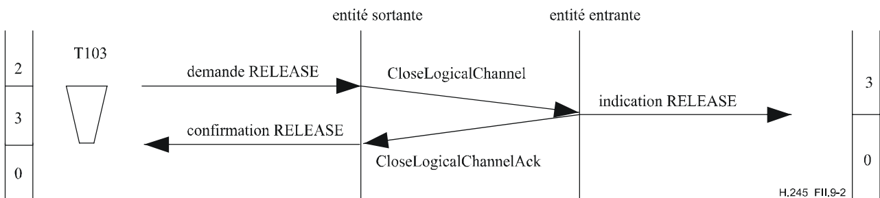
Figure II.9-2/H.245 – Libération de voie logique bidirectionnelle
