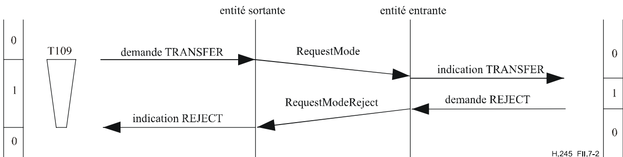
Figure II.7-2/H.245 – Demande de mode avec rejet provenant de l'utilisateur de l'entité MRSE homologue
