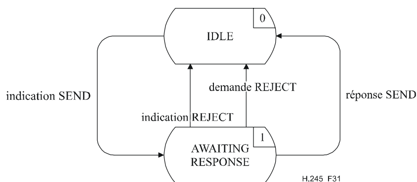
Figure C.31/H.245 – Diagramme de changement d'état pour la séquence de primitives dans l'entité RMESE entrante
