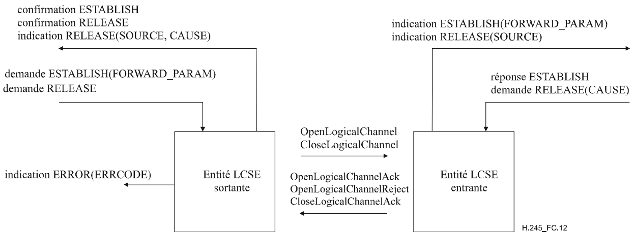
Figure C.12/H.245 – Primitives et messages de l'entité de signalisation de voie logique (LCSE)
