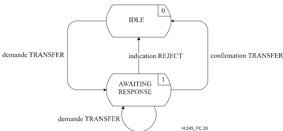
Figure C.35/H.245 – Diagramme de changement d'état pour la séquence de primitives de l'entité MRSE sortante
