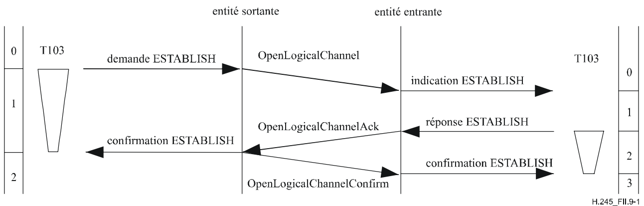
Figure II.9-1/H.245 – Etablissement de voie logique bidirectionnelle
