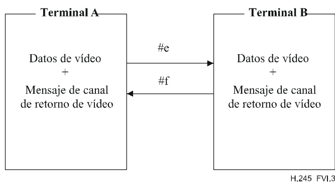
Figura VI.3/H.245 – Canales lógicos para modo multiplex de vídeo
