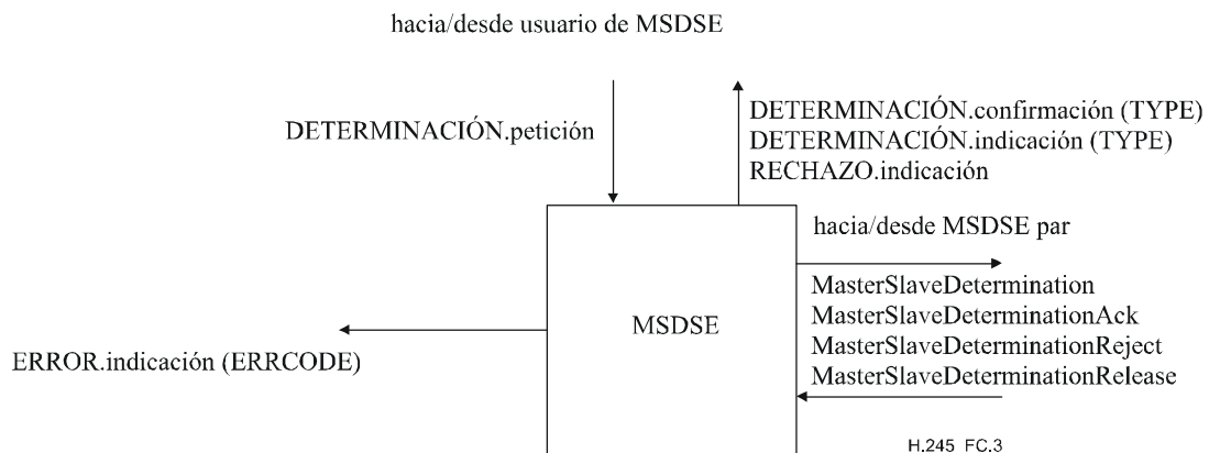
Figura C.3/H.245 – Primitivas y mensajes en la MSDSE
