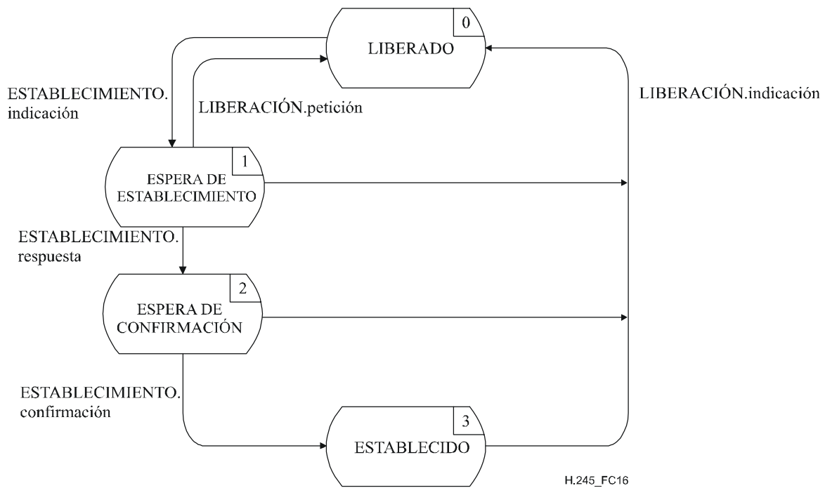
Figura C.16/H.245 – Diagrama de transición de estados para la secuencia de primitivas en una B-LCSE de entrada
