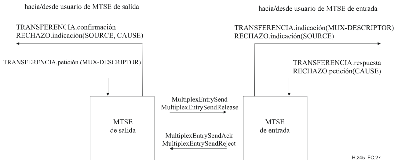
Figura C.27/H.245 – Primitivas y mensajes en la entidad de señalización de tabla múltiple
