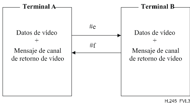
Figura VI.3/H.245 – Canales lógicos para modo múltiplex de vídeo
