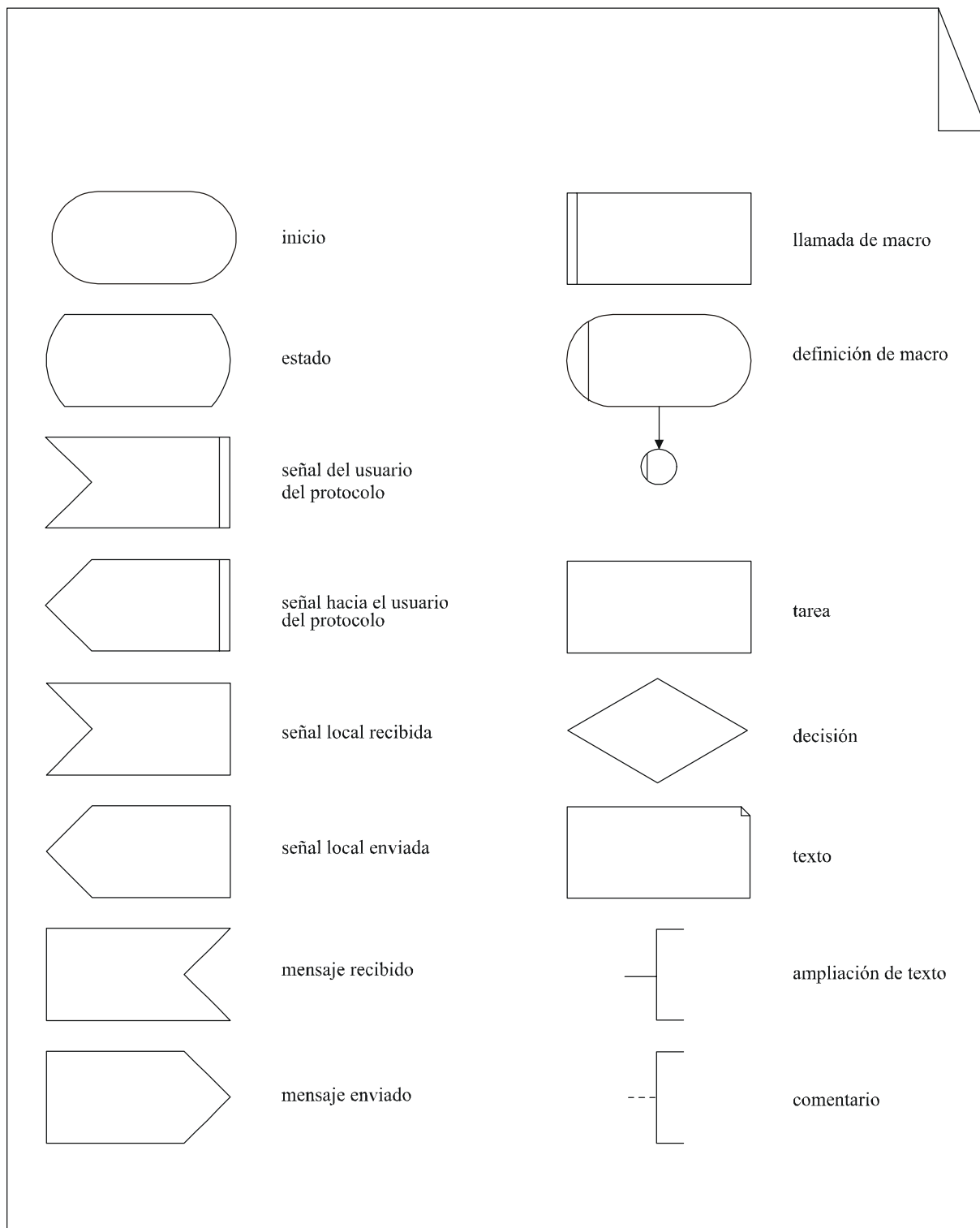
Figura C.1/H.245 – Símbolos gráficos utilizados en los diagramas SDL
