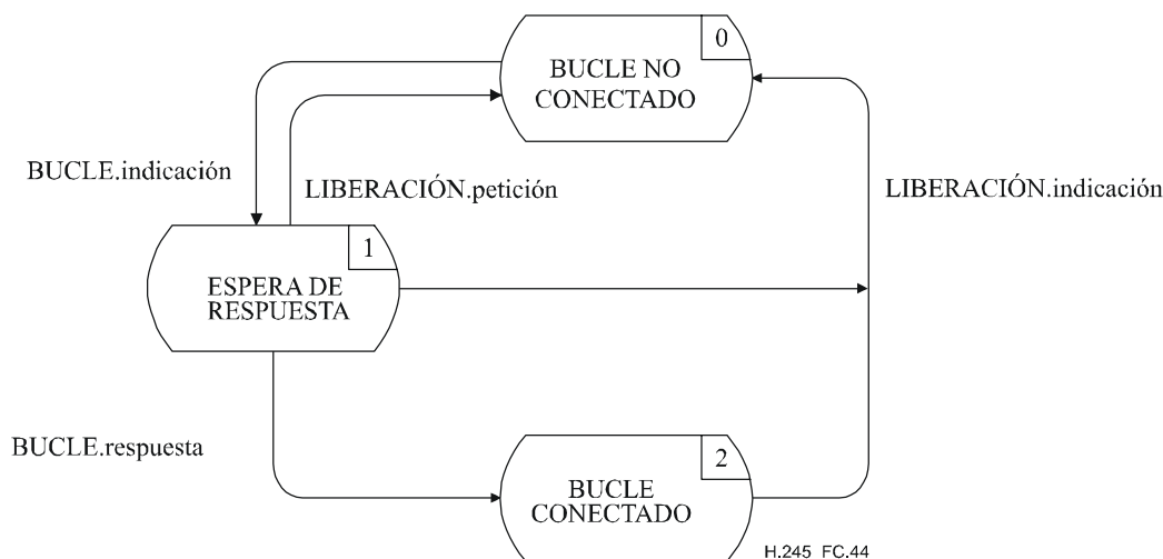
Figura C.44/H.245 – Diagrama de transición de estados para la secuencia de primitivas en la MLSE de entrada
