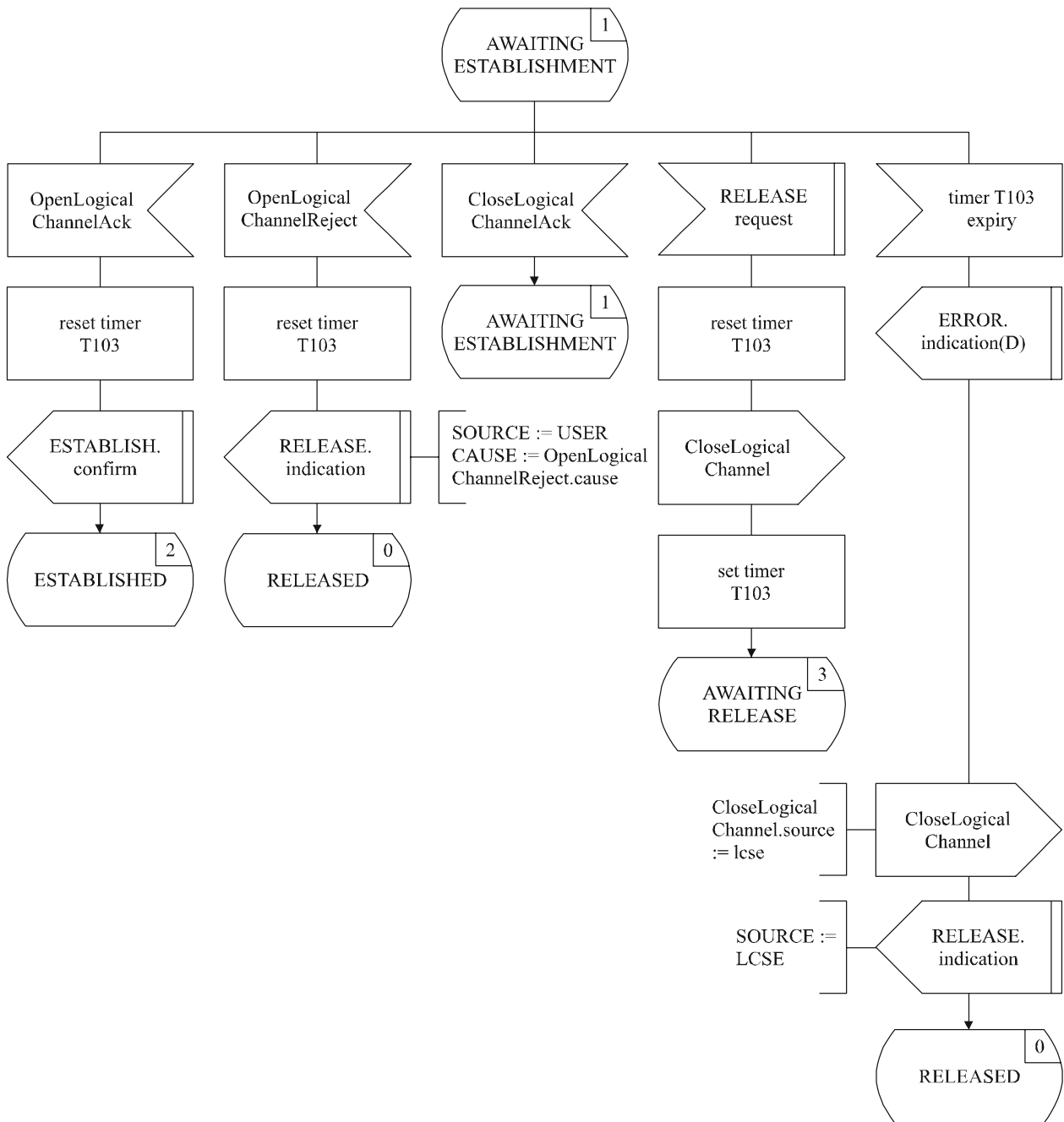
Figura C.13/H.245 – Diagrama SDL de la LCSE de salida (hoja 2 de 4)
