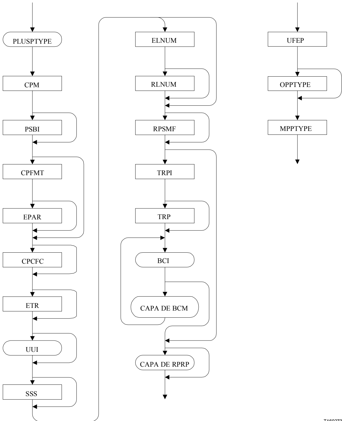
Figura 6/H.263 – Diagrama de sintaxis para el tren de bits de vídeo (parte 2 de 7)
