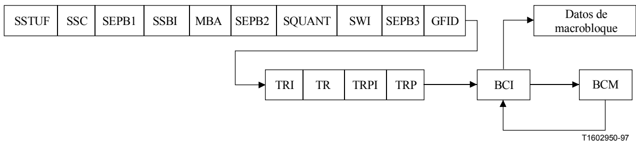
Figura N.3/H.263 – Estructura de la capa de rebanada para NEWPRED
