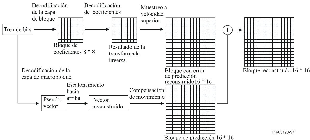
Figura Q.1/H.263 – Diagrama de bloques de la decodificación de bloques del modo actualización de resolución reducida
