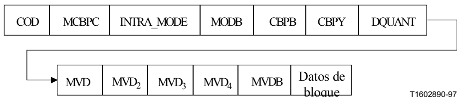
Figura I.1/H.263 – Estructura de la capa de macrobloque
