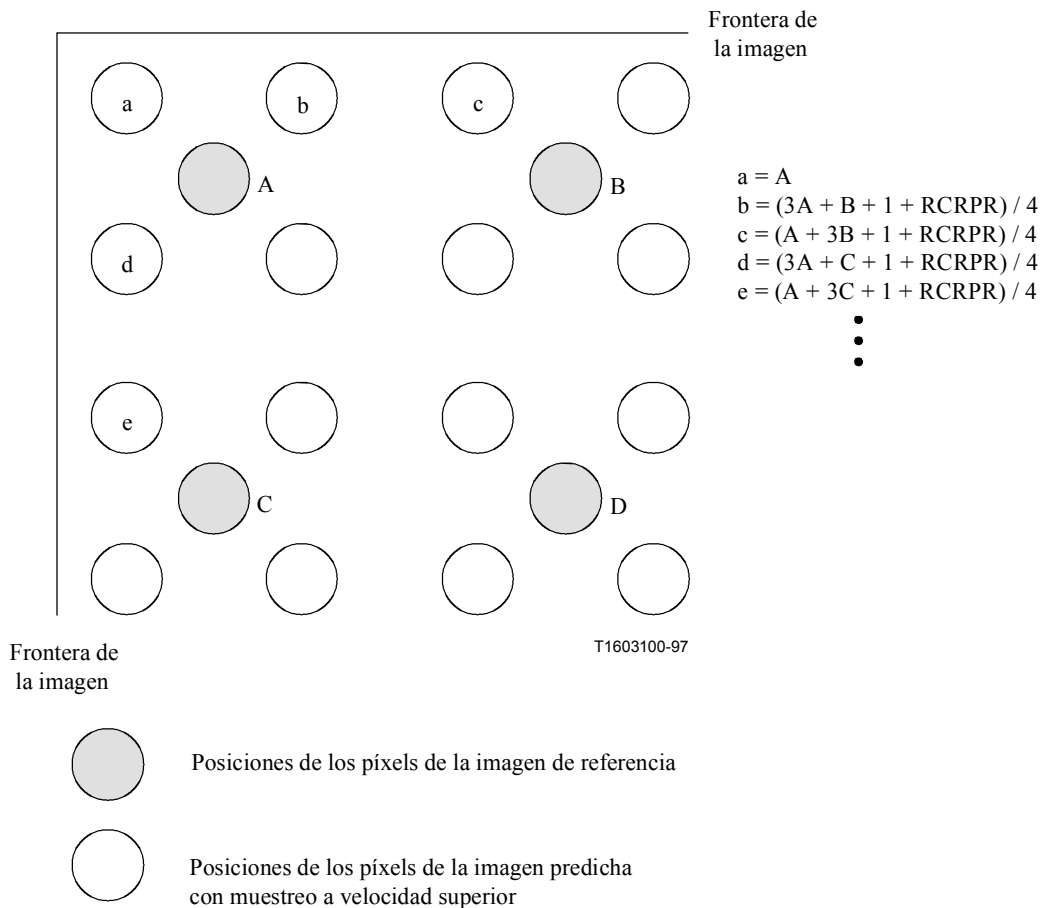
Figura P.5/H.263 – Muestreo a velocidad superior con factor de 4 para píxels en la frontera de la imagen (modo de recorte = recorte )
