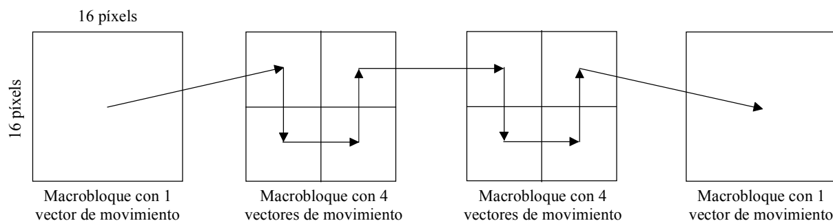
Figura V.2/H.263 – Predicción del vector de movimiento por camino único
