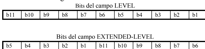
Figura T.1/H.263 – Rotación cíclica de la representación de coeficientes
