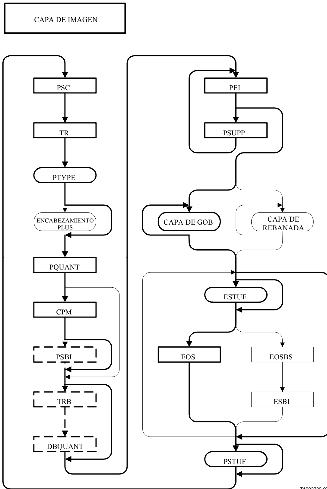
Figura 6/H.263 – Diagrama de sintaxis para el tren de bits de vídeo (parte 1 de 7)
