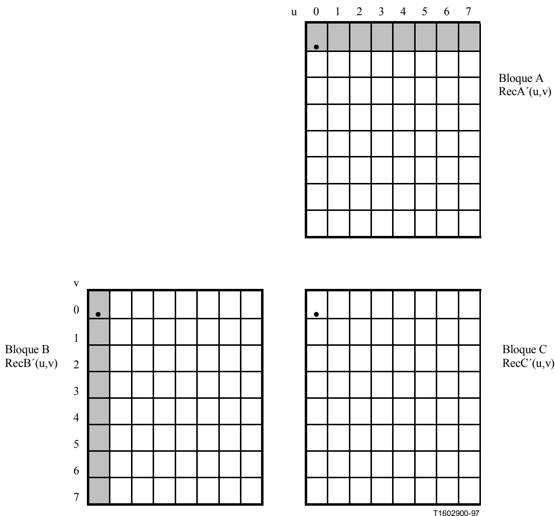
Figura I.3/H.263 – Tres bloques contiguos en el dominio DCT
