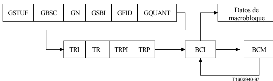
Figura N.2/H.263 – Estructura de la capa de GOB para NEWPRED
