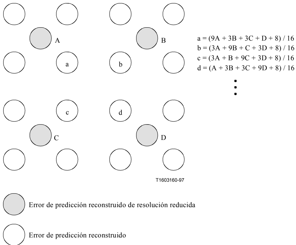
Figura Q.8/H.263 – Creación de error de predicción reconstruido para píxels situados dentro de un bloque
