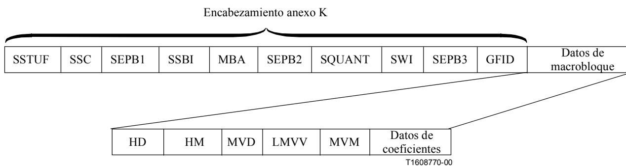
Figura V.1/H.263 – Sintaxis de la partición de datos
