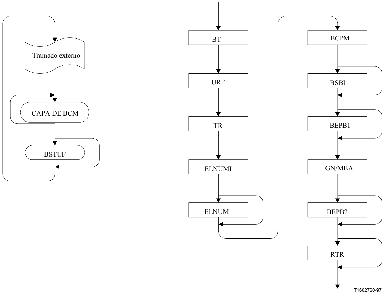
Figura 6/H.263 – Diagrama de sintaxis para el tren de bits de vídeo (parte 5 de 7)
