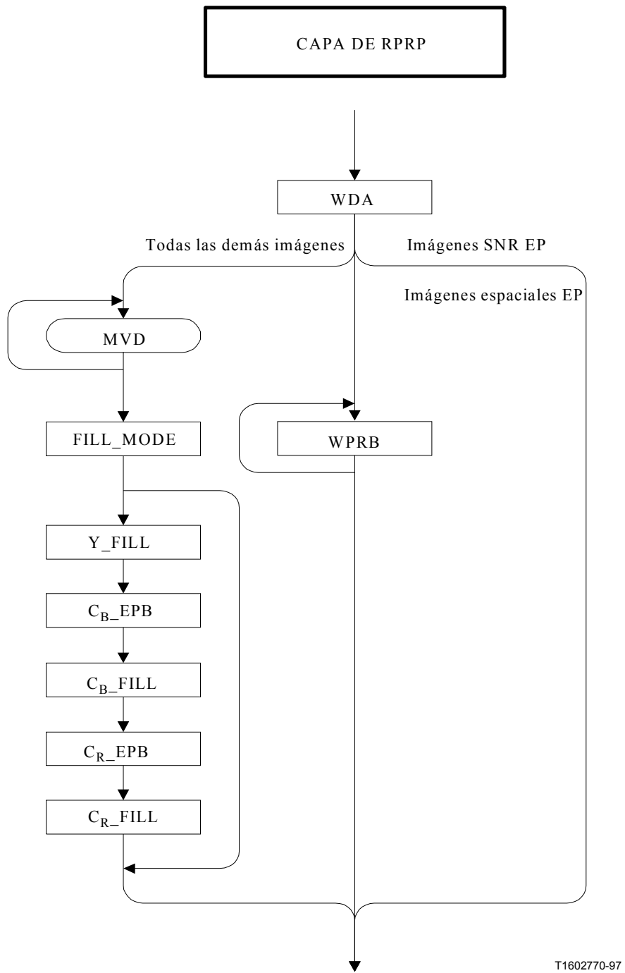
Figura 6/H.263 – Diagrama de sintaxis para el tren de bits de vídeo (parte 6 de 7)
