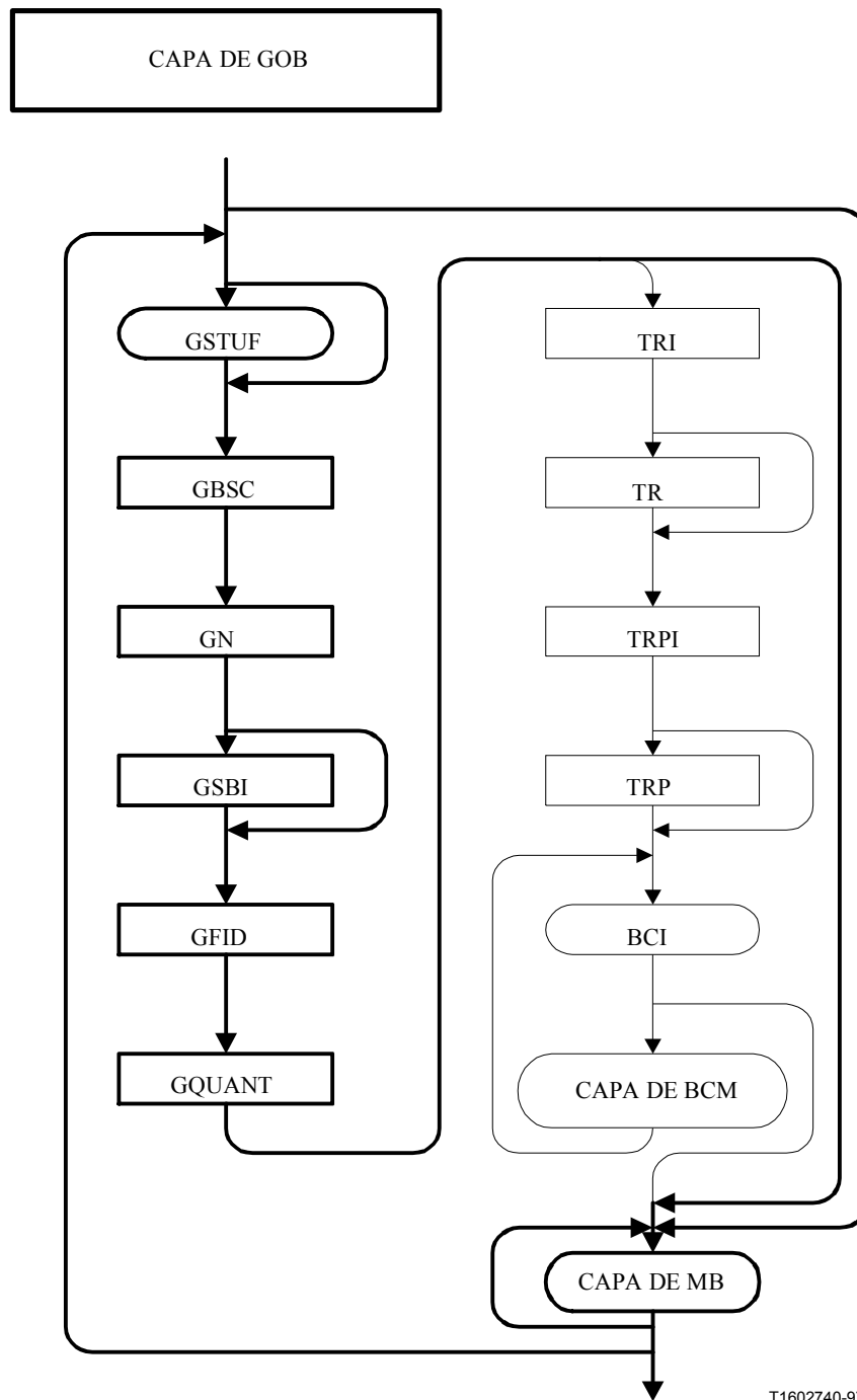
Figura 6/H.263 – Diagrama de sintaxis para el tren de bits de vídeo (parte 3 de 7)
