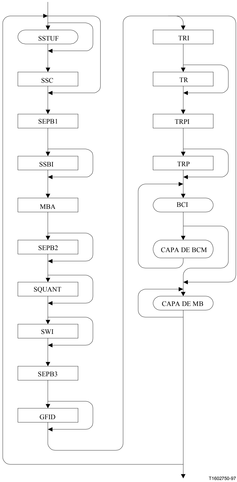
Figura 6/H.263 – Diagrama de sintaxis para el tren de bits de vídeo (parte 4 de 7)
