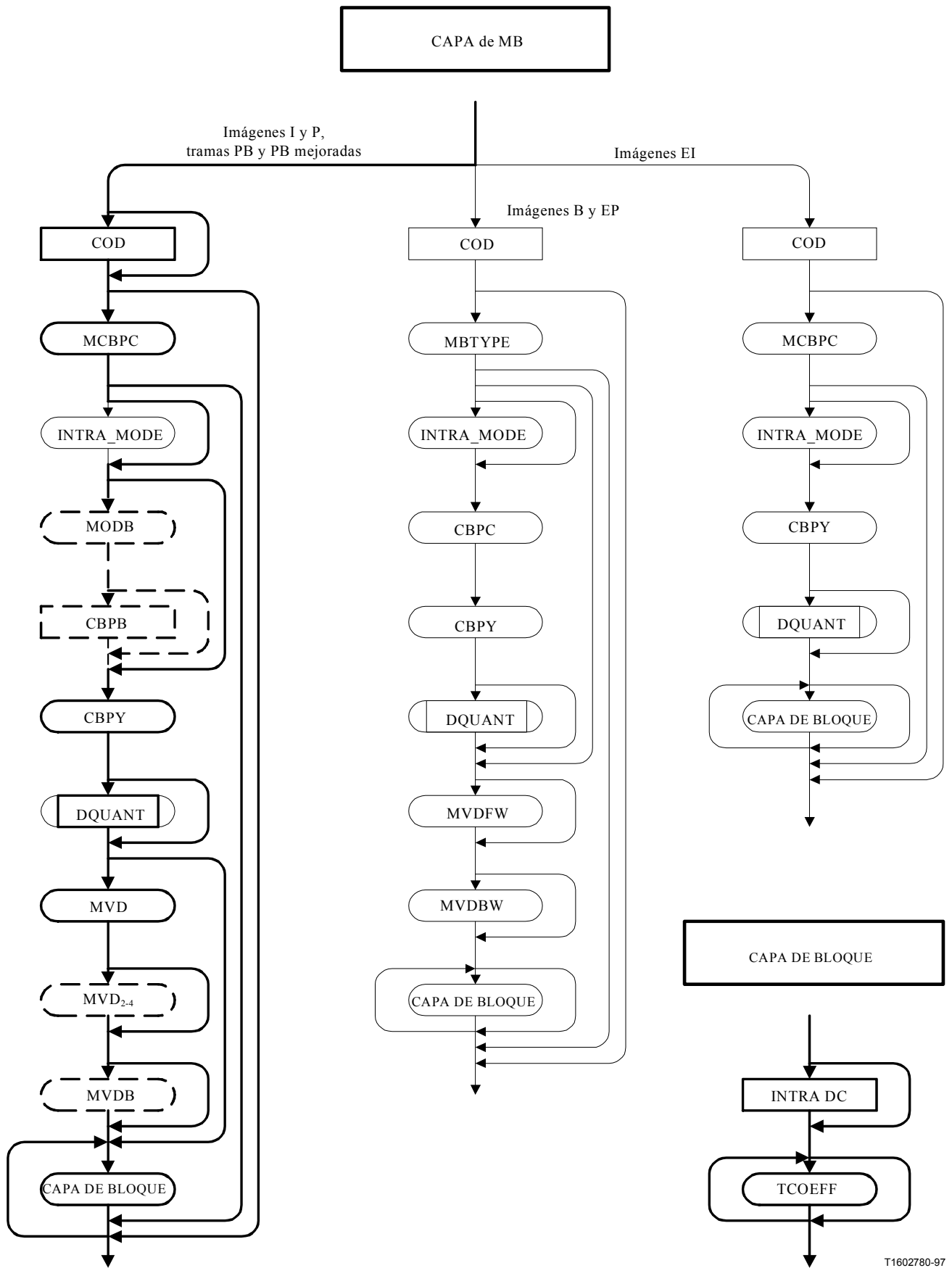
Figura 6/H.263 – Diagrama de sintaxis para el tren de bits de vídeo (parte 7 de 7)
