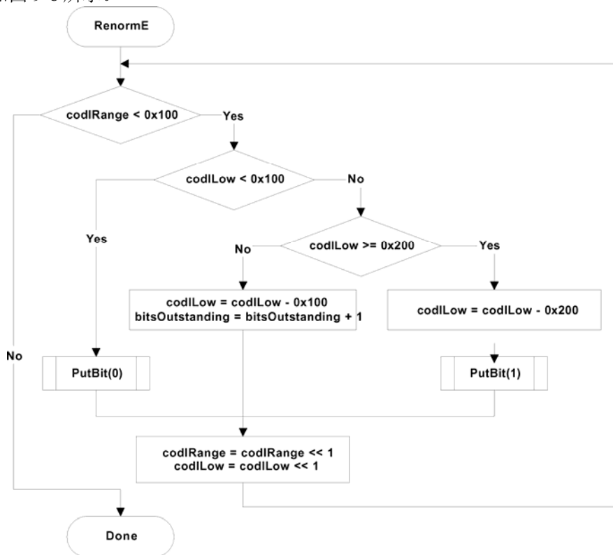
图 9-8— 编码器重归一化流程图
