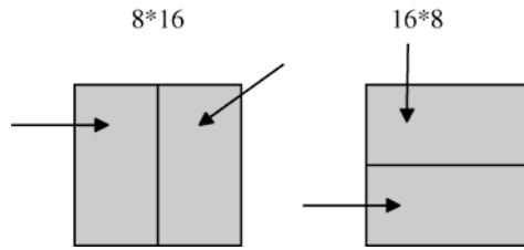
图 8-3—带方向的分段预测（资料性）
