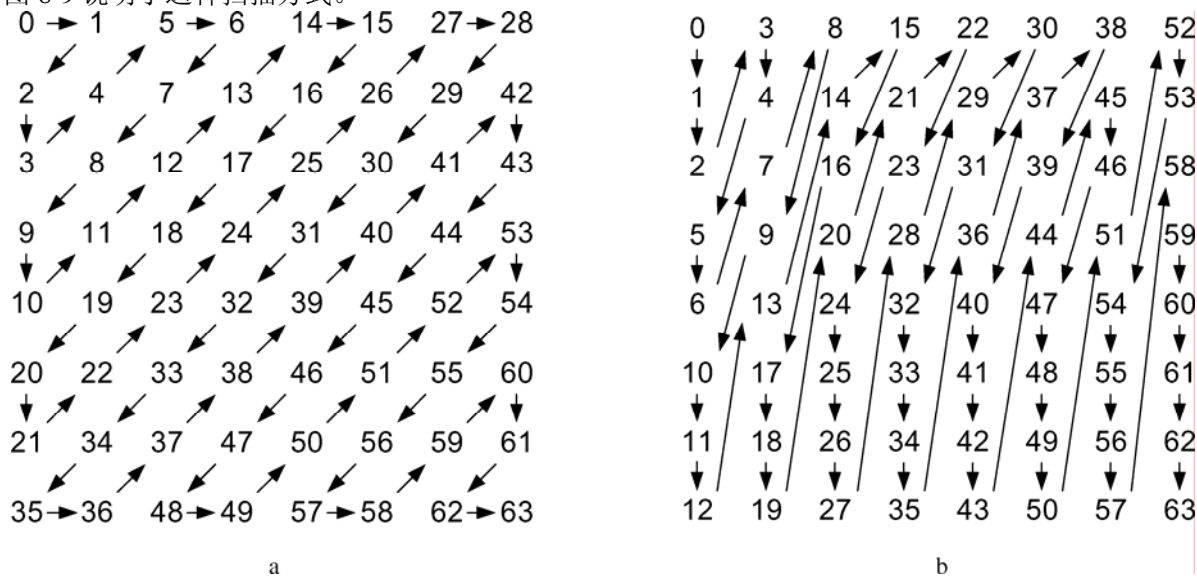
图 8-9— 8 \times 8 块扫描 (a) 8 \times 8 Z 型扫描 (b) 8 \times 8 域扫描 (资料性)
