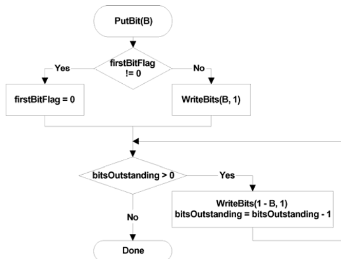
图 9-9— PutBit(B)流程图
