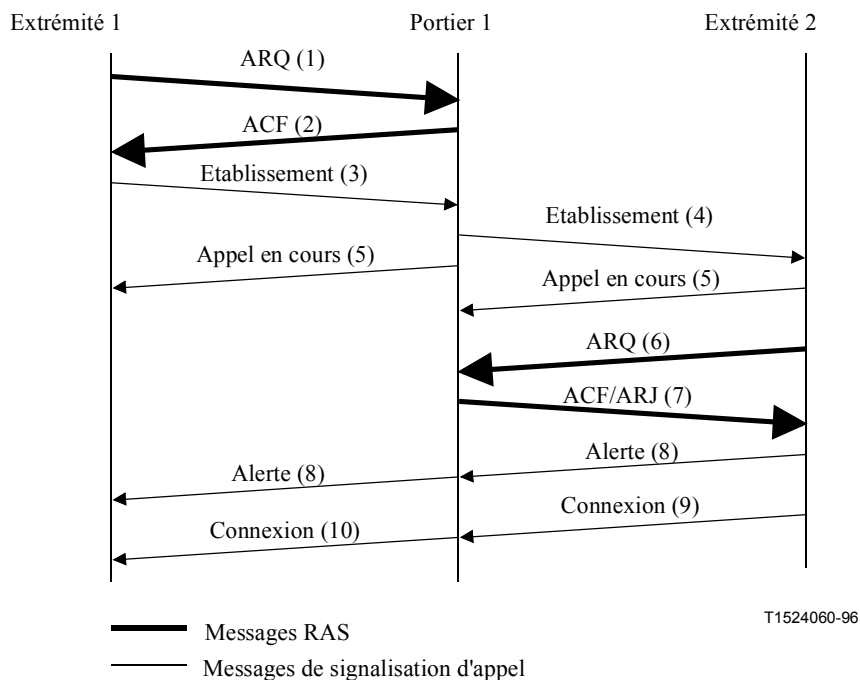
Figure 31/H.323 – Enregistrement des deux extrémités auprès du même portier – Signalisation d'appel indirecte par l'intermédiaire du portier
