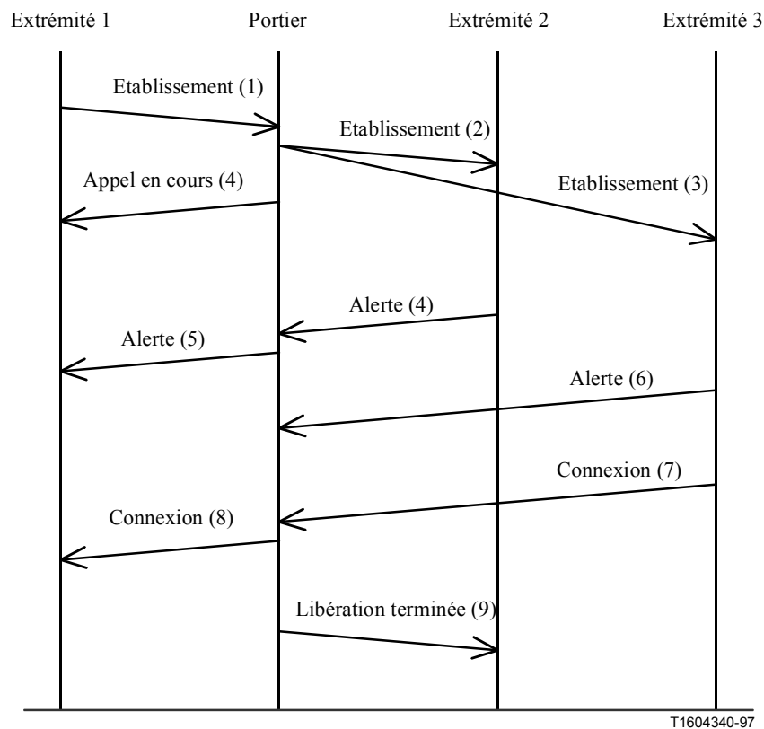
Figure III.2/H.323 – Exemple de localisation d'utilisateur par signalisation H.225.0/Q.931 (la signalisation RAS n'est pas représentée pour plus de clarté)
