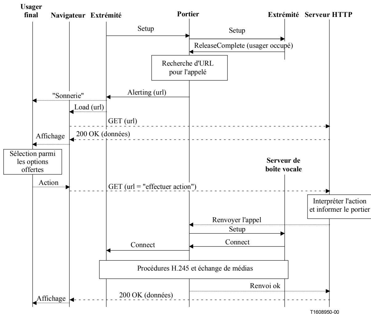
Figure K.5/H.323 – Commande de service associée à l'appel, routé par portier
