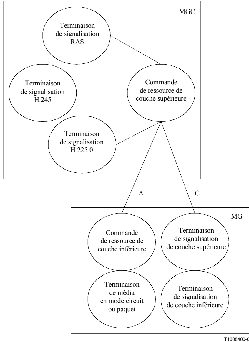
Figure 8/H.323 – Passerelle FAS avec signalisation H.323 dans la passerelle de support
