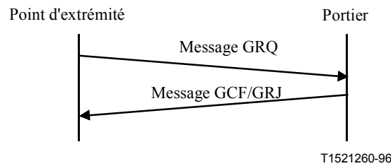
Figure 23/H.323 – Recherche automatique
