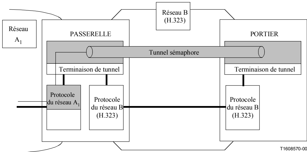
Figure 54/H.323 – Canalisation en tunnel de la signalisation entre une passerelle et une terminaison de tunnel située dans un portier
