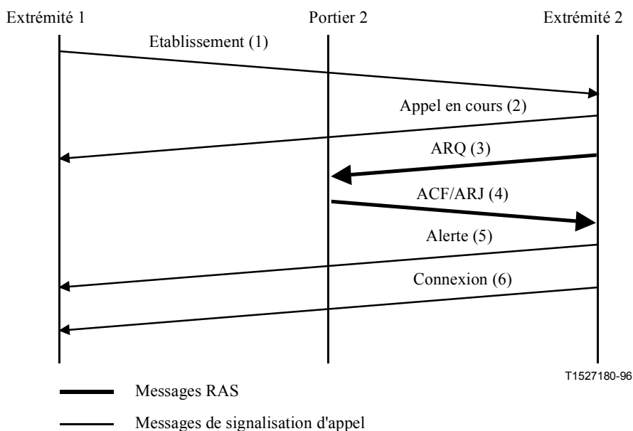
Figure 34/H.323 – Enregistrement de la seule extrémité appelée – Signalisation d'appel directe
