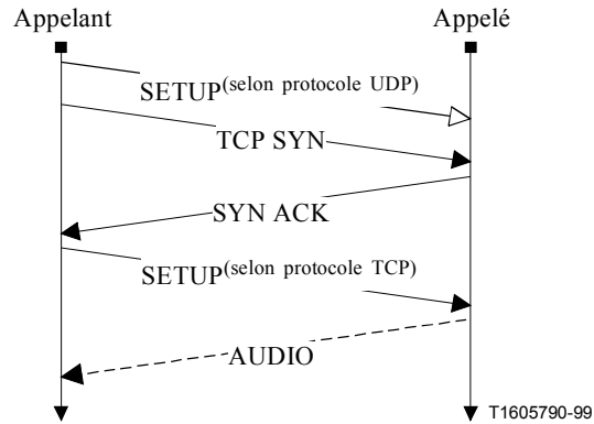
Figure E.25/H.323 – Flux d'informations lorsque le protocole UDP n'est pas accepté
