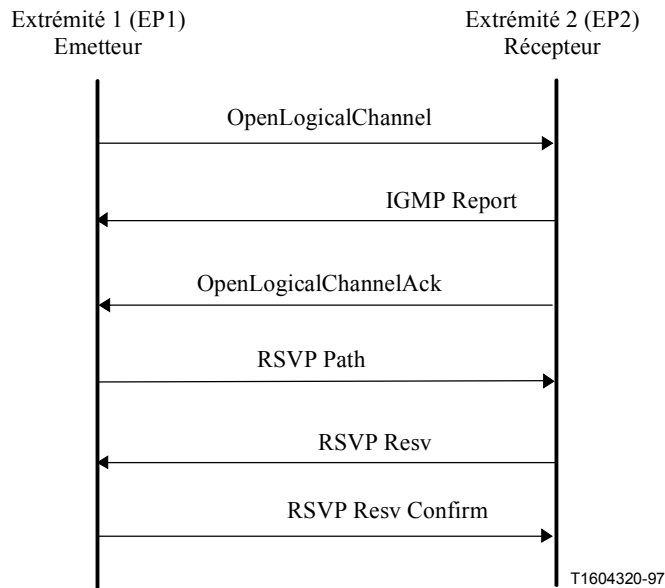
Figure II.4/H.323 – Séquence des messages pour l'ouverture d'une voie logique multidiffusée avec protocole RSVP
