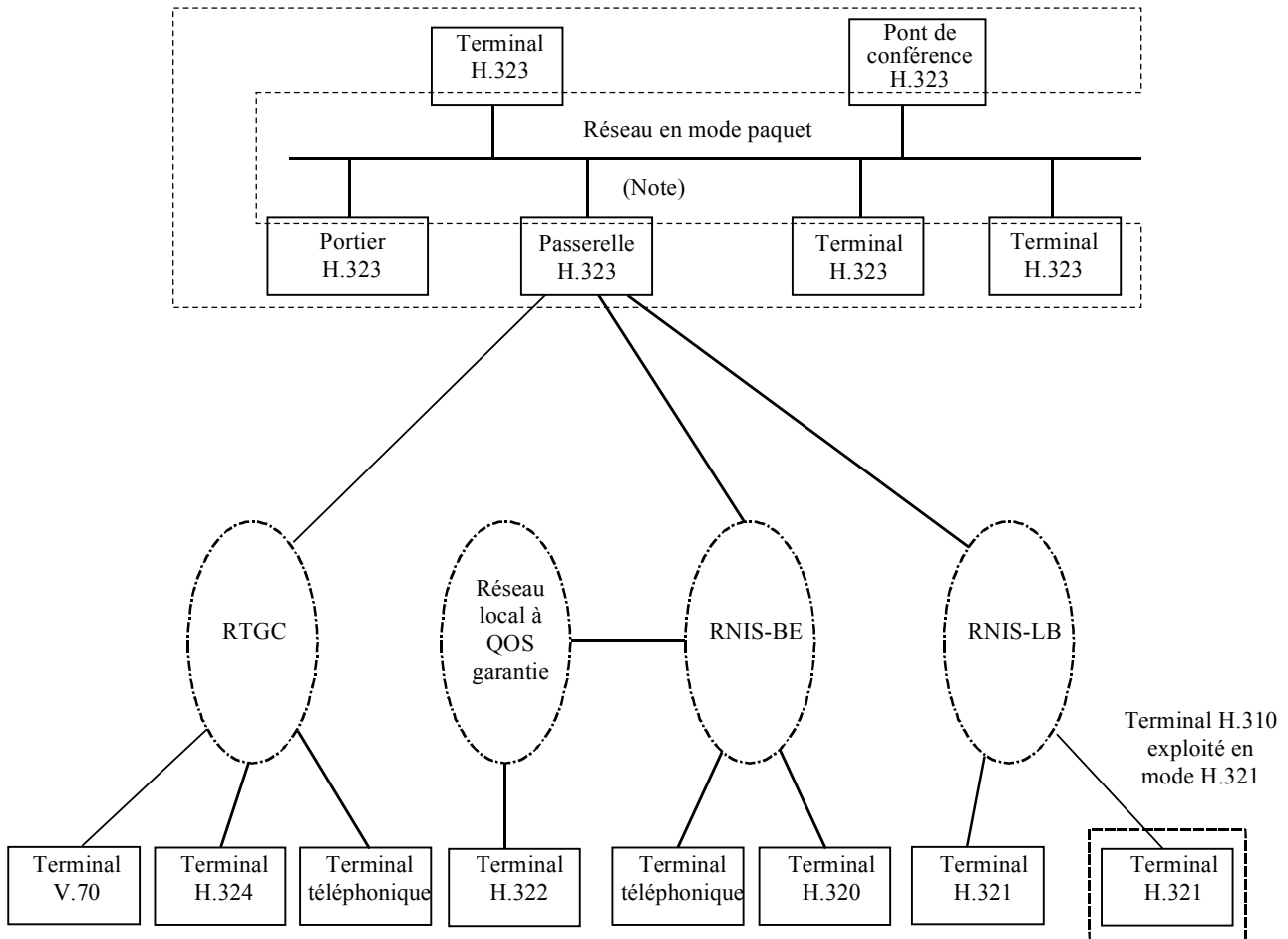
Figure 1/H.323 – Interopérabilité des terminaux H.323
