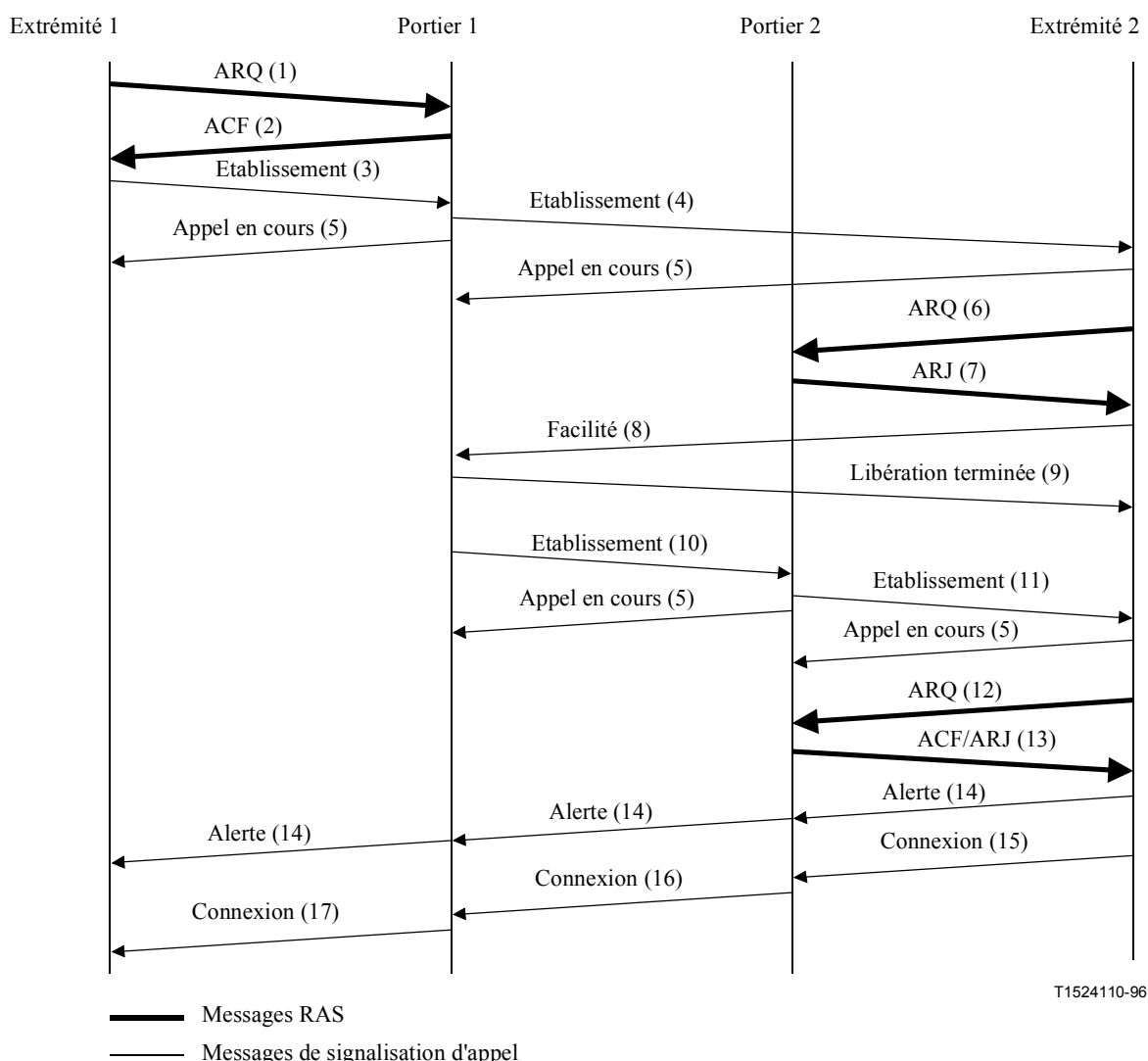
Figure 39/H.323 – Enregistrement des deux extrémités – Utilisation de la signalisation d'appel indirecte par les deux portiers
