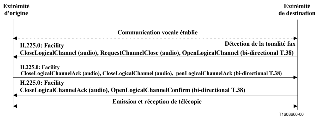
Figure D.11/H.323 – Commutation correcte d'une communication vocale existante à une communication T.38 au moyen d'une seule voie média bidirectionnelle (TCP) avec mise en tunnel
