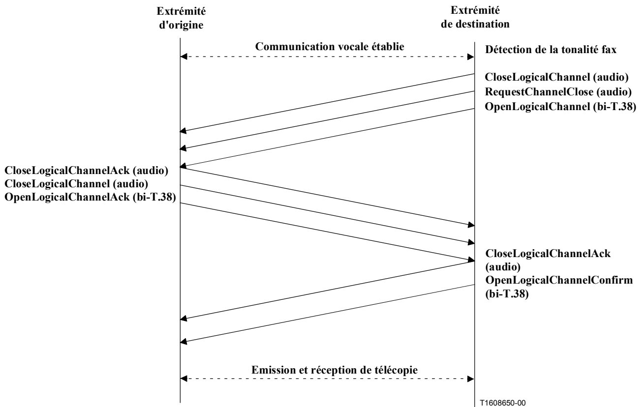
Figure D.10/H.323 – Commutation correcte d'une communication vocale existante à une communication T.38 au moyen d'une seule voie média bidirectionnelle (TCP) sans mise en tunnel
