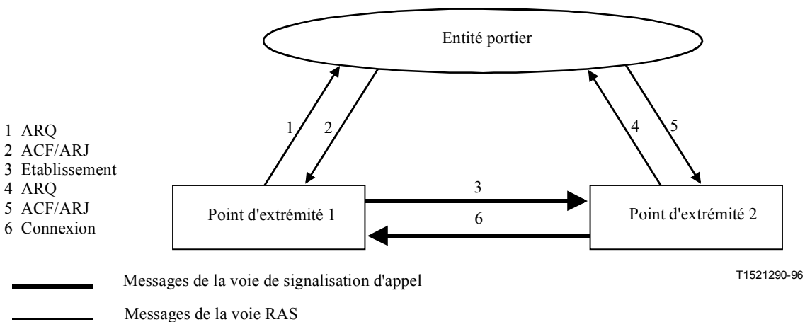
Figure 26/H.323 – Signalisation d'appel directe entre extrémités
