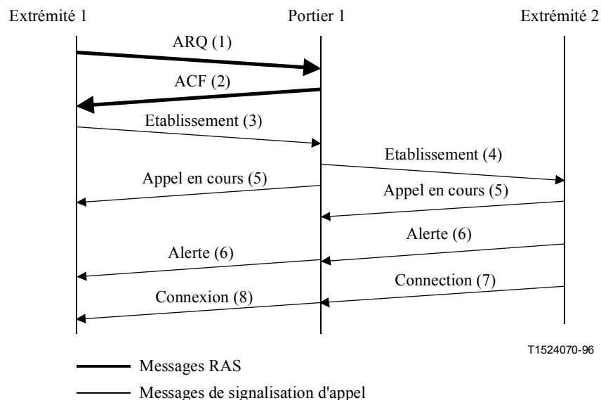
Figure 33/H.323 – Enregistrement de la seule extrémité appelante – Signalisation d'appel indirecte par l'intermédiaire du portier
