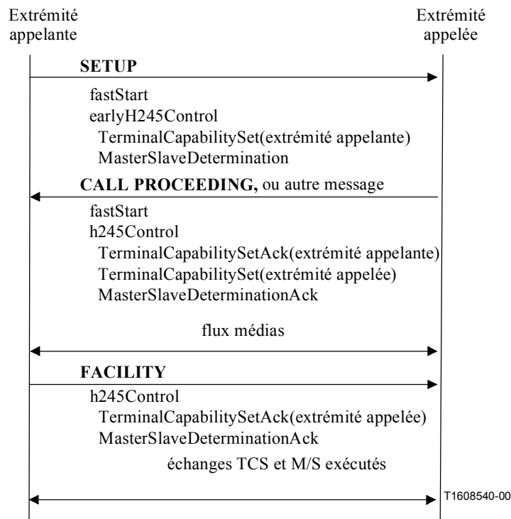
Figure 41/H.323 – Initiation d'une mise en tunnel H.245 en parallèle – sans échec
