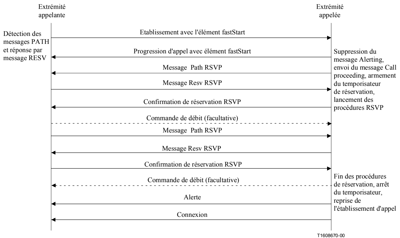
Figure II.6/H.323 – Synchronisation RSVP avec utilisation de la procédure FastConnect
