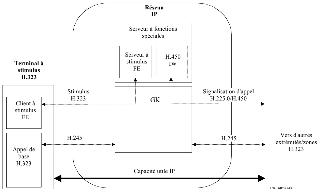
Figure L.2/H.323 – Exemple de configuration conforme à l'Annexe L conjointement avec le modèle de signalisation acheminé par le portier
