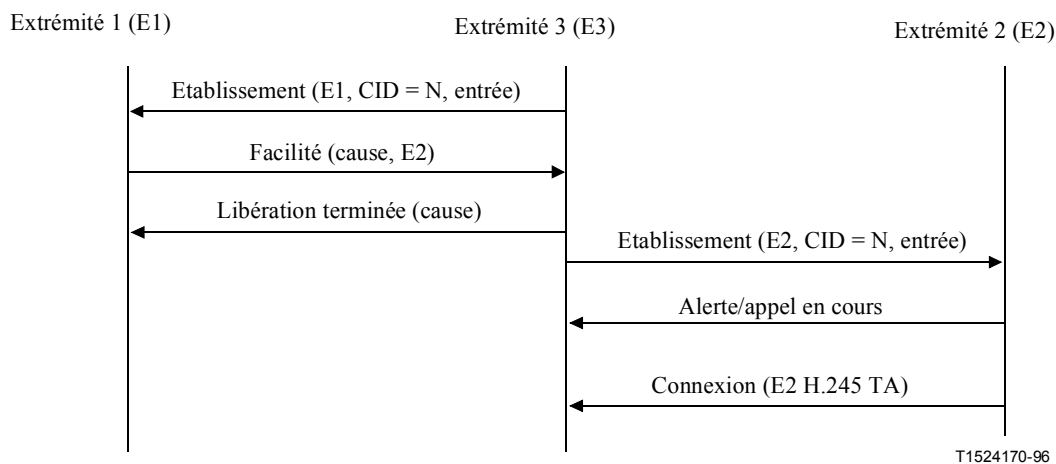
Figure 48/H.323 – Signalisation autre que par le contrôleur multipoint pour l'entrée dans une conférence
