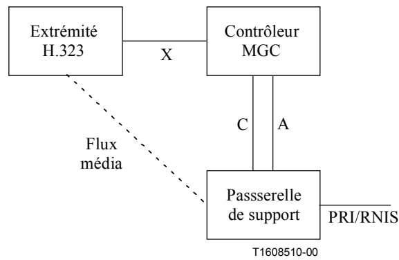
Figure 19/H.323 – Passerelle décomposée et extrémité H.323
