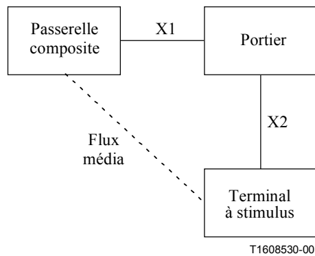
Figure 21/H.323 – Passerelle composite et terminal à stimulus
