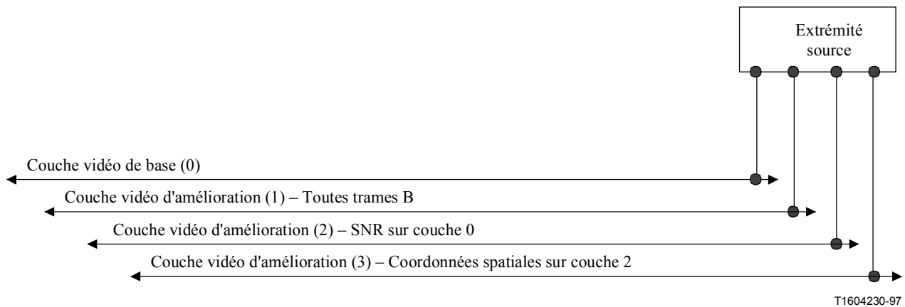
Figure B.1/H.323 – Modèle stratifié en couches vidéo
