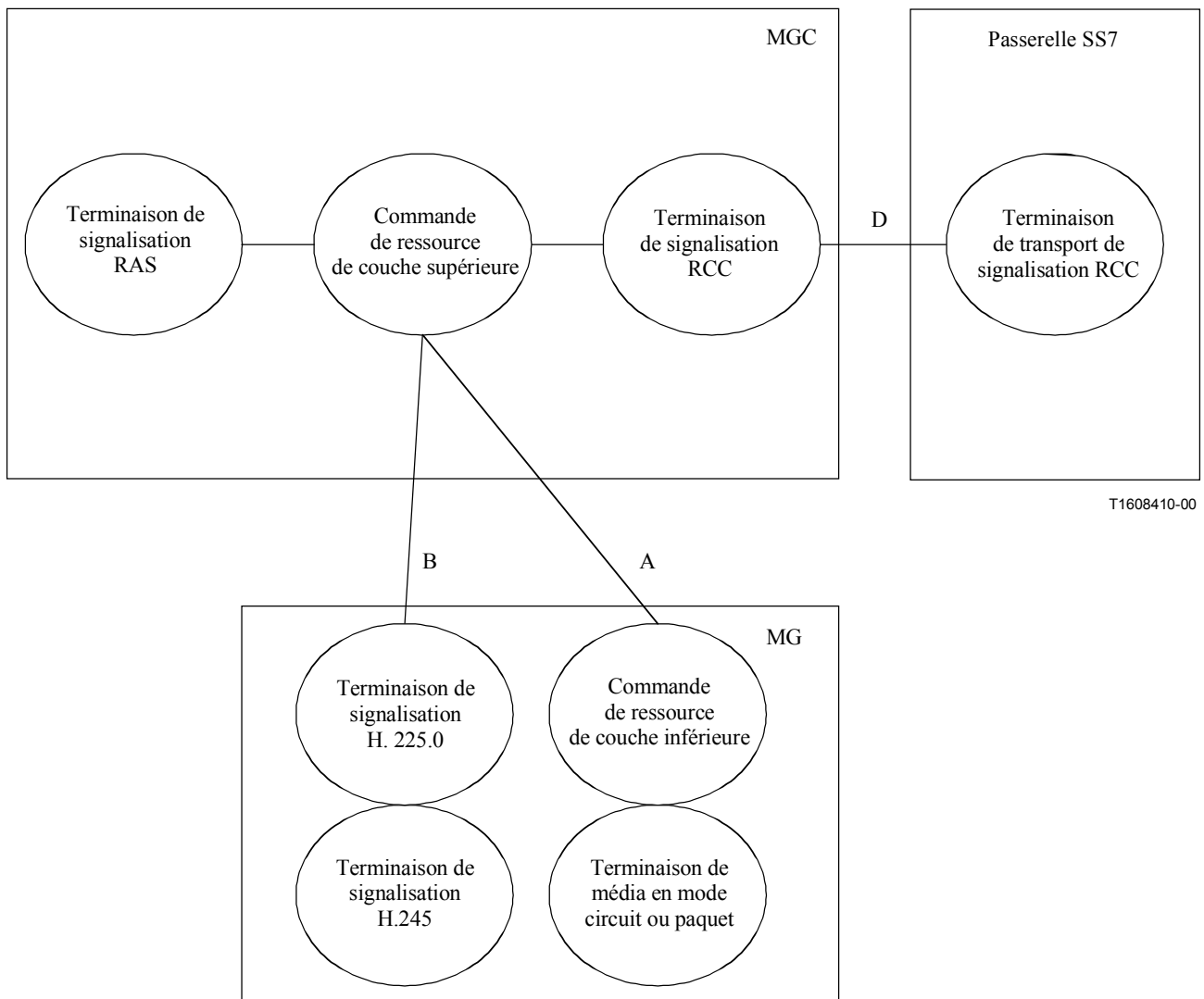
Figure 9/H.323 – Signalisation SS7 reçue dans la passerelle de support
