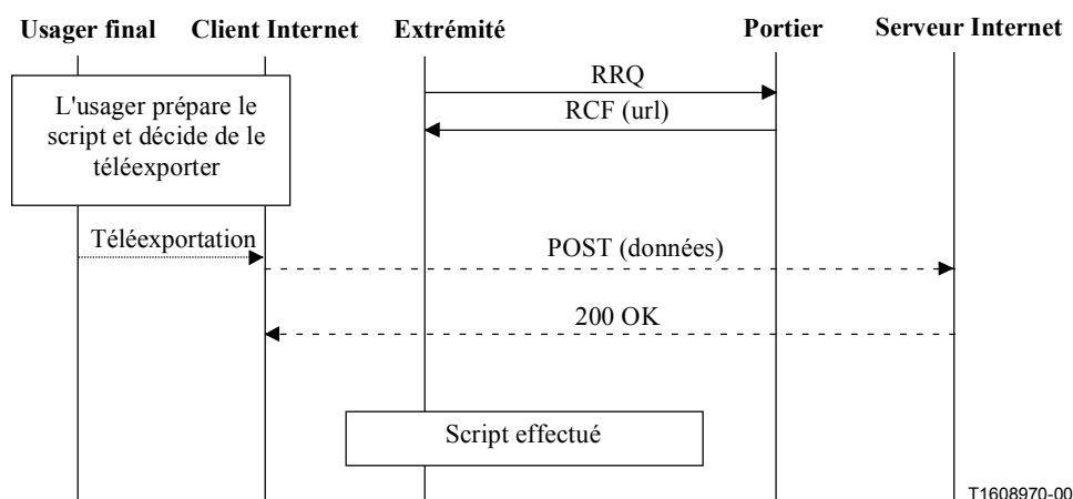
Figure K.7/H.323 – Commande de service non associée à l'appel, téléexportation de script
