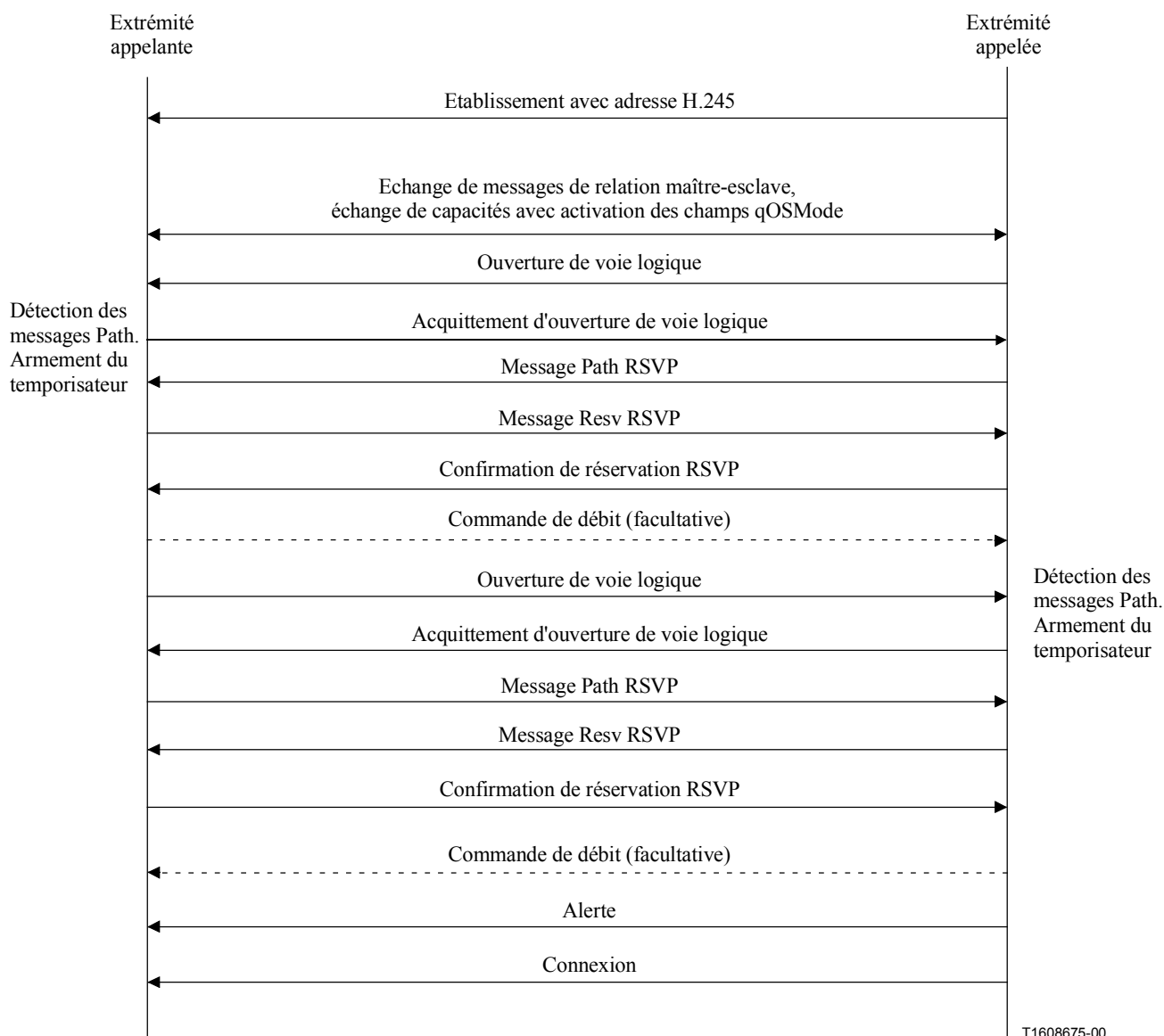
Figure II.5/H.323 – Synchronisation RSVP sans utilisation de la procédure FastConnect
