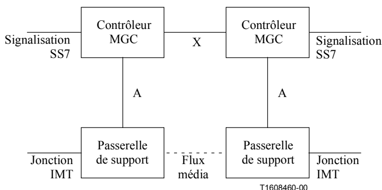
Figure 14/H.323 – Décomposition de deux passerelles de jonction de fournisseur de service
