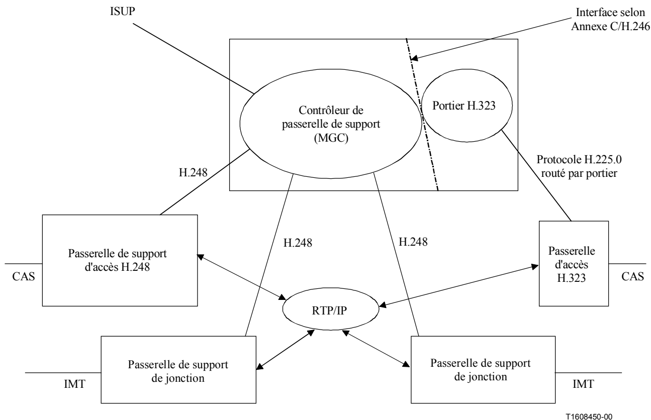
Figure 13/H.323 – Relation entre protocoles H.323 et H.248
