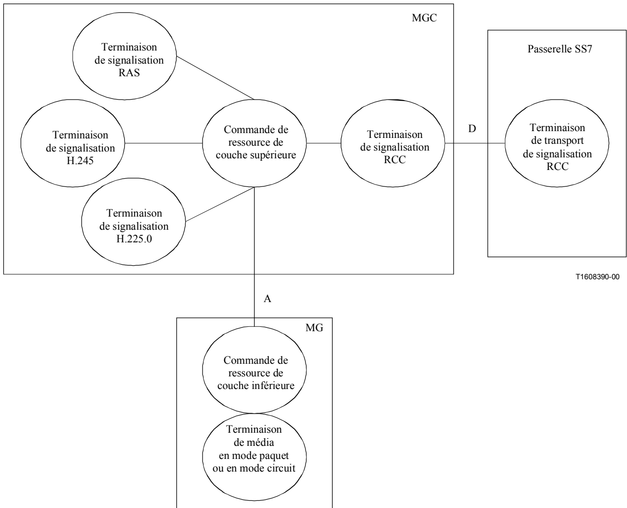
Figure 7/H.323 – Décomposition de passerelle SS7
