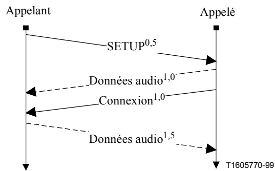
Figure E.23/H.323 – Flux d'informations pour l'établissement d'appel utilisant le protocole UDP
