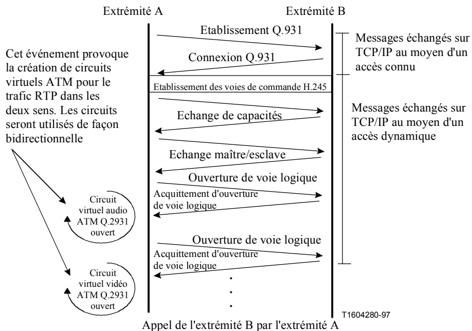
Figure C.3/H.323 – Etablissement d'une communication H.323 montrant l'utilisation bidirectionnelle d'un circuit virtuel ATM
