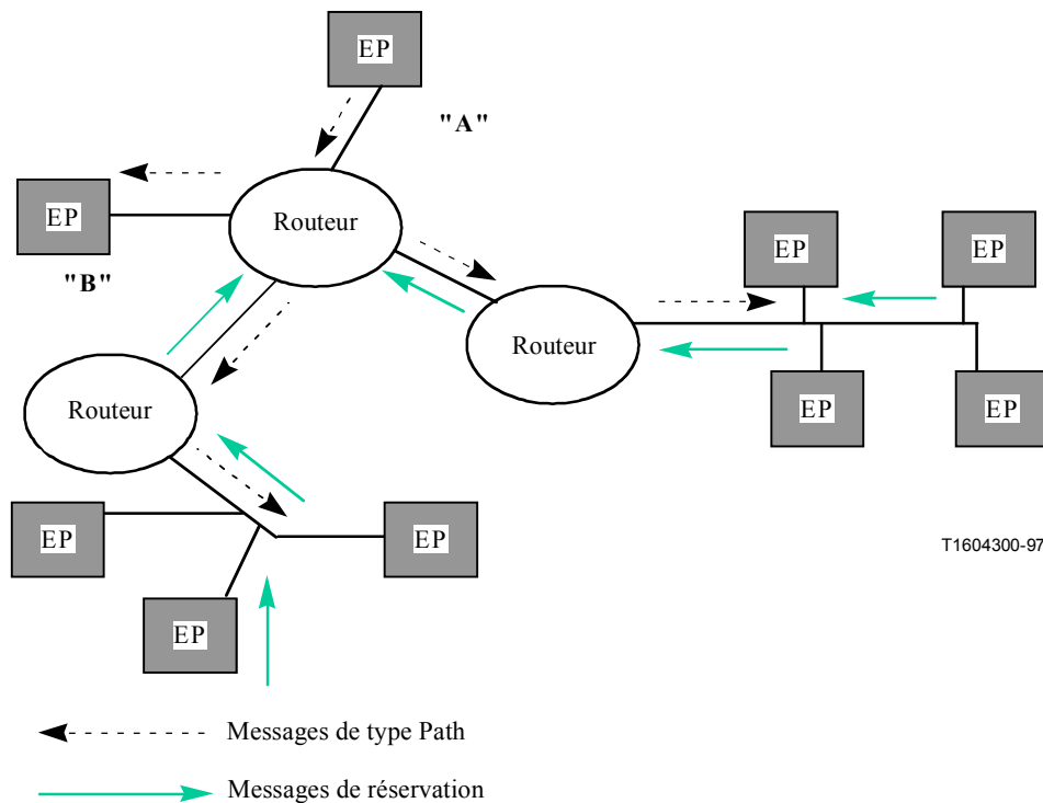
Figure II.2/H.323 – Réserveation de ressources pour une connexion point à multipoint
