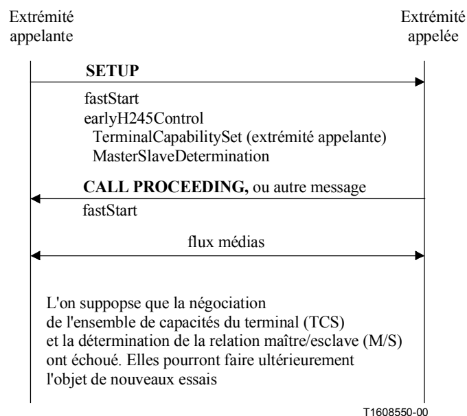
Figure 42/H.323 – Initiation d'une mise en tunnel H.245 en parallèle – avec échec
