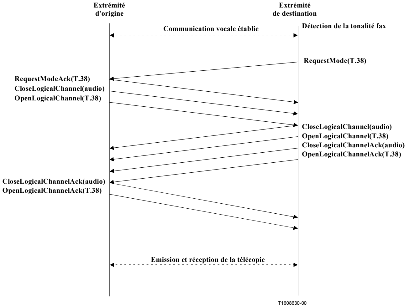
Figure D.8/H.323 – Commutation correcte d'une communication vocale existante à une communication T.38 au moyen de deux voies médias unidirectionnelles sans mise en tunnel
