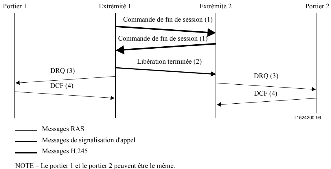
Figure 51/H.323 – Déclenchement de la libération de la communication par l'extrémité
