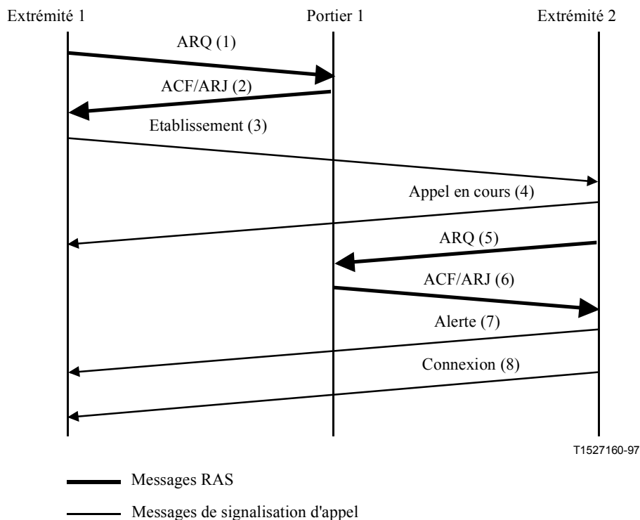
Figure 30/H.323 – Enregistrement des deux extrémités auprès du même portier – Signalisation d'appel directe
