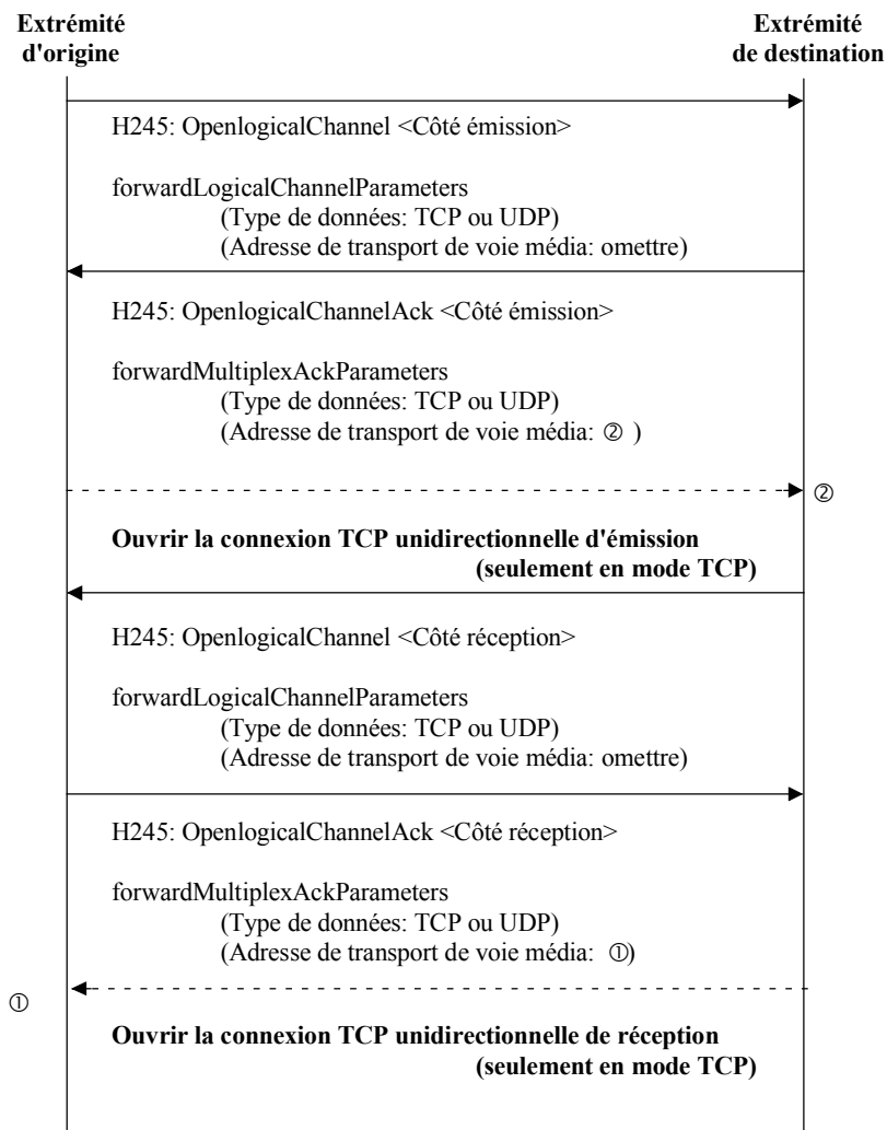
Figure D.6/H.323 – Deux voies unidirectionnelles sans connexion rapide
