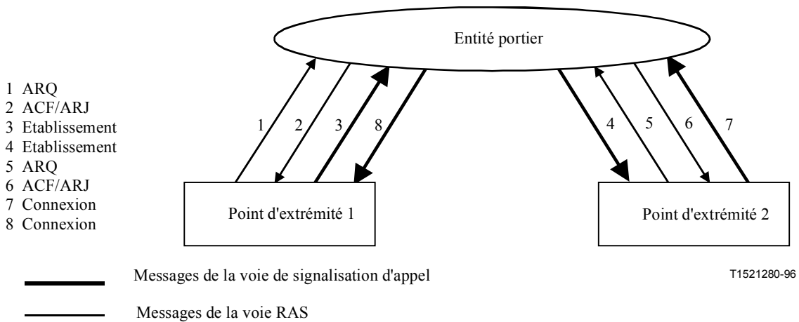
Figure 25/H.323 – Signalisation d'appel acheminée par le portier
