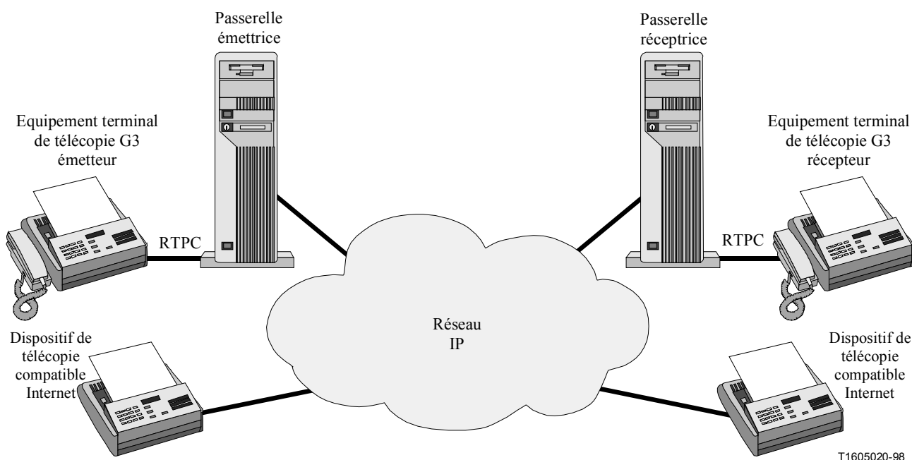
Figure D.1/H.323 – Modèle pour la transmission de télécopie sur des réseaux IP
