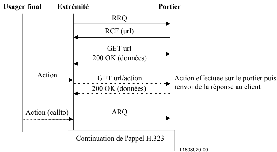
Figure K.2/H.323 – Exemple de commande de service non associée à l'appel
