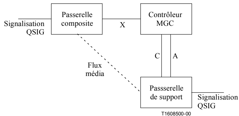
Figure 18/H.323 – Exemple de canalisation en tunnel du protocole QSIG
