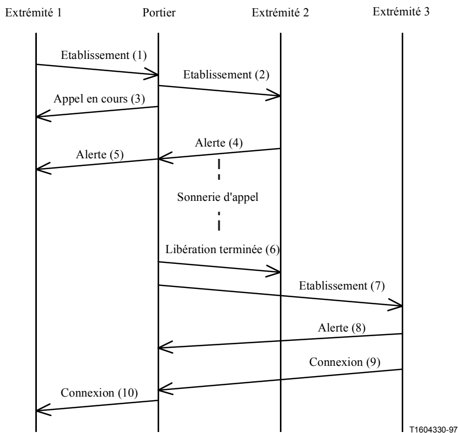
Figure III.1/H.323 – Exemple de localisation d'utilisateur par signalisation H.225.0/Q.931 (la signalisation RAS n'est pas représentée pour plus de clarté)
