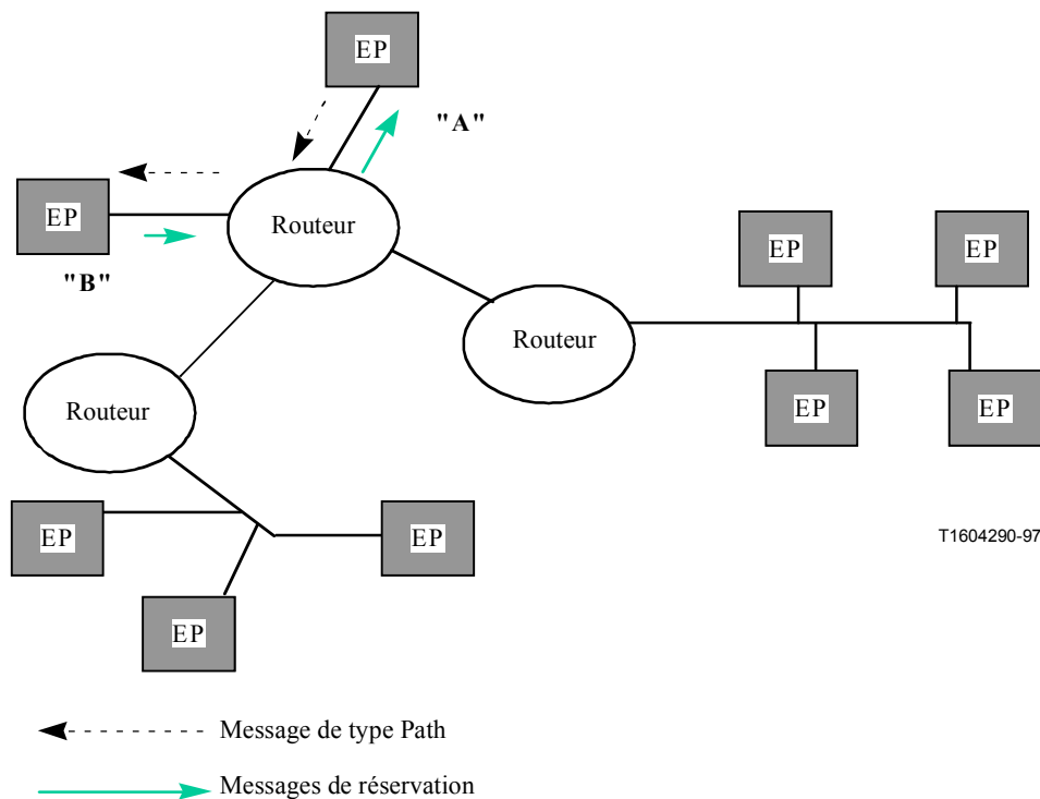
Figure II.1/H.323 – Réserveation de ressources pour une connexion point à point
