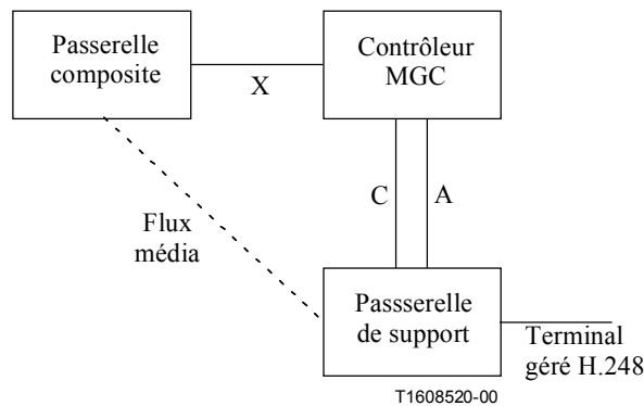
Figure 20/H.323 – Passerelle composite et terminal géré H.248
