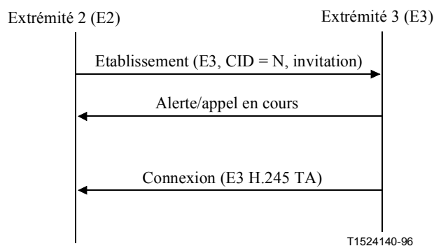
Figure 45/H.323 – Signalisation d'invitation du contrôleur multipoint
