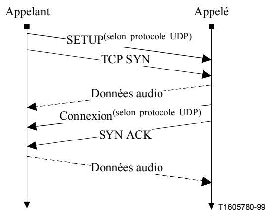
Figure E.24/H.323 – Flux d'informations pour la procédure mixte TCP et UDP
