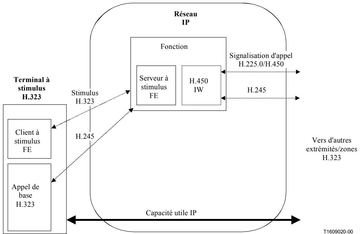
Figure L.1/H.323 – Exemple de configuration conforme à l'Annexe L conjointement avec le modèle de signalisation direct
