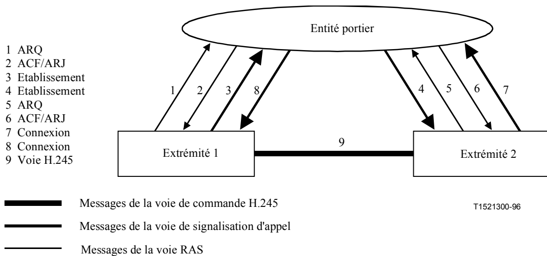
Figure 27/H.323 – Connexion directe de la voie de commande H.245 entre extrémités
