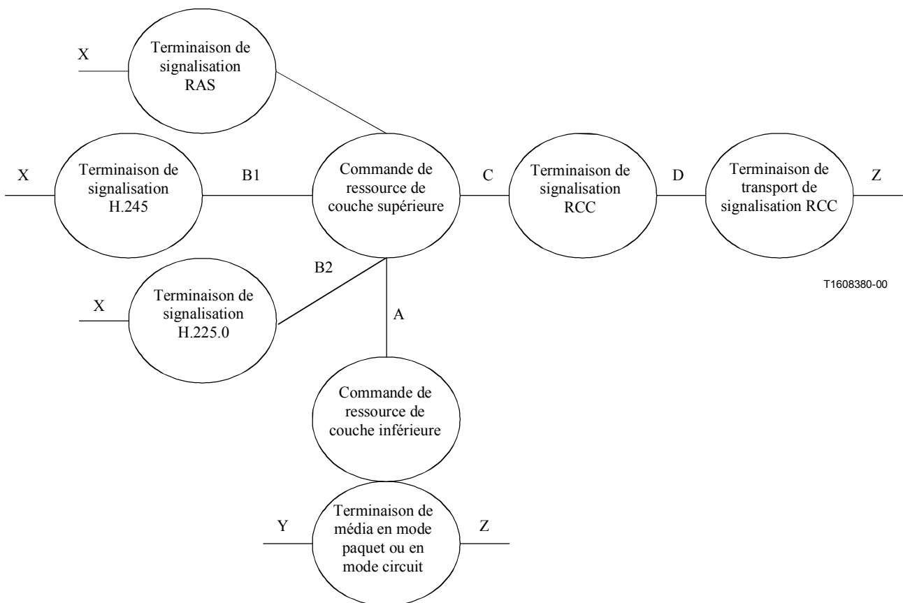
Figure 6/H.323 – Architecture fonctionnelle de la passerelle décomposée
