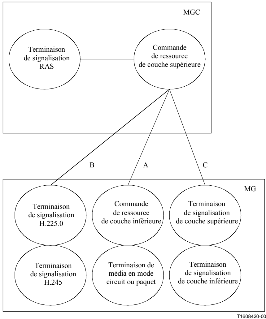
Figure 10/H.323 – Signalisations FAS et H.323 dans la passerelle de support
