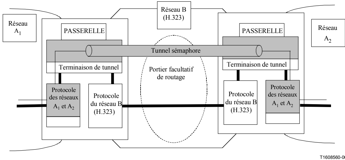
Figure 53/H.323 – Canalisation en tunnel de la signalisation entre passerelles
