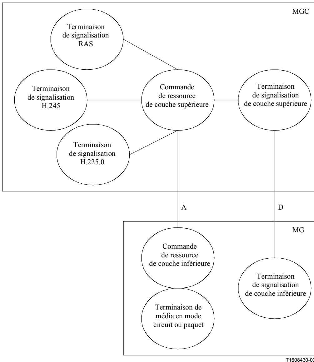
Figure 11/H.323 – Signalisation SS7 aboutissant dans la passerelle de support
