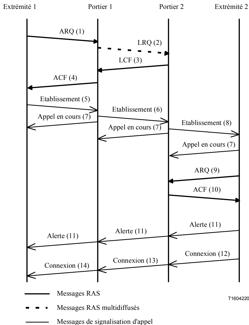
Figure 40/H.323 – Signalisation facultative de l'extrémité appelée
