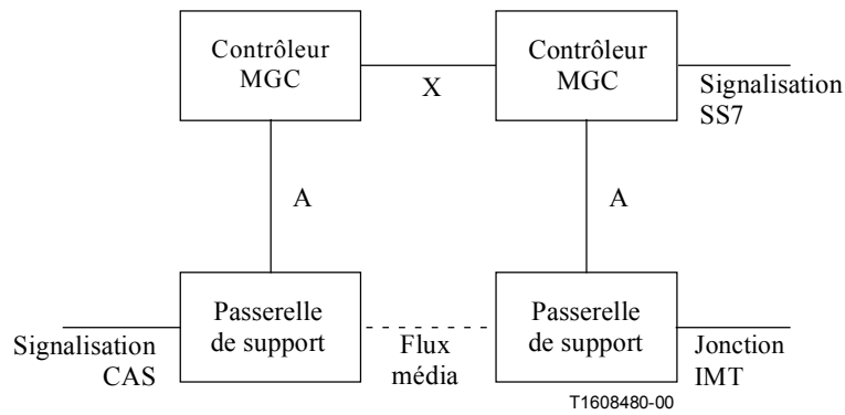
Figure 16/H.323 – Décomposition de passerelles d'accès et de jonction de fournisseur de services
