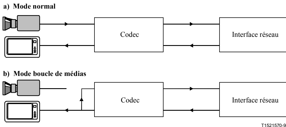
Figure 55/H.323 – Fonction de bouclage
