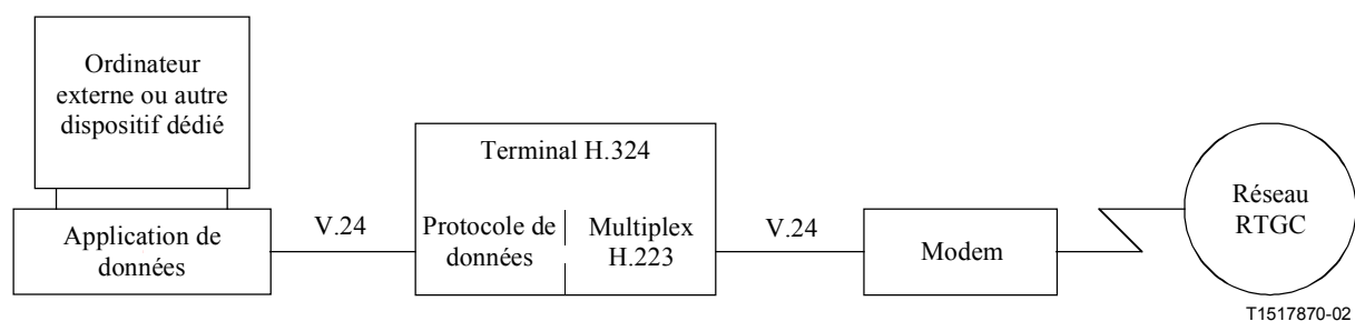
Figure 2/H.324 – Application de données – Interface de protocole de données
