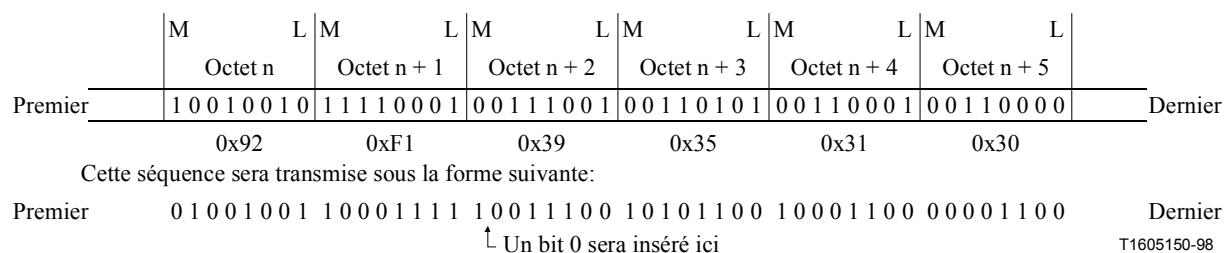
Figure I.3/H.324 – Exemple de séquence
