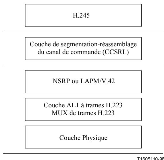
Figure C.2/H.324 – Pile de protocoles pour canal de commande H.324
