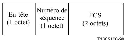
Figure A.3/H.324 – Format de la trame de réponse NSRP
