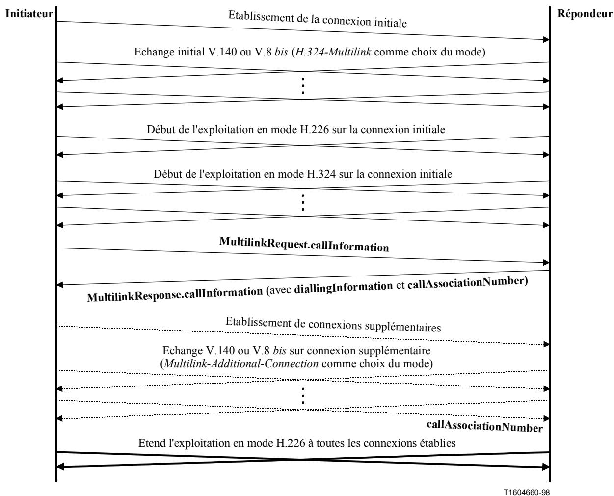
Figure F.2/H.324 – Diagramme séquentiel pour l'établissement d'une exploitation multiliasion
