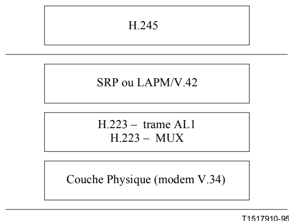
Figure A.1/H.324 – Pile de protocoles pour le canal de commande H.324
