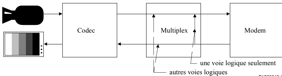
d) bouclage de voie logique
