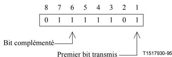
Figure B.1/H.324 – Octet de commande d'échappement pour la procédure de tunnel de trame HDLC
