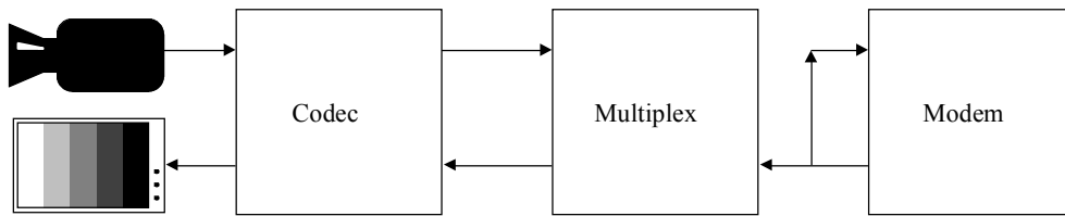
b) bouclage local du système
