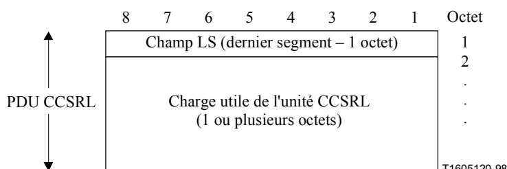
Figure C.3/H.324 – Format des unités PDU CCSRL
