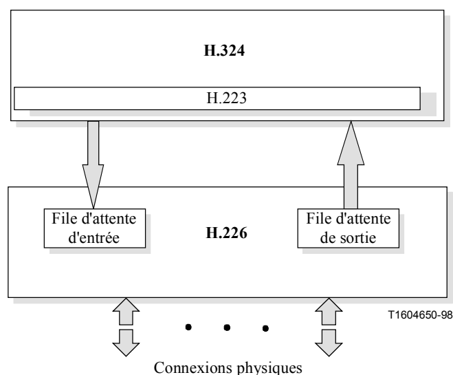
Figure F.1/H.324 – Modèle d'exploitation H.324 en mode multiliasion
