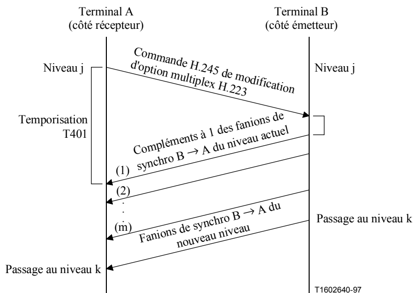
Figure C.1/H.324 – Procédure de modification de niveau ou d'option
