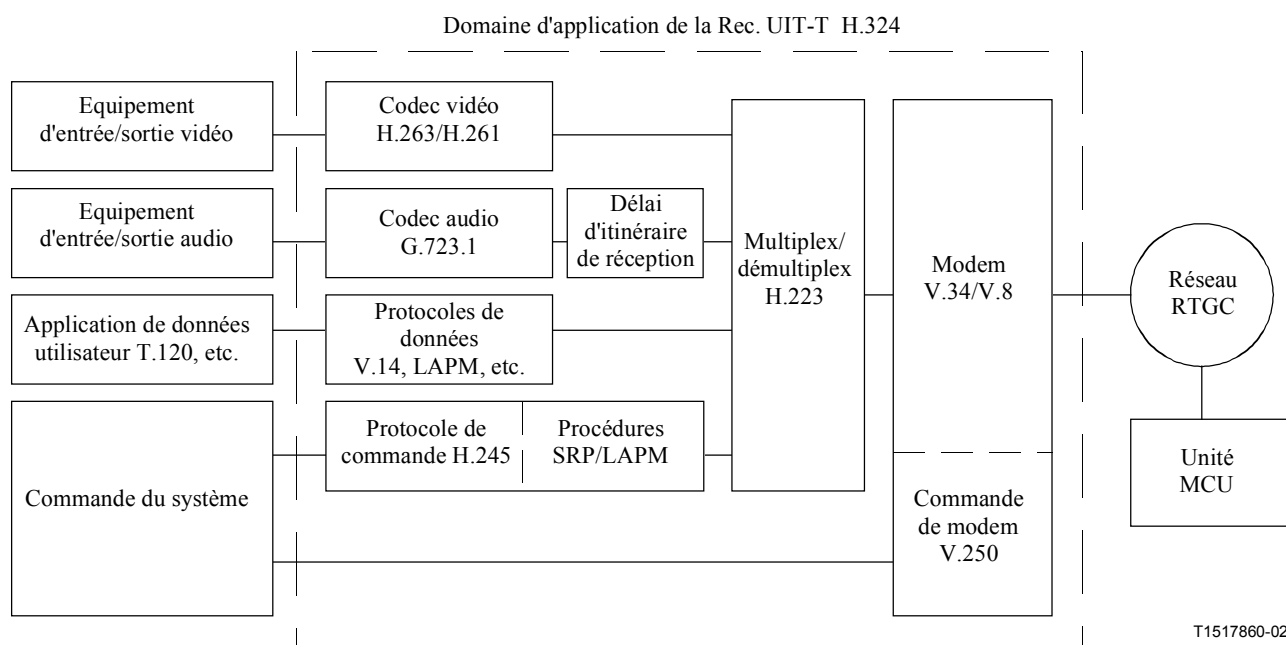
Figure 1/H.324 – Diagramme de principe d'un système multimédia H.324
