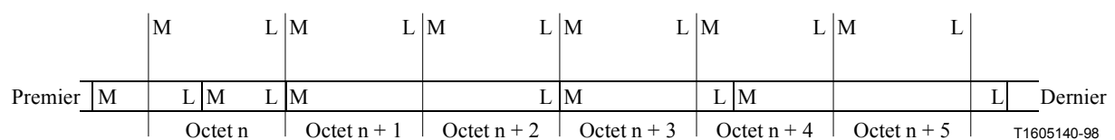
Figure I.2/H.324 – Découpage en octets de la séquence remise
