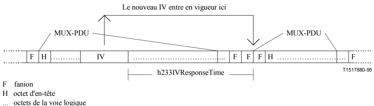
Figure 3/H.324 – Synchronisation du vecteur d'initialisation de chiffrement
