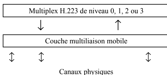
Figure H.1/H.324 – Aperçu général de la couche multiliasion mobile
