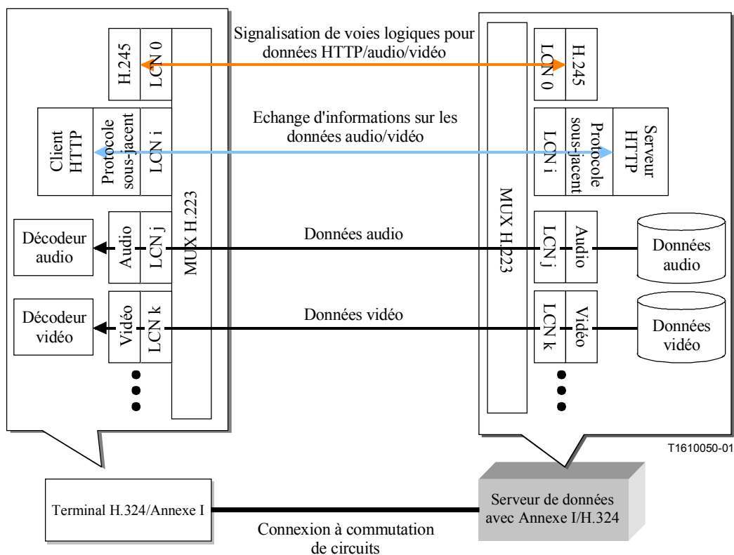
Figure I.1/H.324 – Application utilisant les capacités décrites à l'Annexe I/H.324
