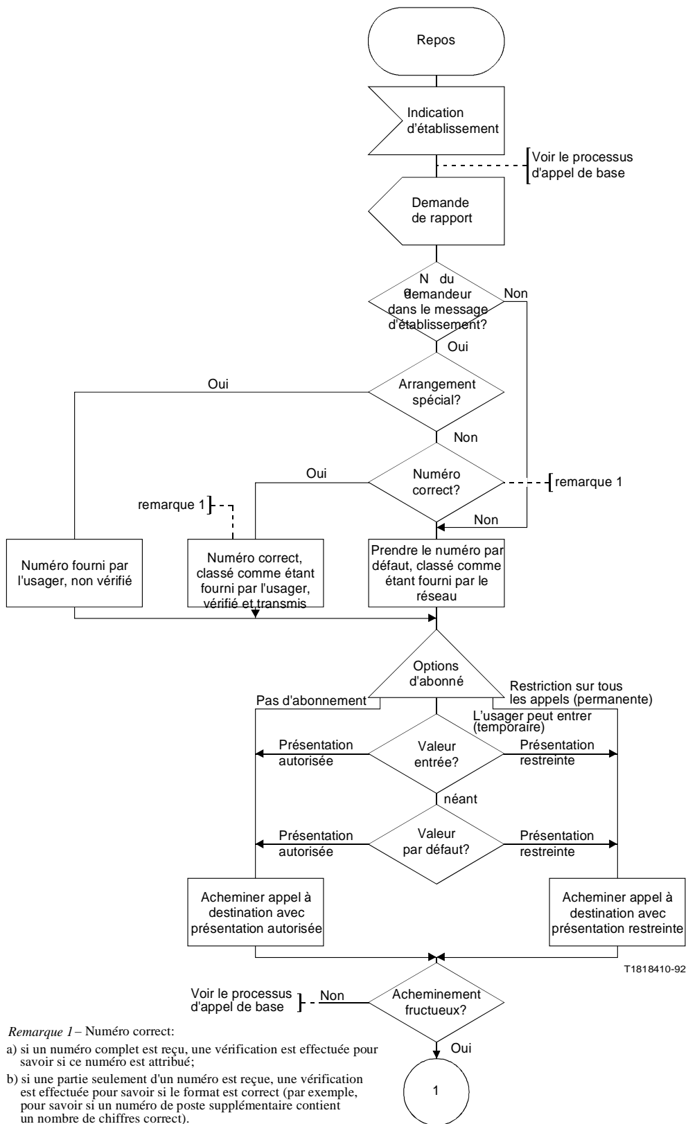
FIGURE 1/I.251.3 (feuille 1 sur 2) Diagramme SDL global pour présentation/restriction d'identification de la ligne appelante
