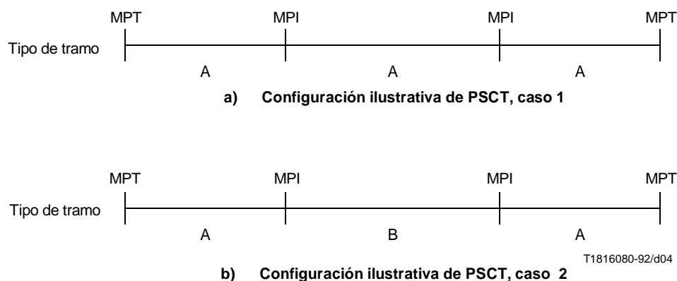
FIGURA B.1/I.355
