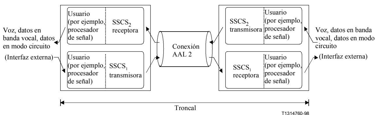
Figura 6-1/I.366.2 – Modelo de referencia de la SSCS para servicios de banda estrecha
