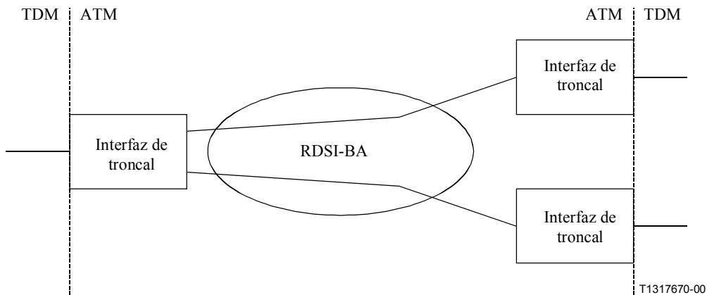
Figura 6-2a/I.366.2 – Ejemplo de troncalización de banda estrecha
