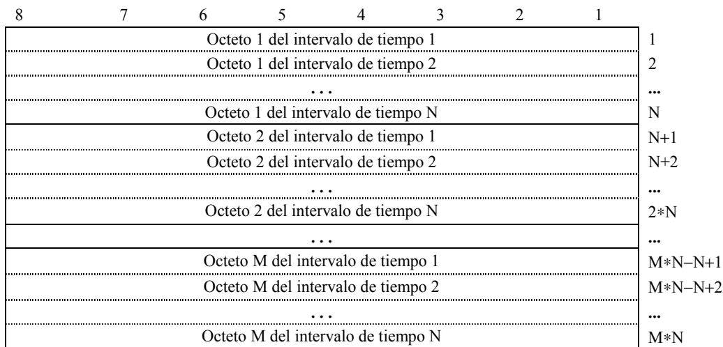
Figura J.1/I.366.2 – Formato de paquete de datos en modo circuito
