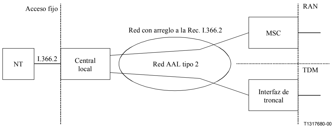
Figura 6-2b/I.366.2 – Ejemplo de troncalización de banda estrecha
