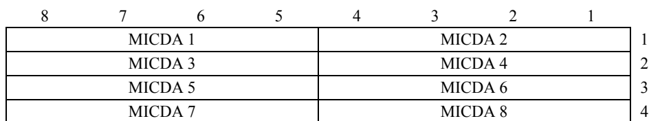
Figura E.2/I.366.2 – Formato de EDU G.726-32
