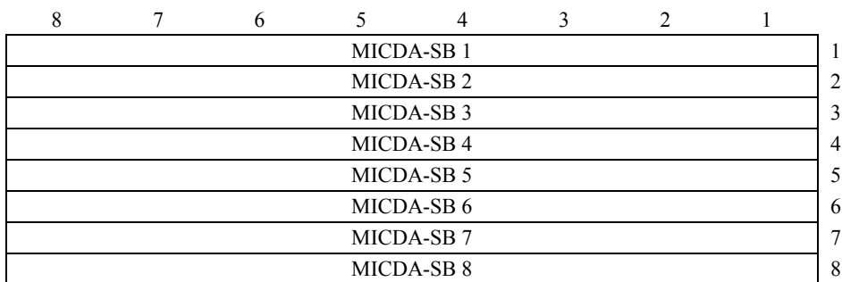
Figura C.1/I.366.2 – Formato de EDU G.722-64
