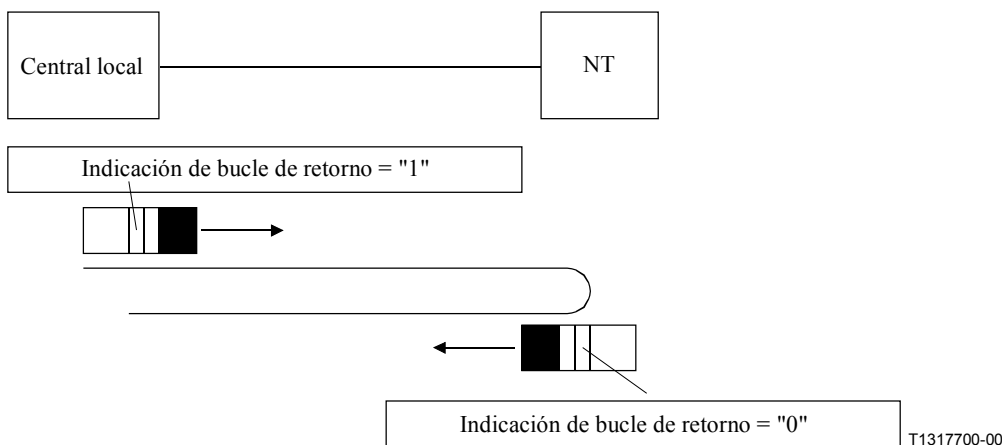
Figura N.4/I.366.2 – Bucle de retorno CID con la función LBI
