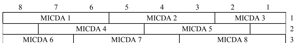
Figura E.3/I.366.2 – Formato de EDU G.726-24
