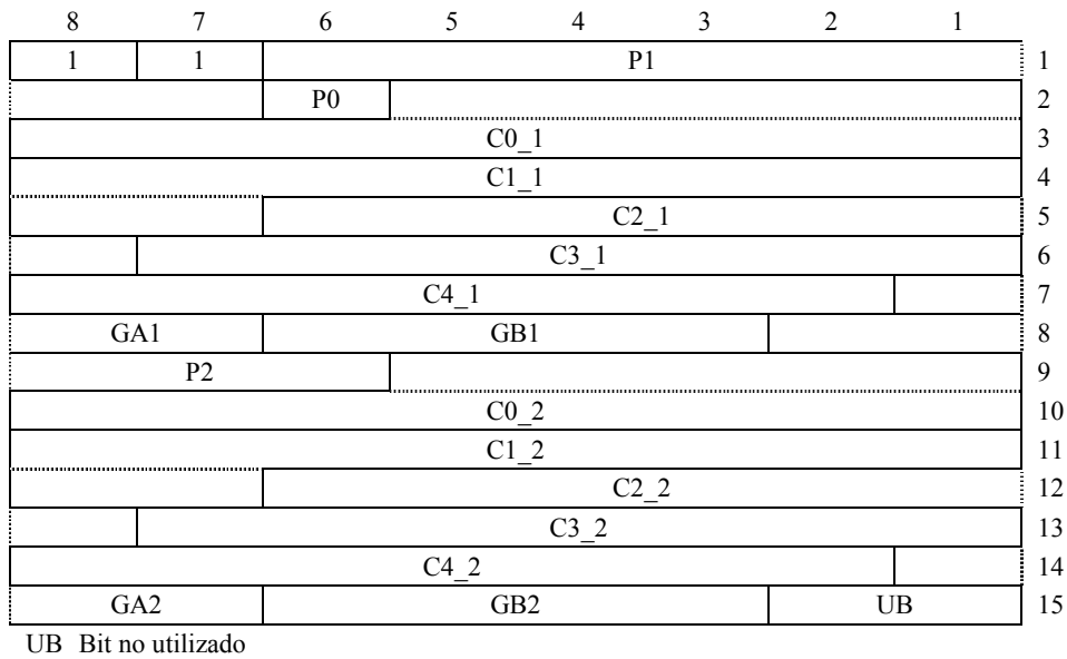
Figura H.4/I.366.2 – Formato de la unidad de datos de codificación G.729-12 para el modo adaptable hacia atrás (parte B)
