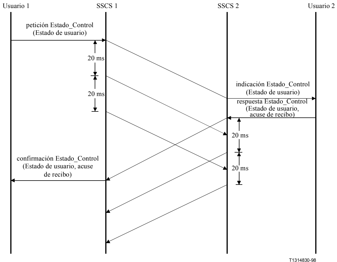
Figura O.2/I.366.2 – Flujo de mensaje control de estados de usuario
