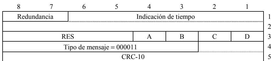
Figura L.1/L.366.2 – Formato de paquete bits de señalización asociada al canal
