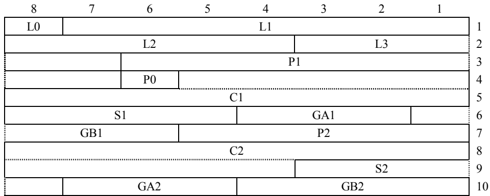
Figura H.1/I.366.2 – Formato de EDU G.729-8
