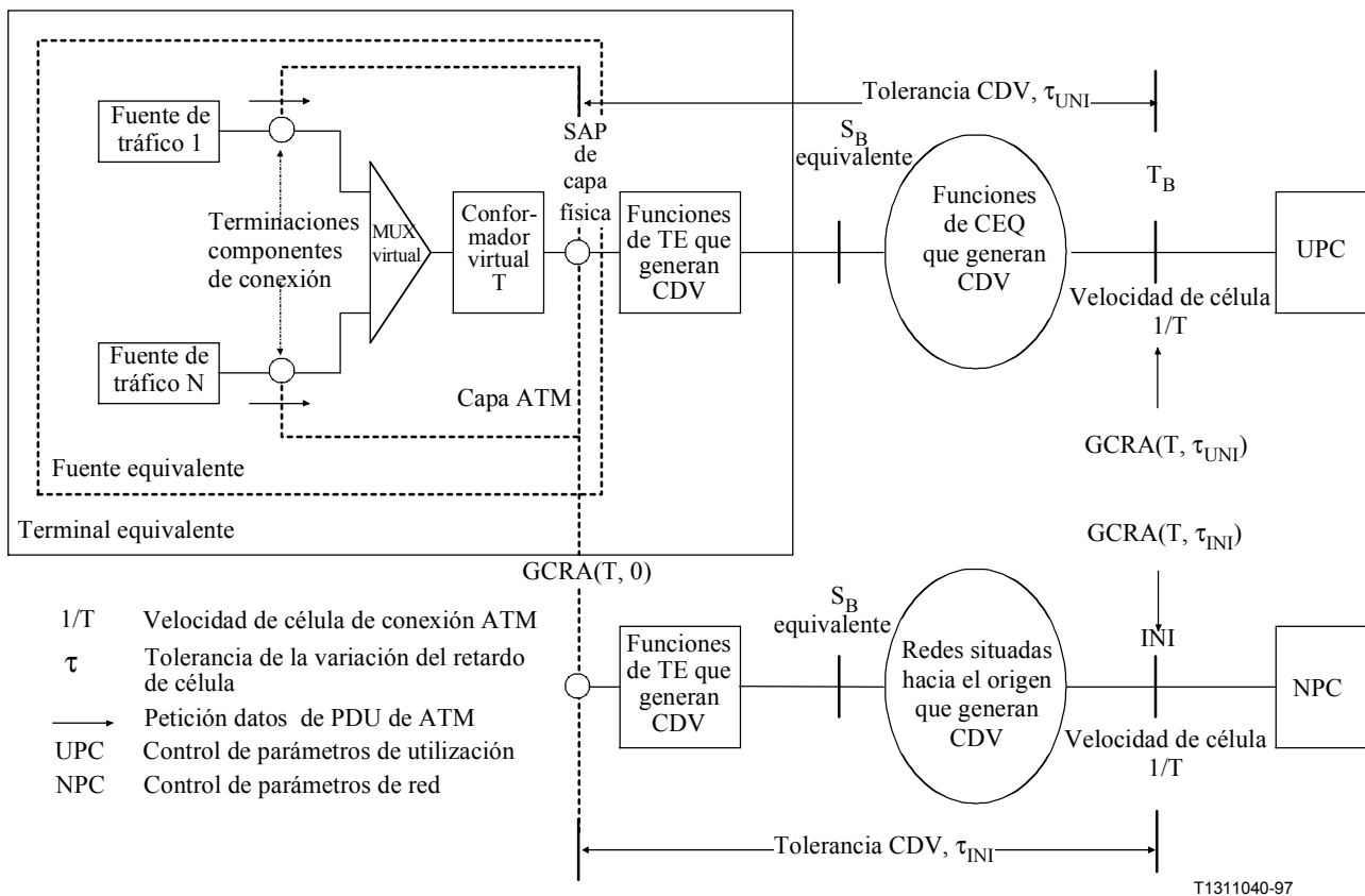
Figura 5/I.371 – Fuente equivalente y terminal equivalente para la definición de una velocidad de célula de una conexión
