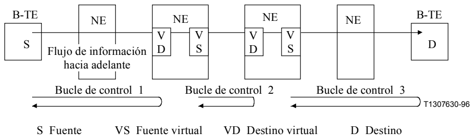
Figura 15/I.371 – Ejemplo de una conexión virtual segmentada
