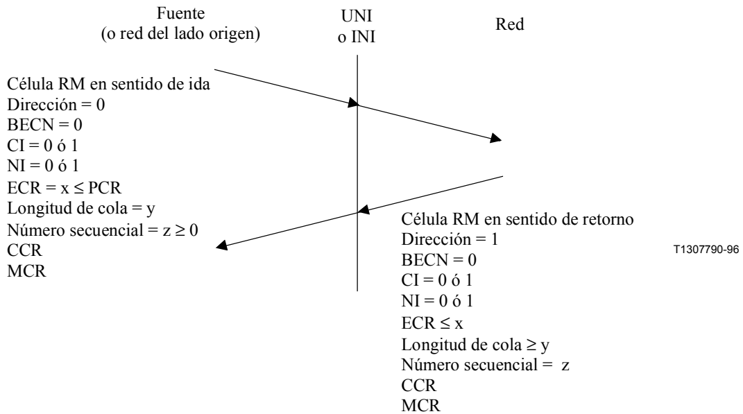
Figura F.1/I.371 – Una sola célula RM pendiente en la conexión bidireccional
