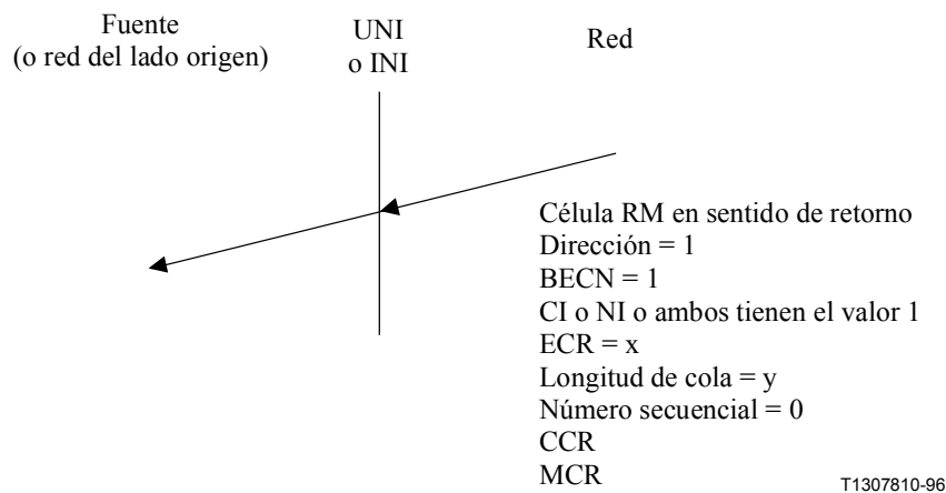
Figura F.3/I.371 – Una célula RM en la conexión de retorno originada por un elemento de red o por el destino
