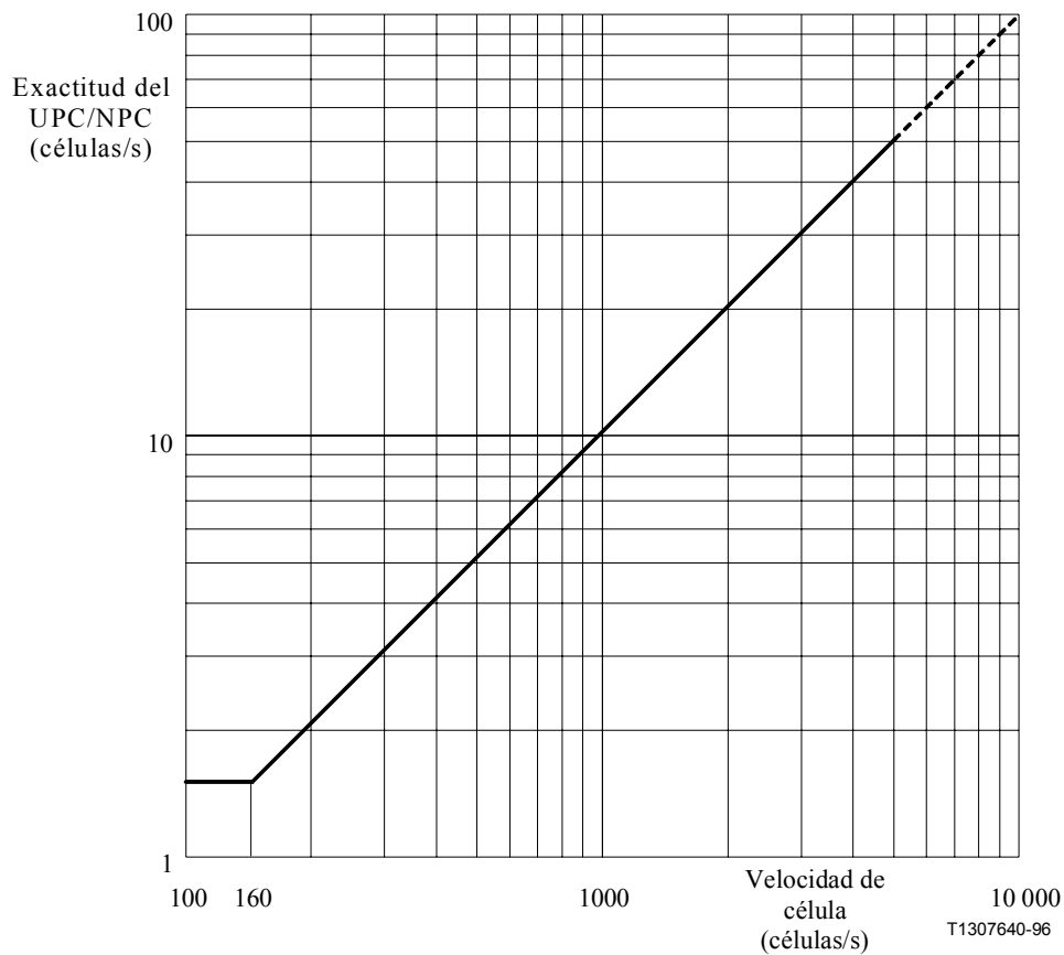
Figura 17/I.371 – Requisito de exactitud del UPC/NPC
