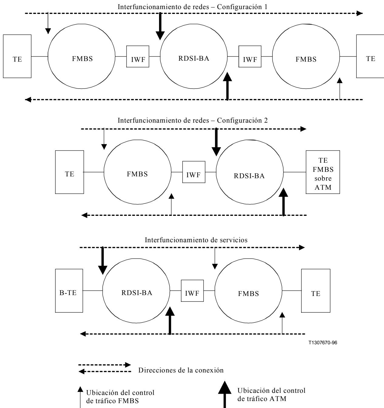
Figura 20/L.371 – Configuraciones de referencia para el interfuncionamiento de control de tráfico entre el FMBS y la RDSI-BA
