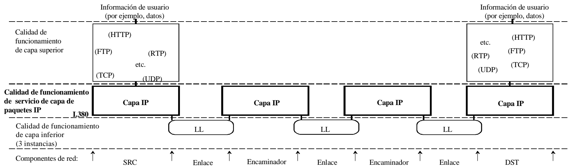
Figura 2/I.380 – Modelo estratificado por capas de calidad de funcionamiento de servicio IP – Ejemplo
