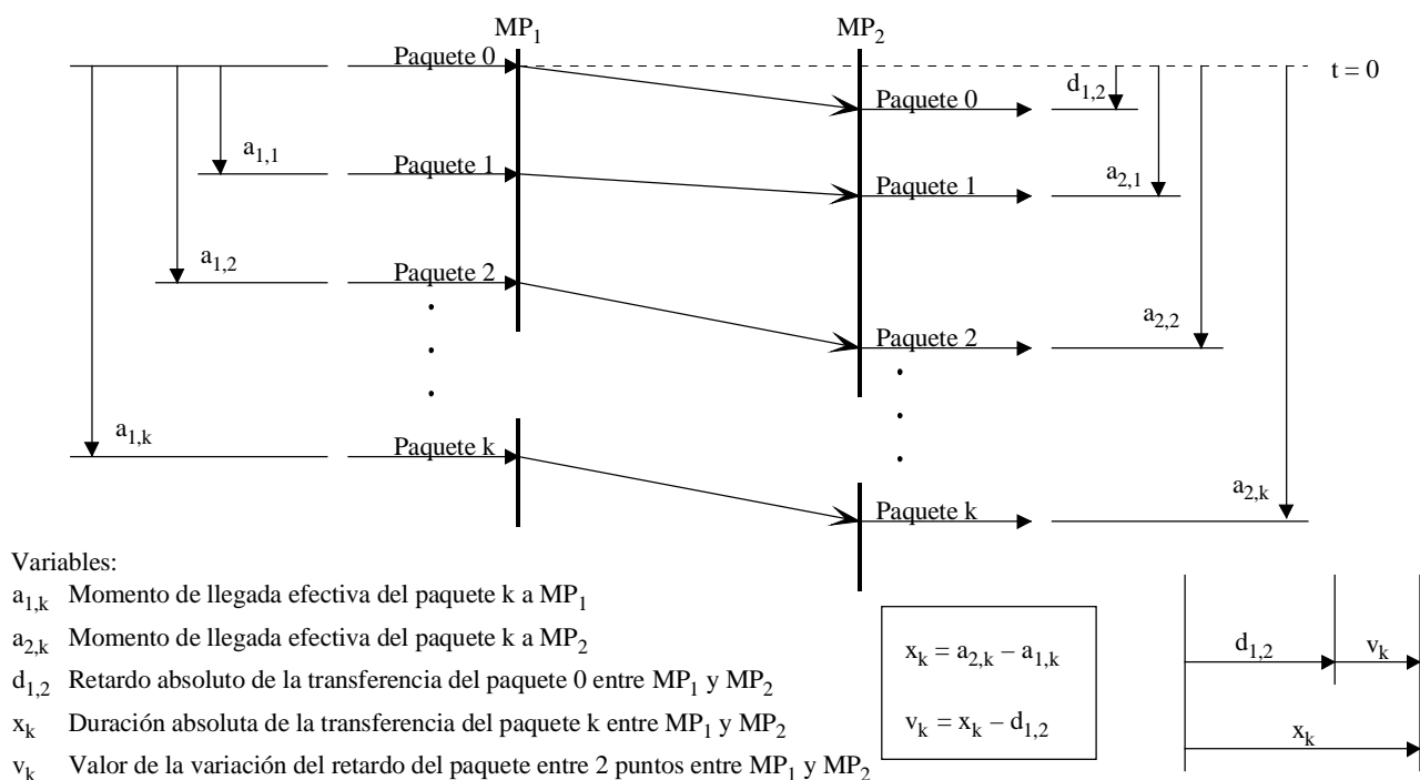
Figura II.1/I.380 – Variación del retardo de paquetes IP entre dos puntos
