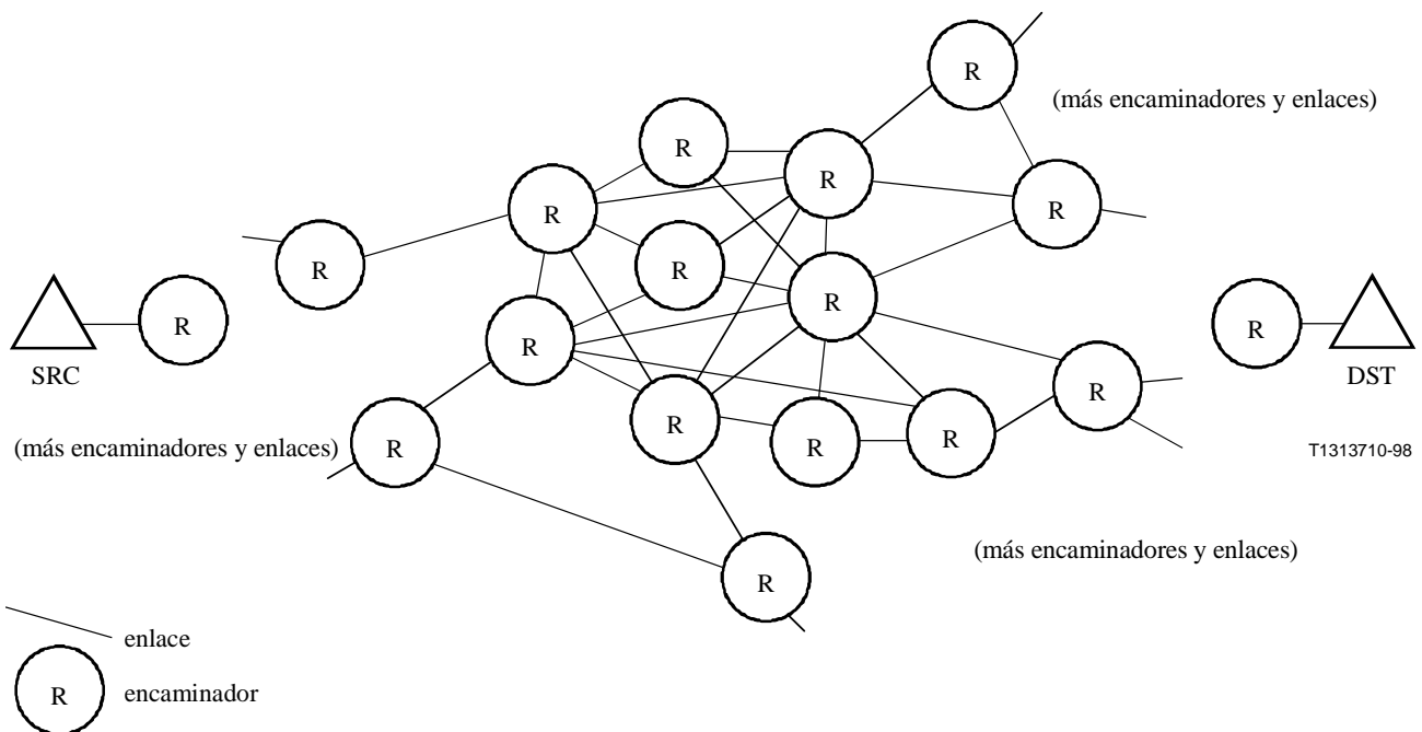
Figura 3/I.380 – Componentes de red IP
