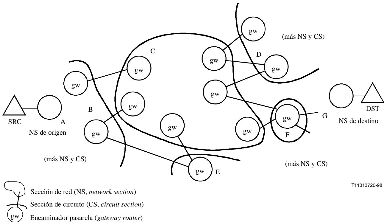
Figura 4/I.380 – Conectividad de red IP
