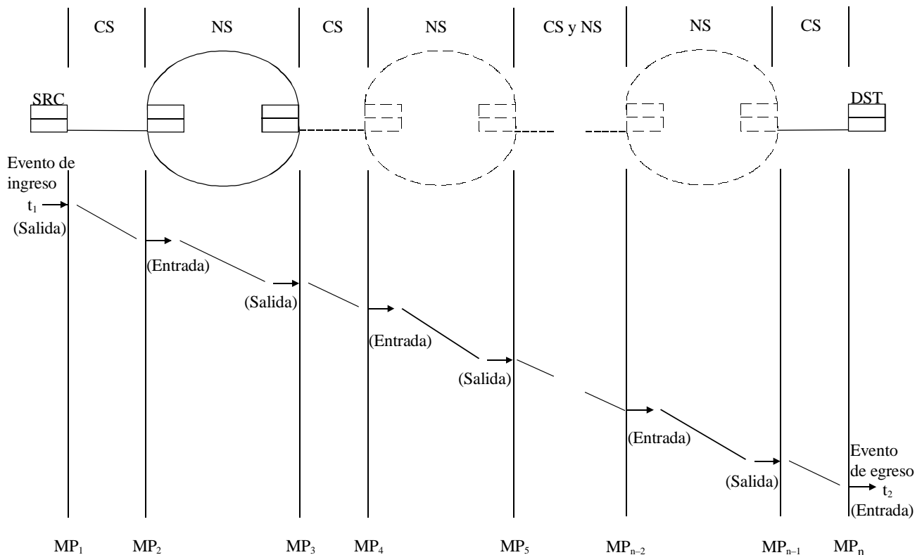
Figura 8/I.380 – Eventos de retardo de transferencia de paquetes IP (ilustración de la transferencia de extremo a extremo de un solo paquete IP)
