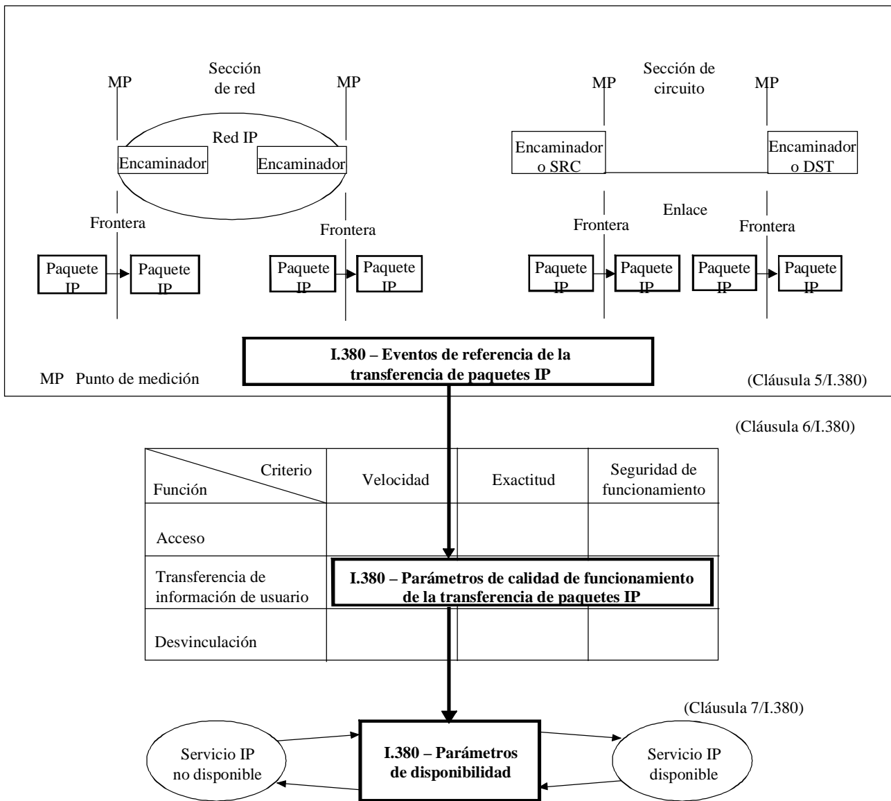
Figura 1/I.380 – Alcance de la Recomendación UIT-T I.380
