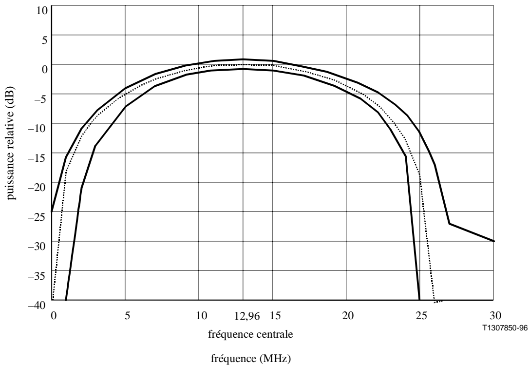
Figure 4/I.432.4 – Gabarit du spectre de puissance du signal à la sortie de l'émetteur
