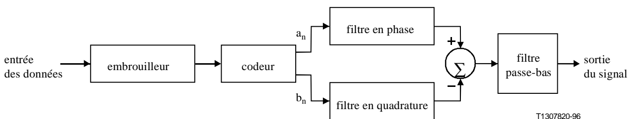
Figure 1/I.432.4 – Diagramme fonctionnel d'un émetteur numérique 16-QAM
