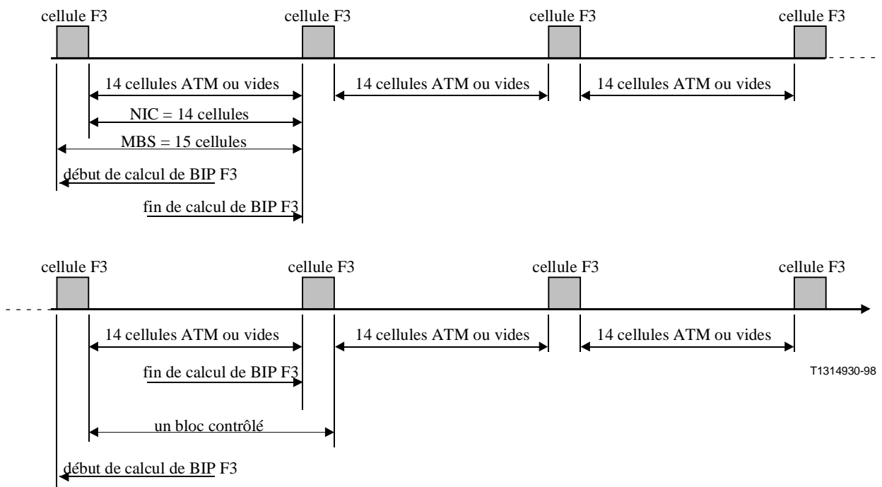
Figure 8/I.432.4 – Implémentation du flux OAM F3 au point S LB
