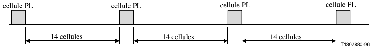
Figure 7/I.432.4 – Adaptation à la capacité de transfert
