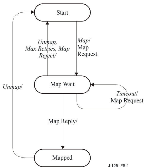
Figure 8-1/J.125 – SA Mapping state machine flow diagram
