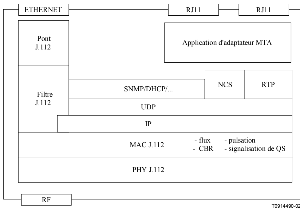
Figure 1/J.173 – Adaptateur MTA intégré
