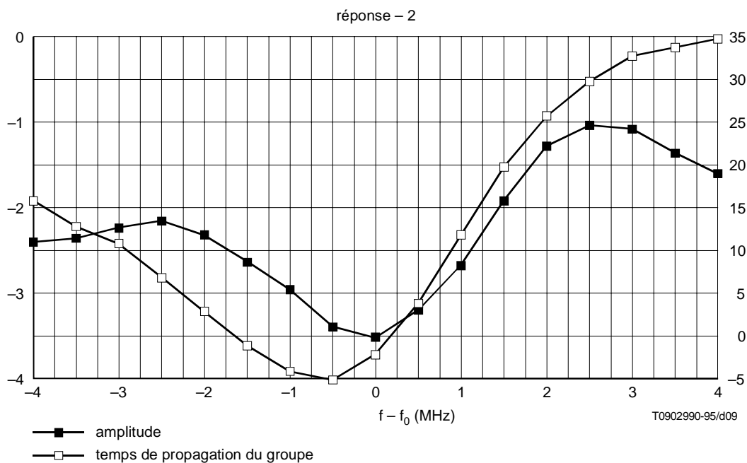
Figure A.II.2/J.84 – Exemple représentatif de la fonction de transfert mesurée sur le réseau SMATV considéré
