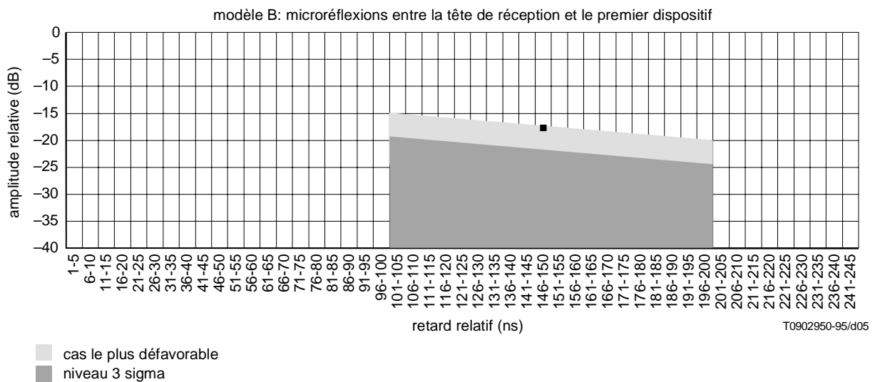
Figure A.I.2/J.84 – Modèle B de réponse du canal RF d'un réseau de distribution SMATV dans les bandes UHF et S
