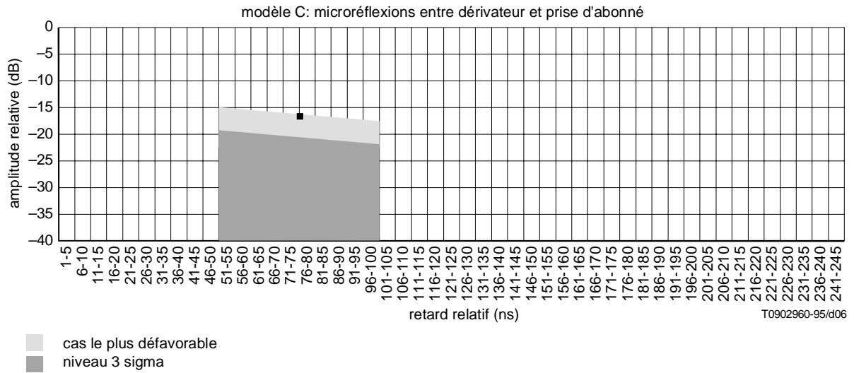
Figure A.I.3/J.84 – Modèle C de réponse du canal RF d'un réseau de distribution SMATV dans les bandes UHF et S
