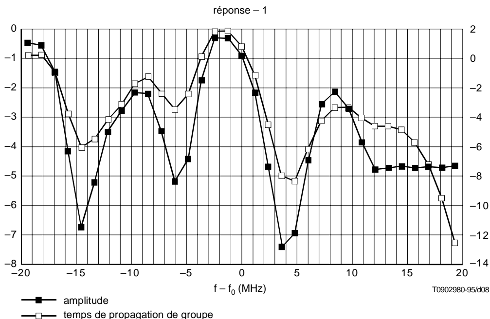
Figure A.II.1/J.84 – Exemple représentatif de la fonction de transfert mesurée sur le réseau SMATV considéré
