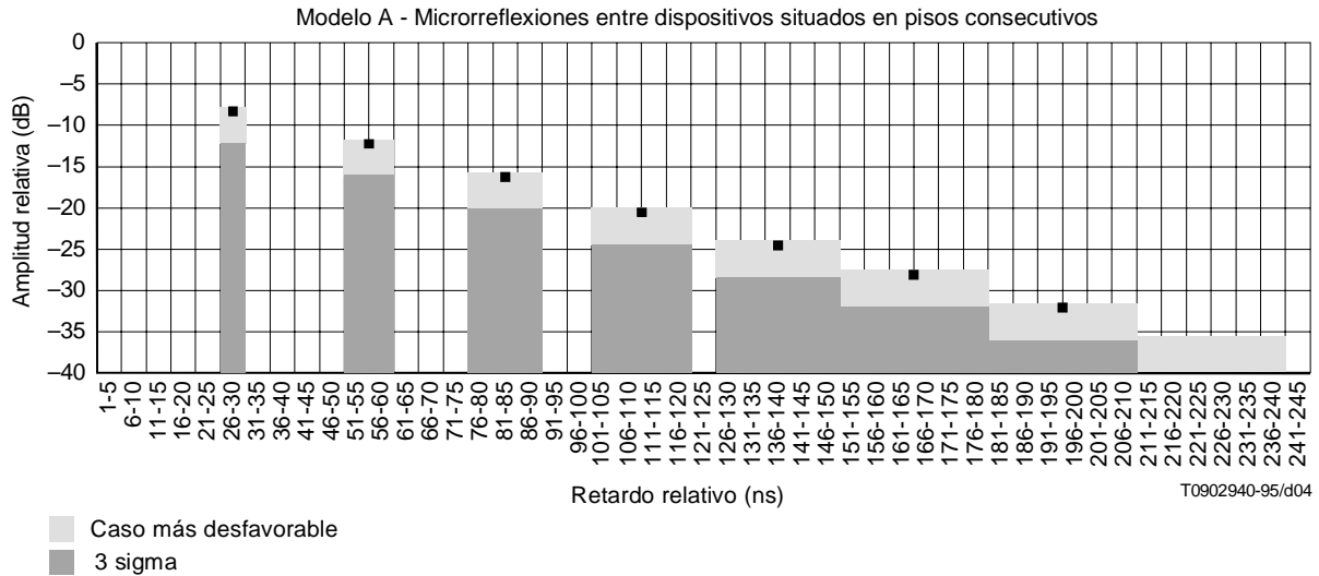
Figura A.I.1/J.84 – Respuesta del modelo A de canal RF de una red de distribución SMATV de UHF y de banda S
