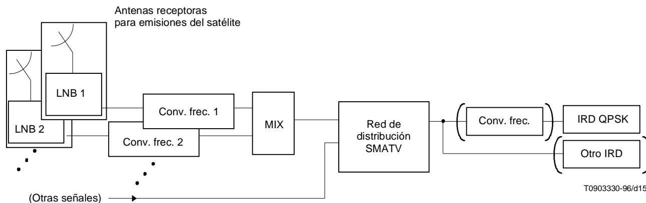
Figura C.2/J.84 – Sistema SMATV C(II)
