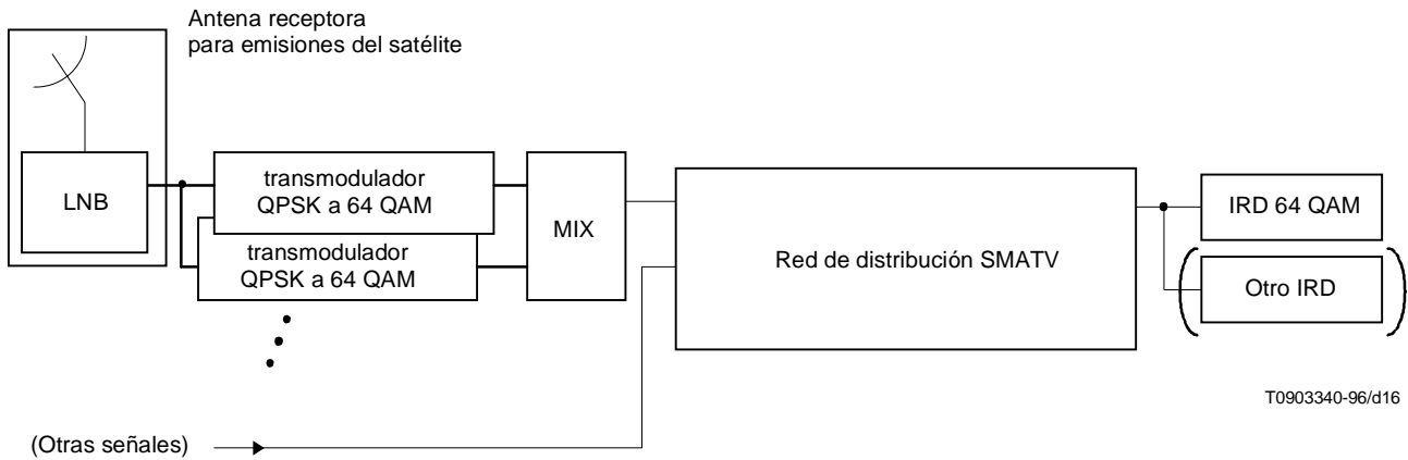
Figura C.3/J.84 – Sistema SMATV C(III)
