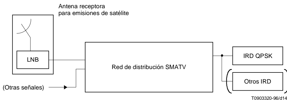
Figura C.1/J.84 – Sistema SMATV C(I)
