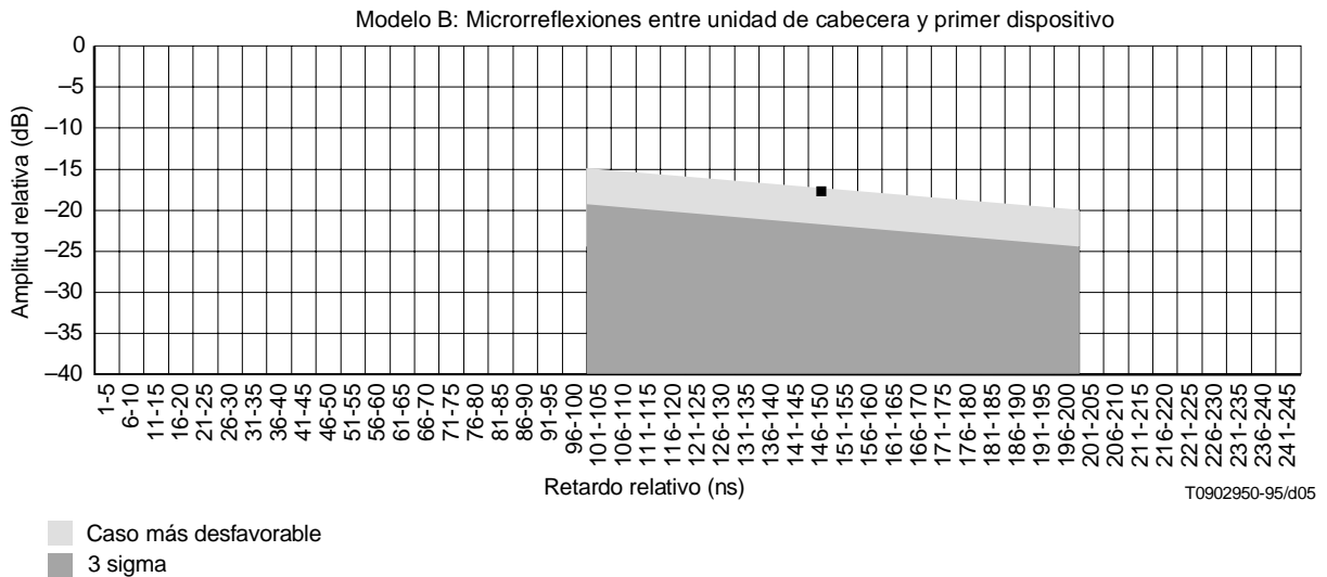
Figura A.I.2/J.84 – Respuesta del modelo B de canal RF de una red de distribución SMATV de UHF y de banda S
