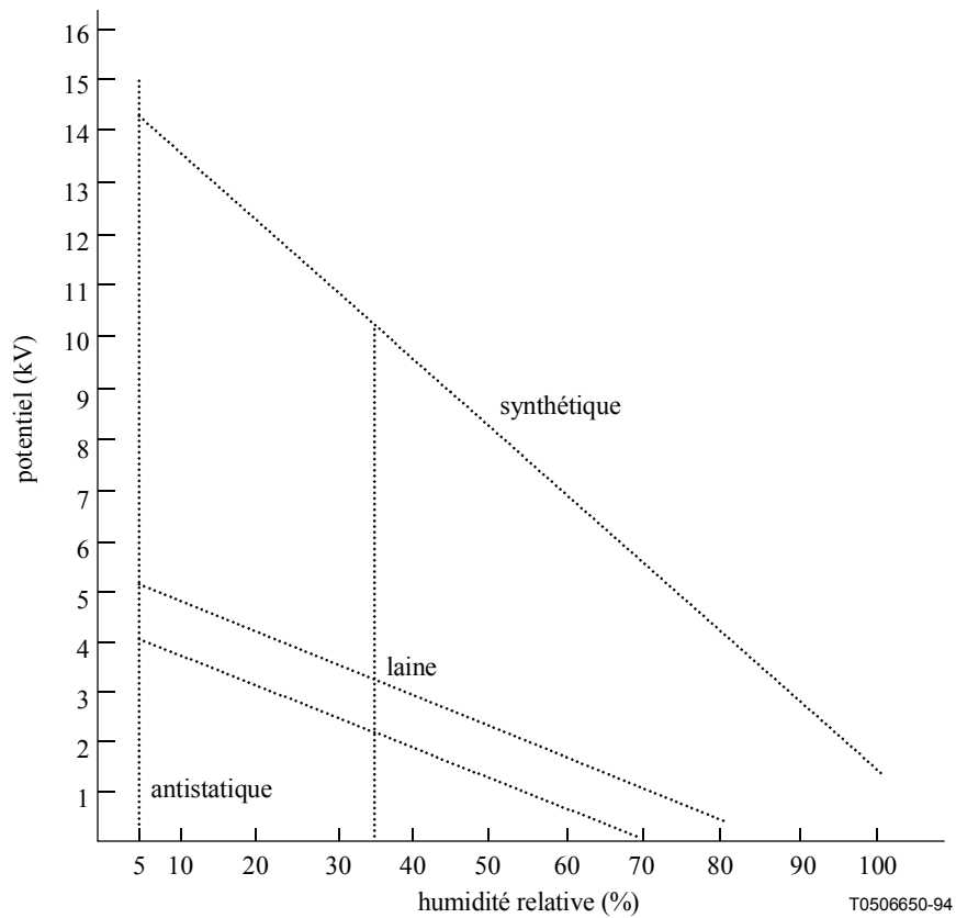
Figure 1/K.34 – Valeurs maximales des potentiels électrostatiques dont peuvent être porteurs des exploitants en contact avec les matériaux indiqués, en l'absence de mesures de protection électrostatique
