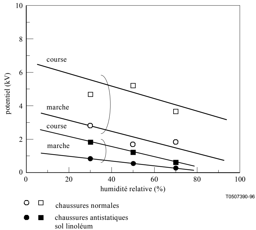
Figure 2/K.34 – Valeur maximale de la tension électrostatique dont les exploitants peuvent être chargés dans un centre de télécommunication
