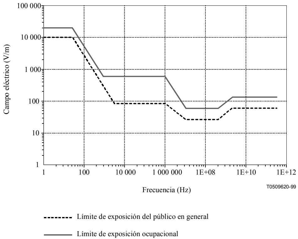
Figura I.1/K.52 – Límites de referencia ICNIRP de intensidad del campo eléctrico
