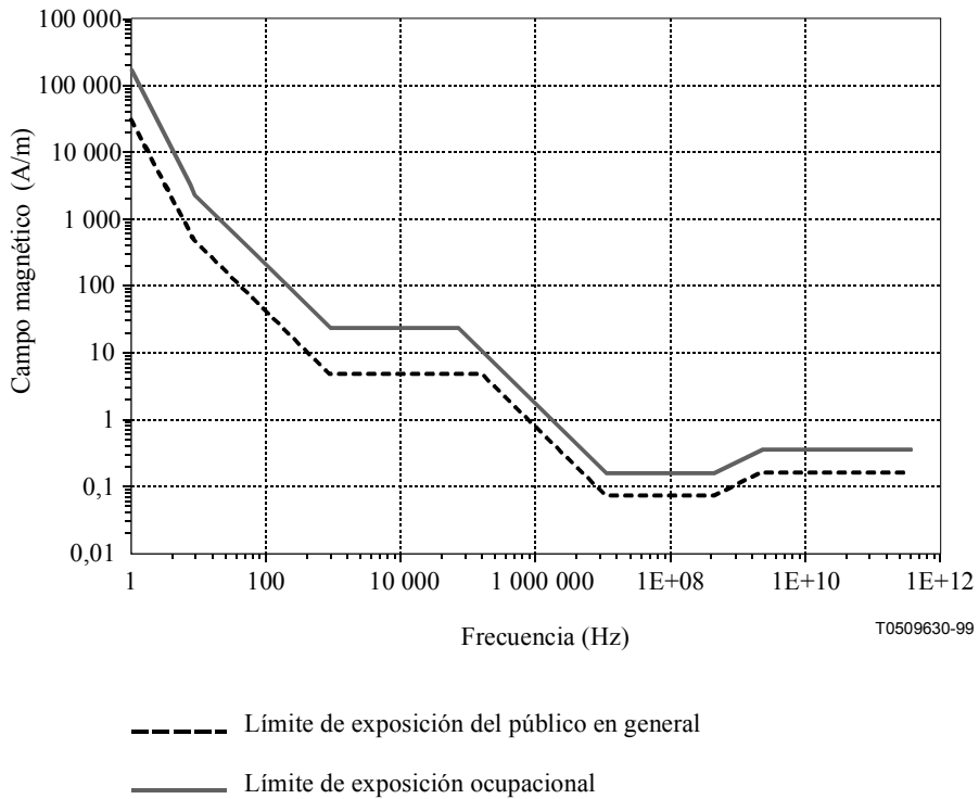
Figura I.2/K.52 – Límites de referencia ICNIRP de intensidad del campo magnético
