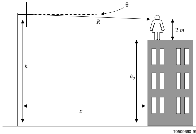
Figura II.3/K.52 – Ejemplo de configuración para calcular la exposición en un edificio adyacente
