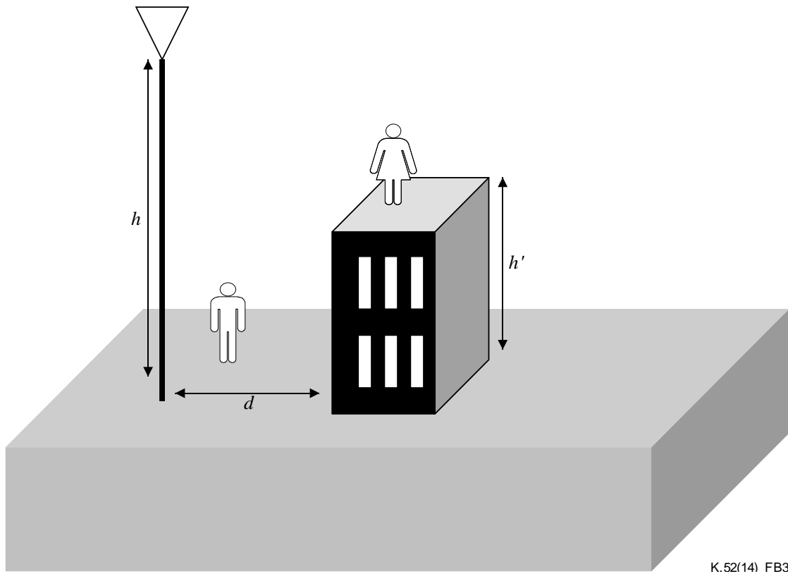
图B.3—可达性类型3示意图
