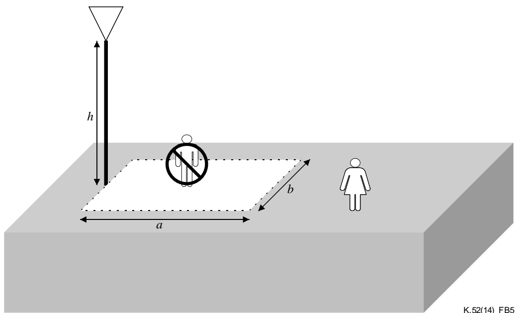
图B.5—可达性类型4示意图，矩形禁止区域
