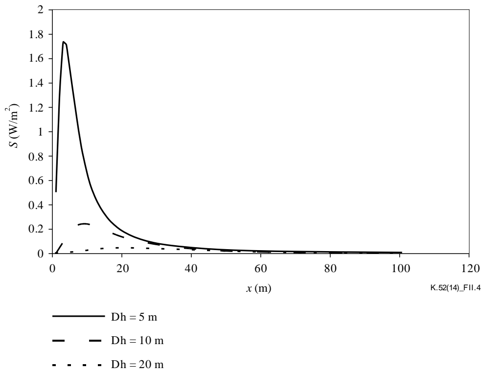
图II.4—附近建筑物上的功率密度对图II.3中示例建筑物与天线塔的距离关系图
