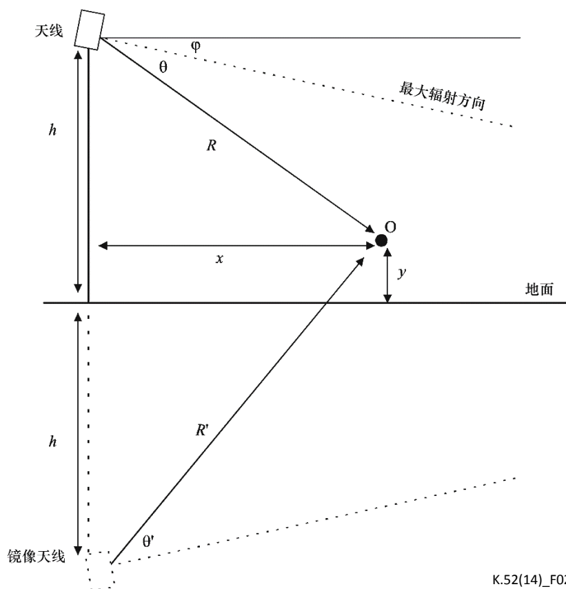
图2—距离和垂直角的定义
