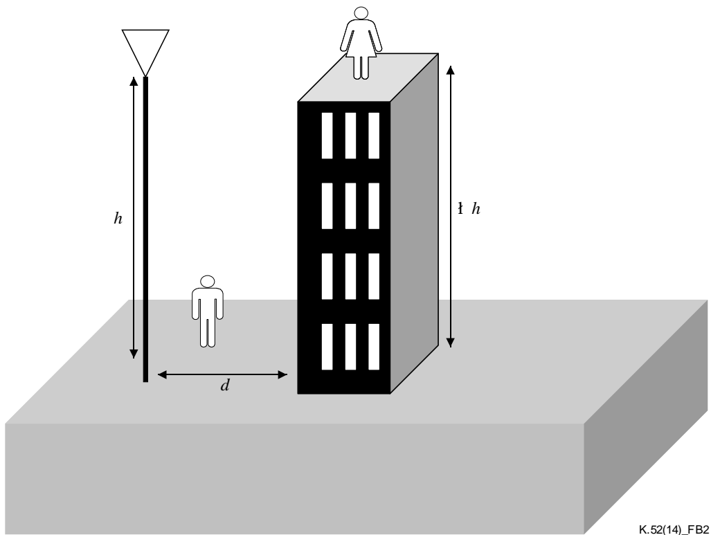
图B.2—可达性类型2示意图
