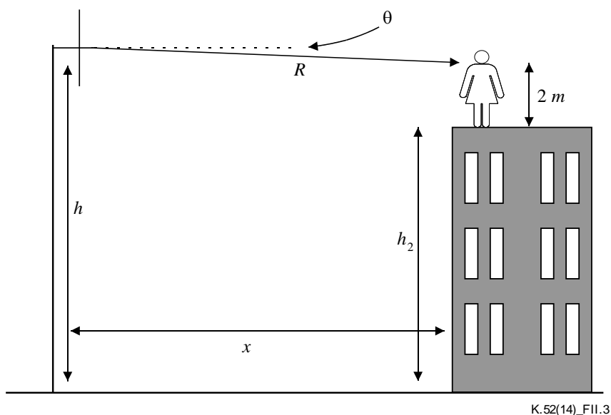
图II.3—计算附近建筑物上的暴露的示意图
