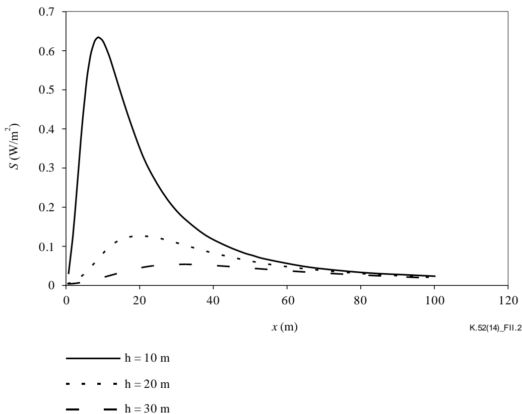
图II.2—地面上的功率密度对图II.1中示例人与天线塔的距离关系图
