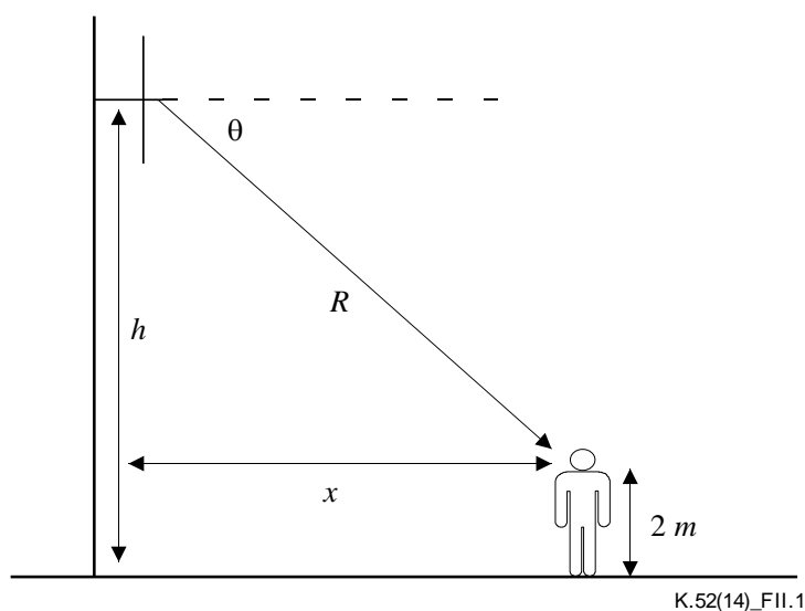
图II.1—计算地面上的暴露的布置示意图
