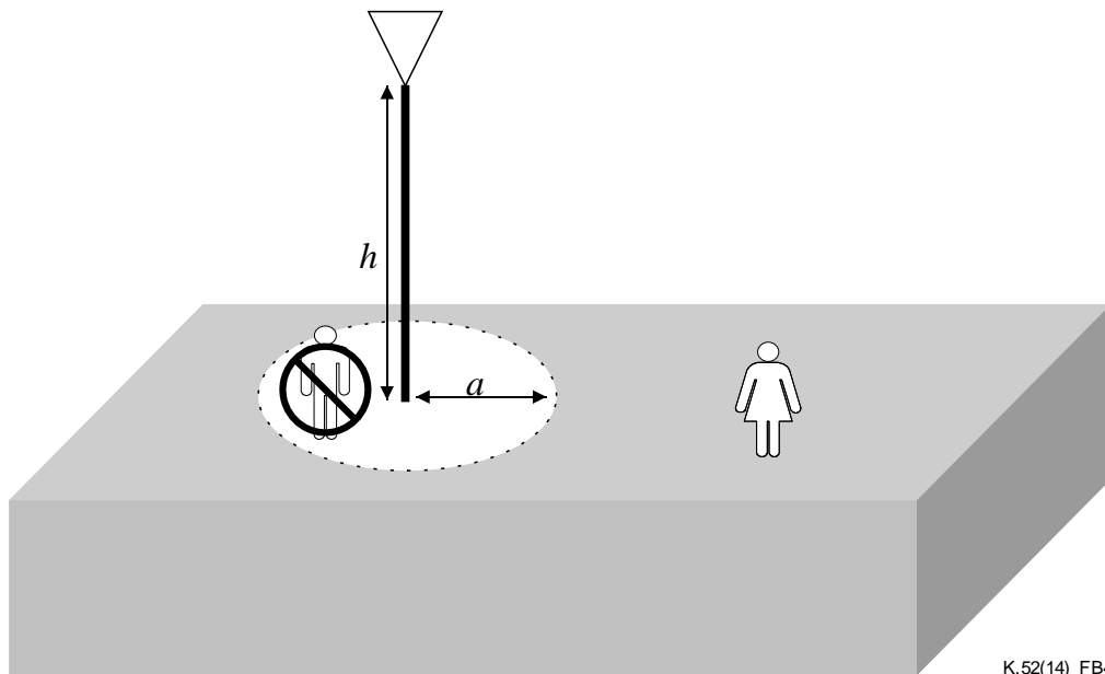
图B.4—可达性类型4示意图，圆形禁止区域
