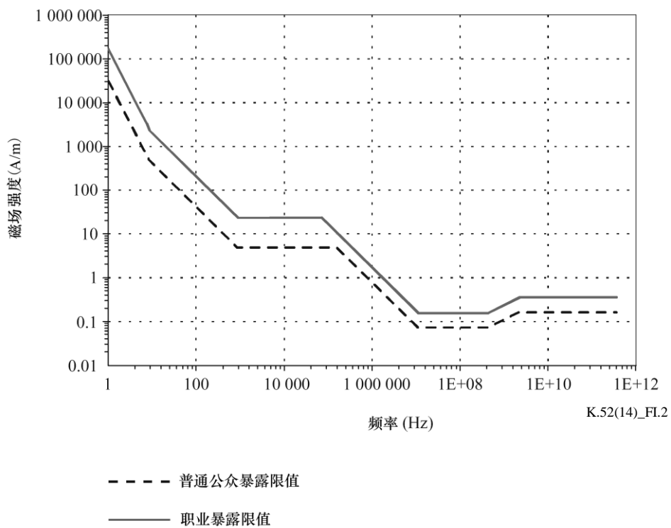
图I.2—ICNIRP磁场强度的导出限值
