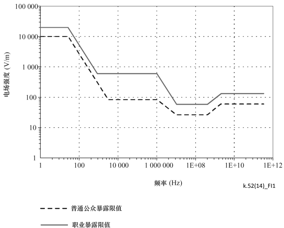
图I.1—ICNIRP电场强度的导出限值
