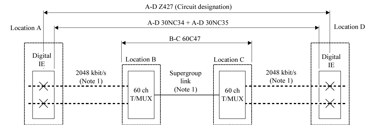
a) Digital-analogue-digital route
