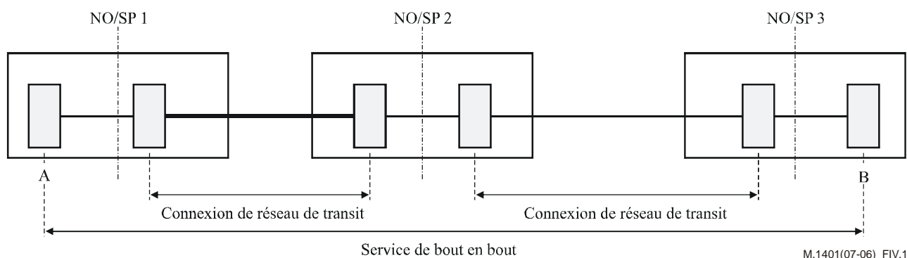
Figure IV.1/M.1401 – Réseau de transit
