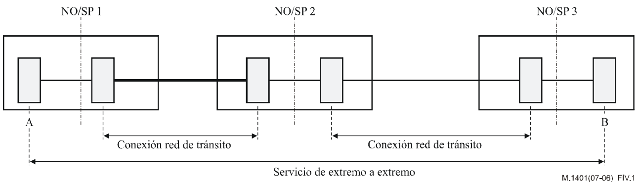
Figura IV.1/M.1401 – Red de tránsito
