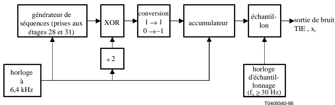
Figure V.1/O.172 – Source de bruit TIE utilisée pour la vérification des algorithmes de calcul d'écart MTIE et TDEV
