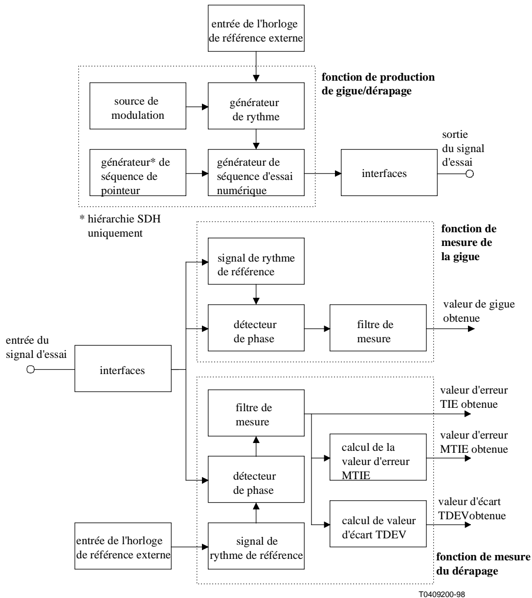
Figure 1/O.172 – Organigramme fonctionnel de l'appareil de test de gigue et de d r page
