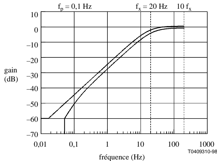
Figure IV.1/O.172 – Limites de masque pour filtre passe-haut de mesure de gigue à 2048 kbit/s à 20 Hz
