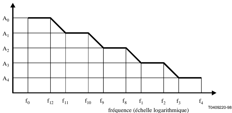
Figure 3/O.172 – Amplitude de la gigue et du dérapage produits en fonction de la fréquence de la gigue et du dérapage
