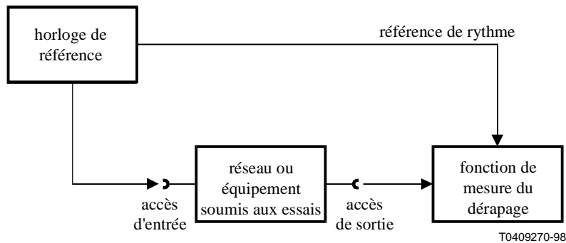
Figure II.1/O.172 – Configuration pour les mesures de dérapage synchronisées
