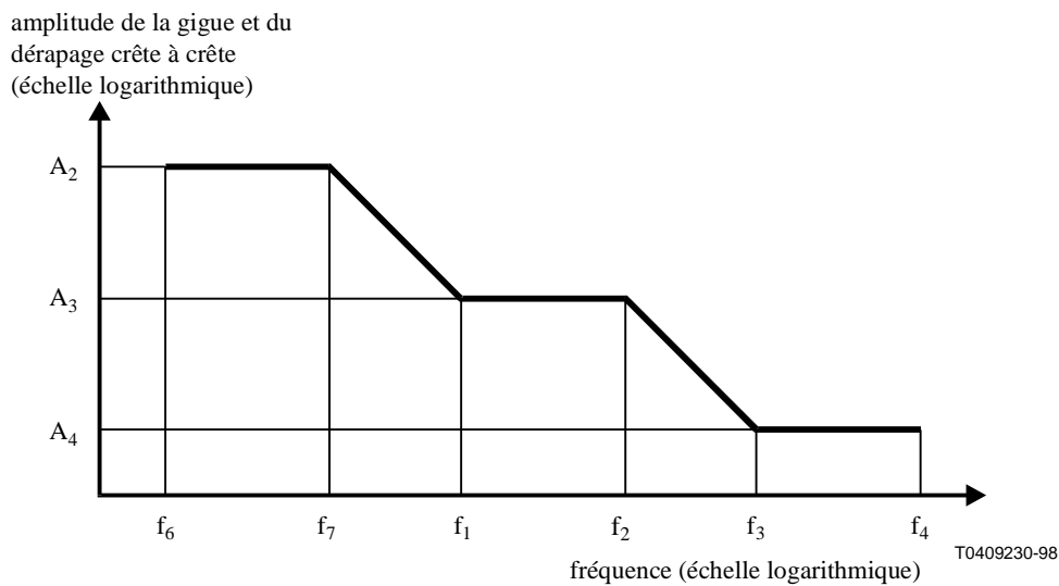
Figure 4/O.172 – Amplitude de la gigue mesurée en fonction de sa fréquence
