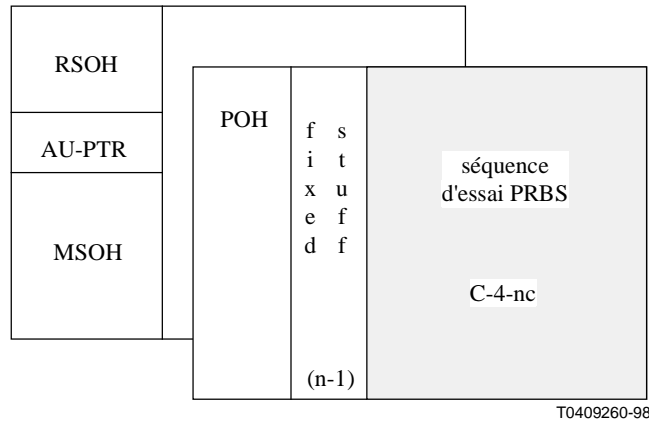
Figure A.3/O.172 – Structure de signal d'essai pour la mesure de la gigue de l'interface STM-N concaténé
