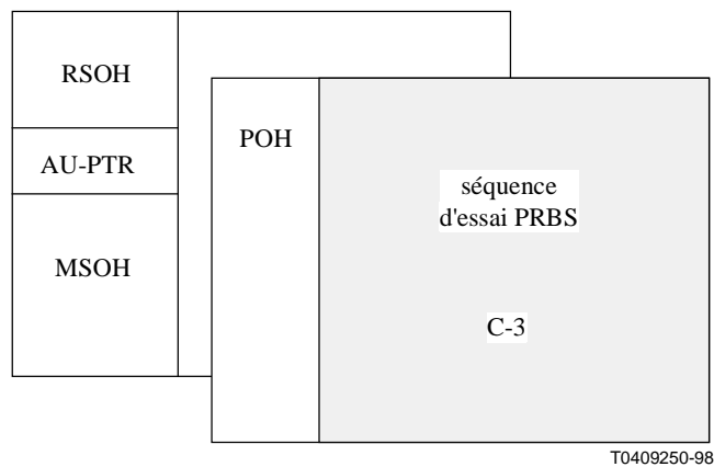
Figure A.2/O.172 – Structure de signal d'essai pour la mesure de la gigue de l'interface STM-0
