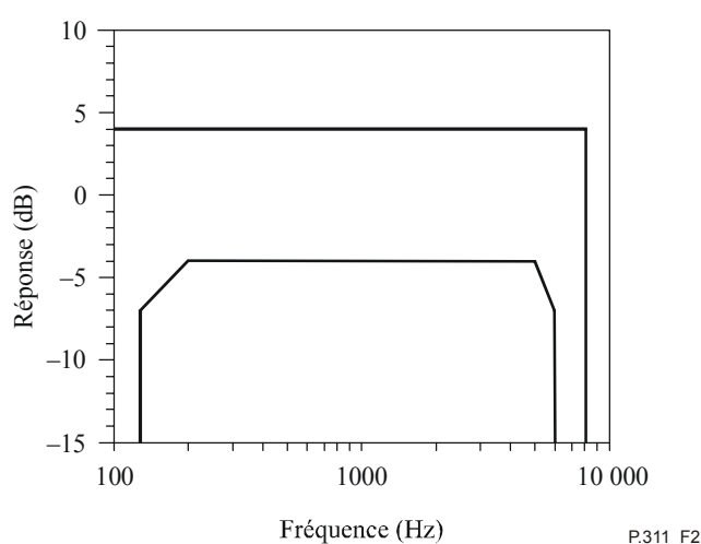
Figure 2/P.311 – Caractéristique du combiné à la réception
