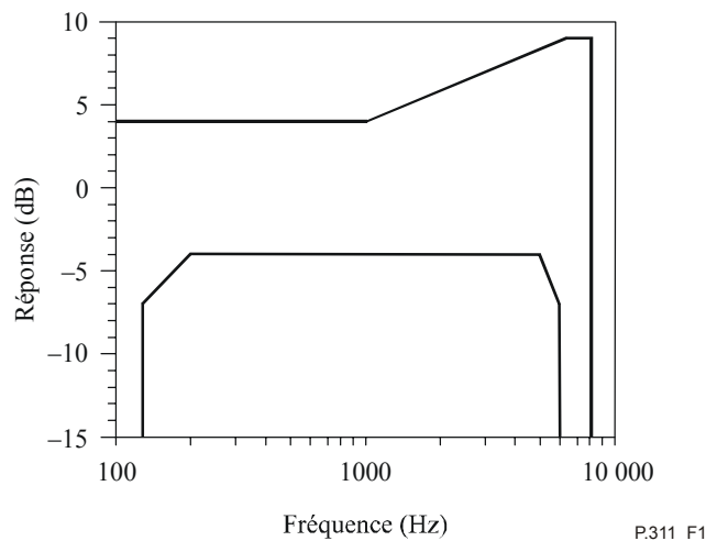
Figure 1/P.311 – Caractéristique du combiné à l'émission
