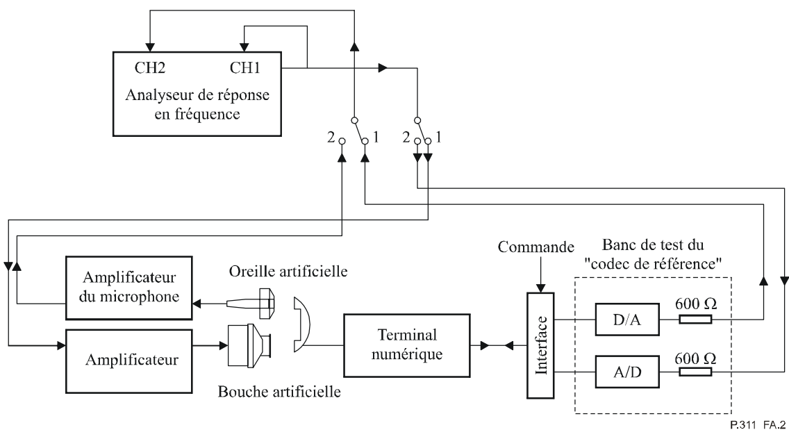
Figure A.2/P.311 – Configuration pour la mesure du temps de propagation de groupe audiofréquence
