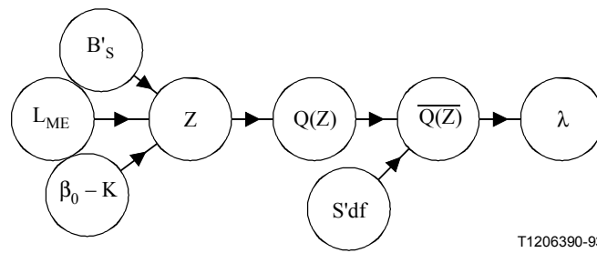
Figura A.3/P.79 – Esquema de principio que muestra la forma en que la sonoridad, \lambda , está relacionada con el nivel de sensación, Z
