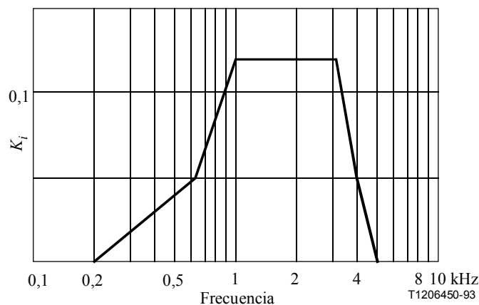
Figura E.1/P.79 – Coeficientes K_i para el factor D
