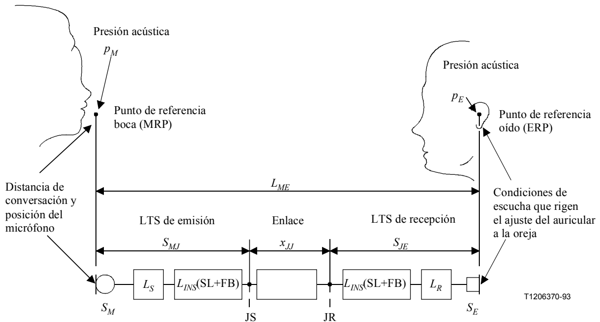
Figura A.1/P.79 – Factores que influyen en la sonoridad de la palabra recibida
