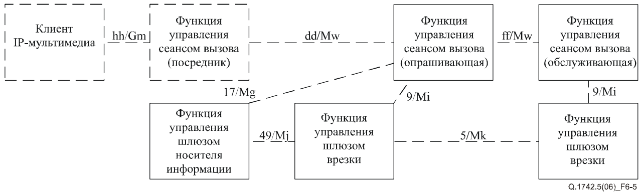
Рисунок 6-5/Q.1742.5 – Эталонная модель управления сеансом
